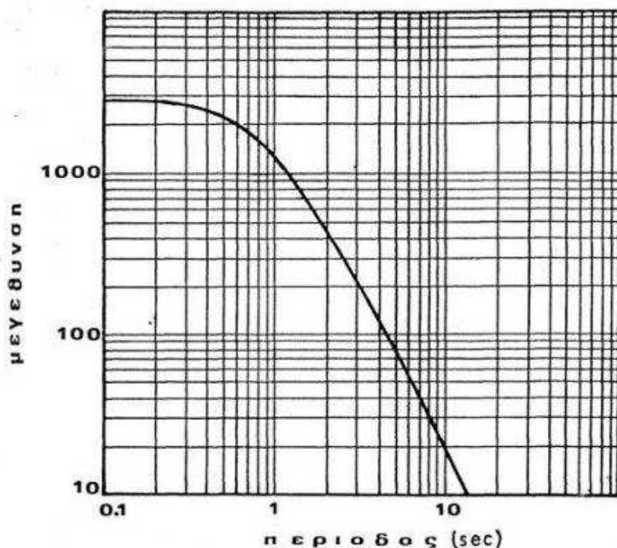
σχήμα 2.2: καμπύλη μεγέθυνσης συναρτήσει της περιόδου
