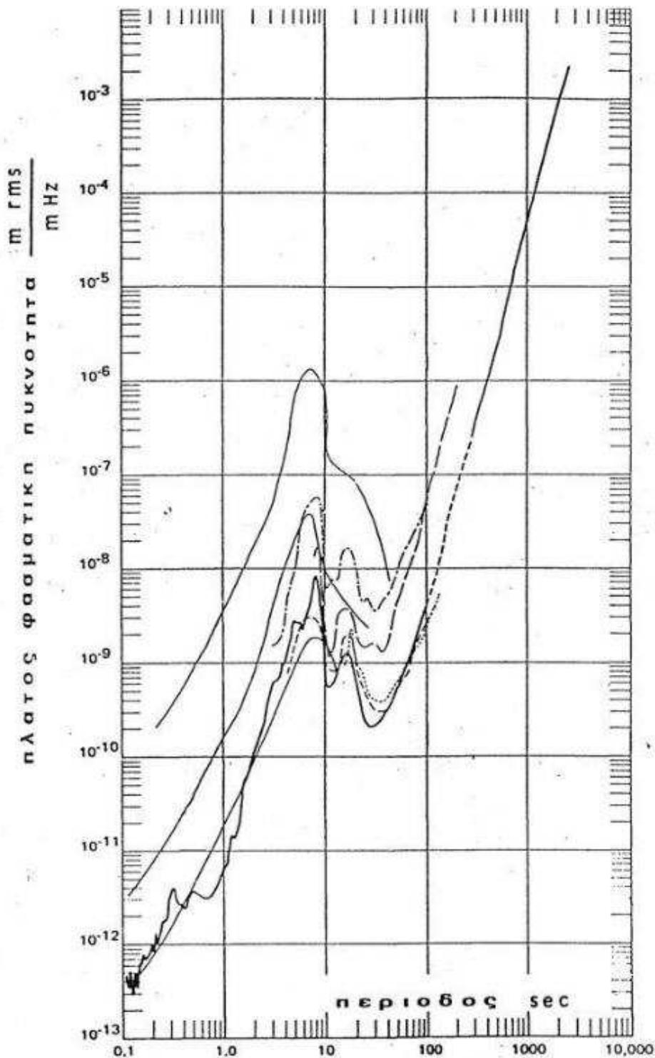
σχήμα 2.6: χαρακτηριστικά φάσματα του πλάτους του θορύβου που καλύπτουν το εύρος περιόδων από 0.1 sec έως 10000 sec (Brune και Oliver 1959) και προέρχονται από εγγραφές κατακόρυφου σεισμομέτρου.
