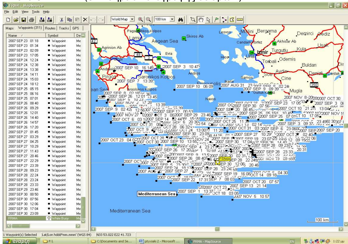
Εικόνα 6 : FRMA: (311 σημεία καταγραφής σεισμών )
