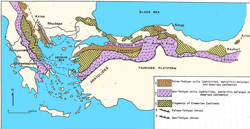
σχήμα 1.1: Ελληνικές γεωτεκτονικές ζώνες
