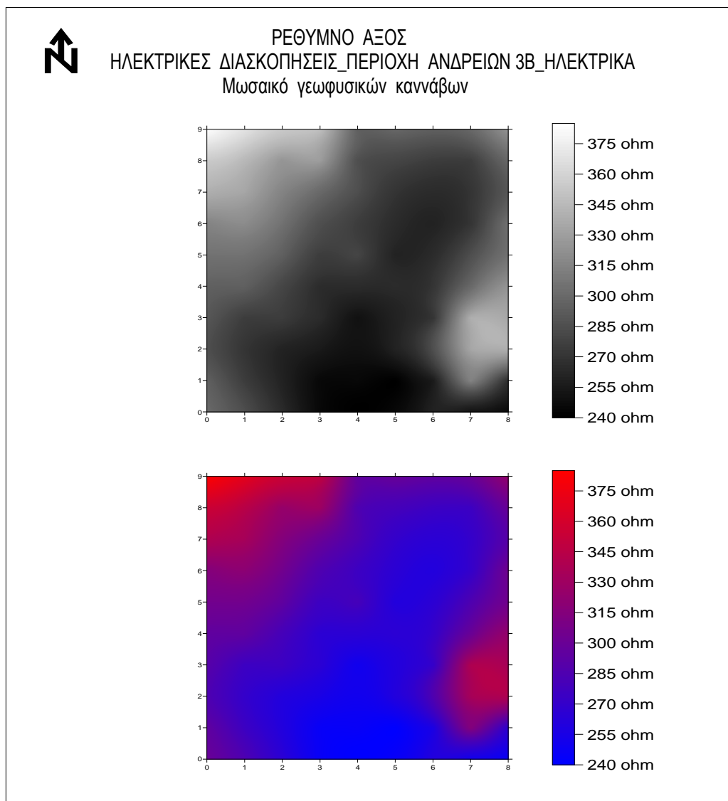
Σχήμα 4.3.3 περιοχή Ανδρείων 3B ηλεκτρικά χωρίς συμπίεση.
