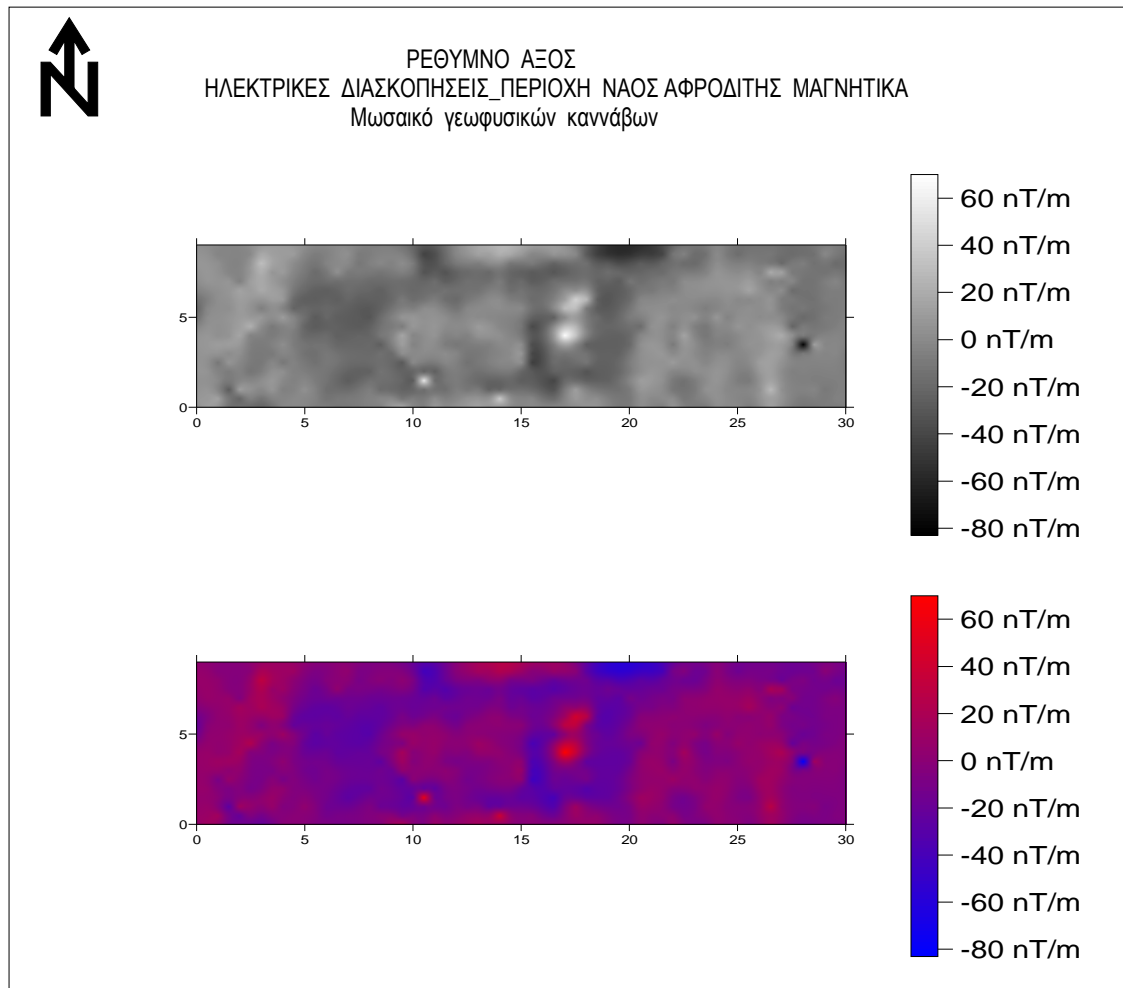
Σχήμα 4.1 περιοχή ναός Αφροδίτης μαγνητικά χωρίς συμπίεση
