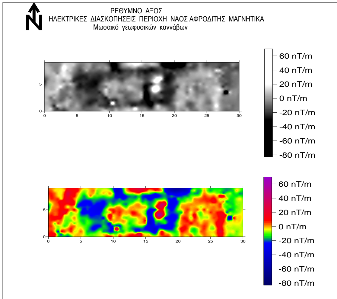
Σχήμα 4.1.1 περιοχή ναός Αφροδίτης μαγνητικά με συμπίεση
