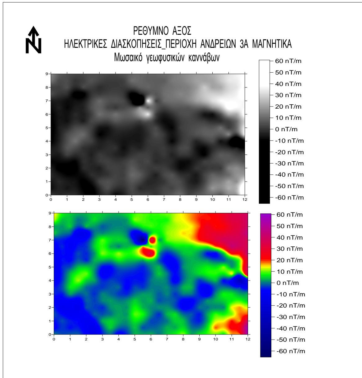
Σχήμα 4.4 περιοχή Ανδρείων 3Α μαγνητικά με συμπίεση.
