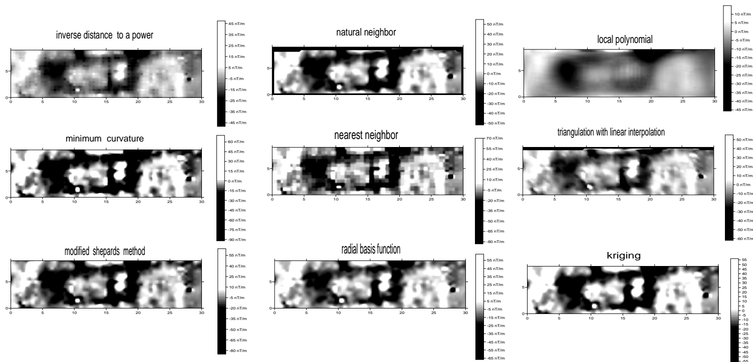
Σχήμα 4.2.4 εφαρμογή του grid data στο ναό Αφροδίτης με διαφορές από τις παραπάνω μεθόδους.
