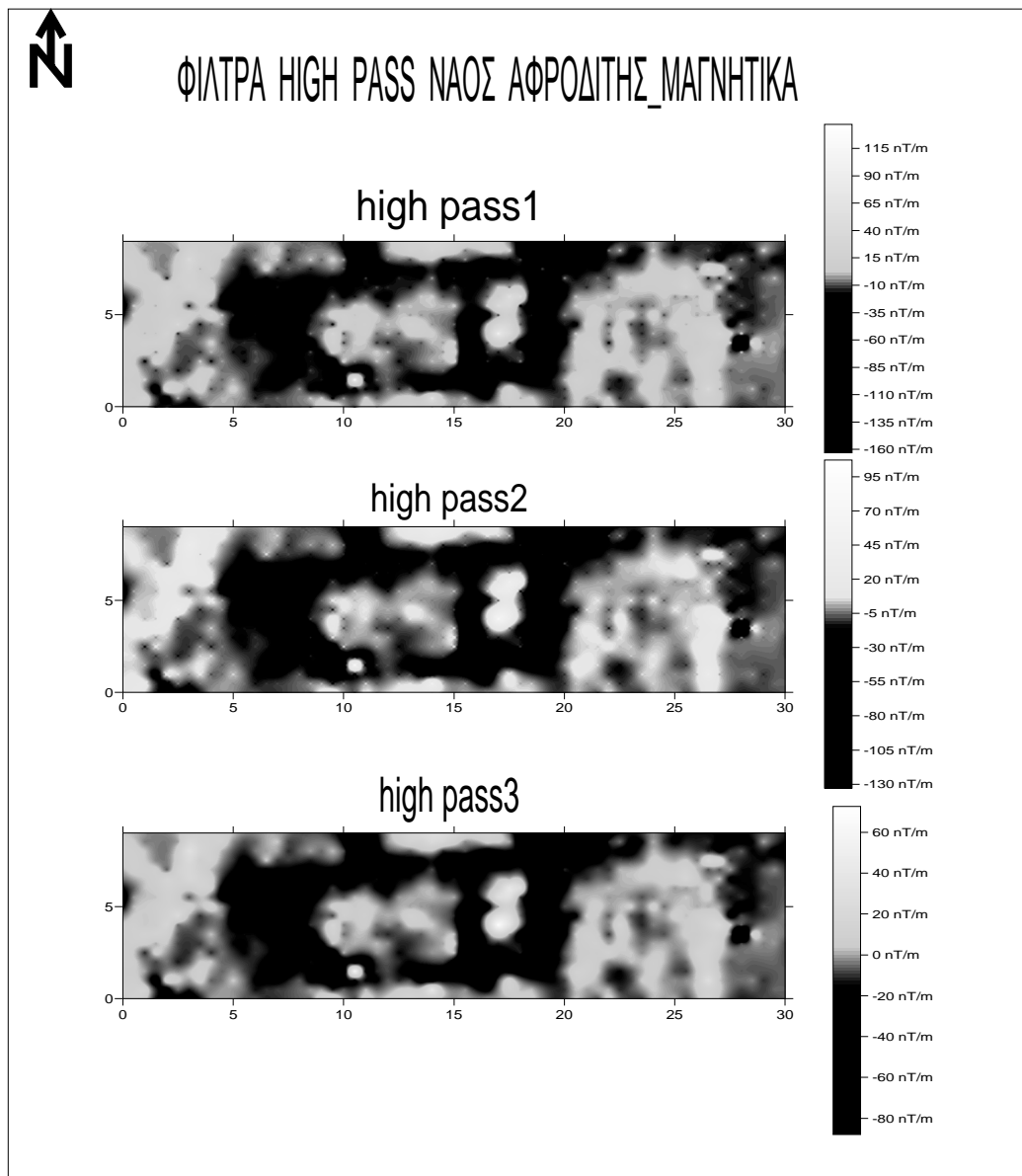
Σχήμα 4.1.5 φίλτρα high pass στο ναό Αφροδίτης-μαγνητικά.
