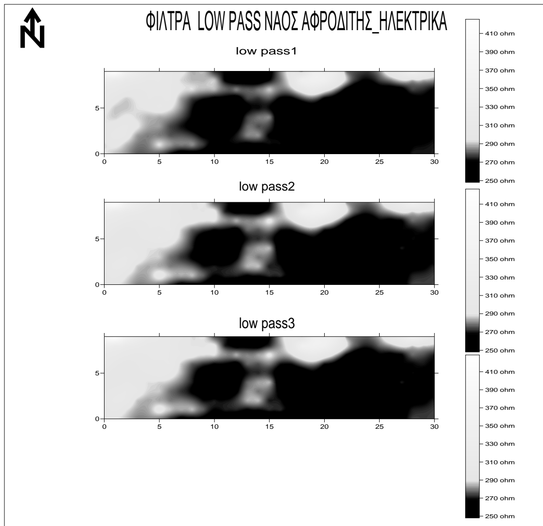
Σχήμα4.2.4 φίλτρα low pass ναός Αφροδίτης-ηλεκτρικά.
