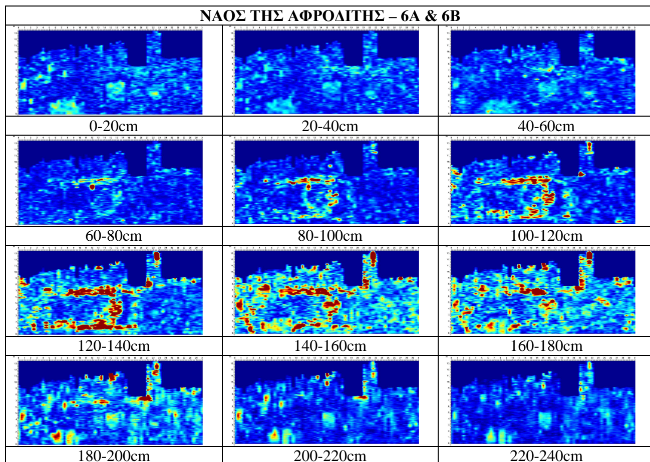
Σχήμα 4.1.4 Οριζόντιες τομές του υπεδάφους με αυξανόμενο βάθος (ανά 20cm) με τη χρήση του γεωραντάρ
