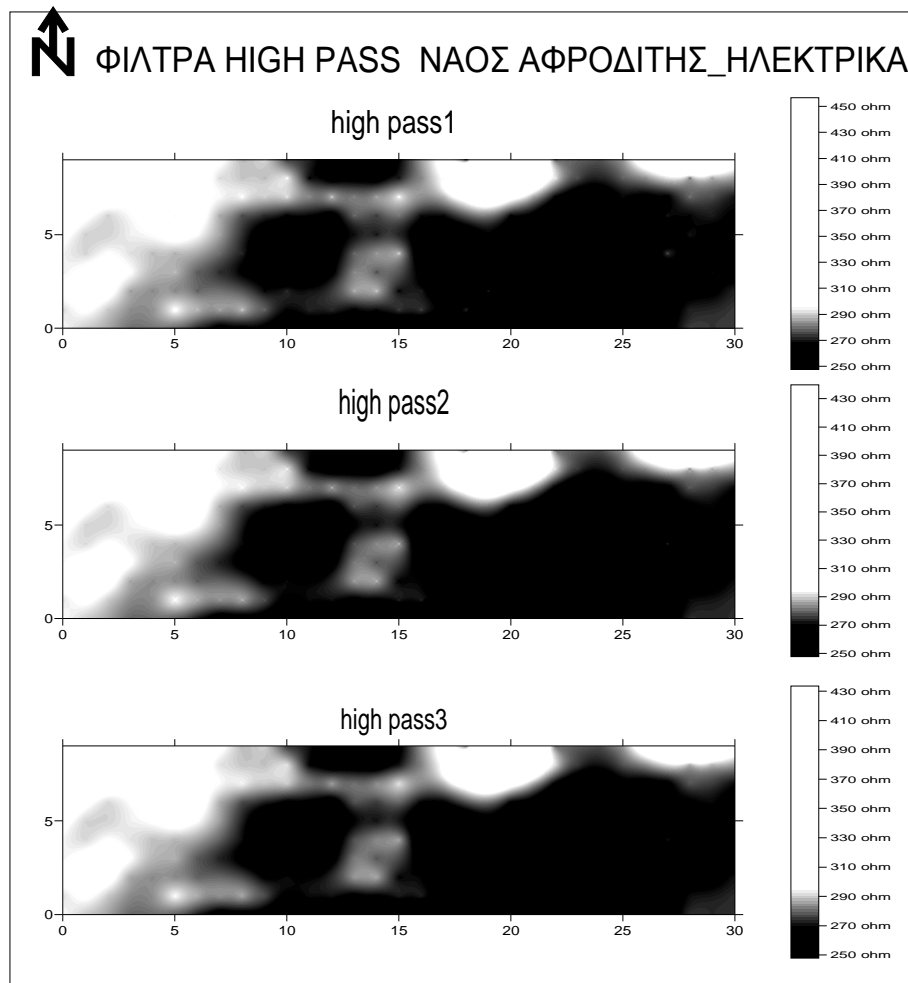
Σχήμα 4.2.2 φίλτρα high pass ναός Αφροδίτης-ηλεκτρικά.
