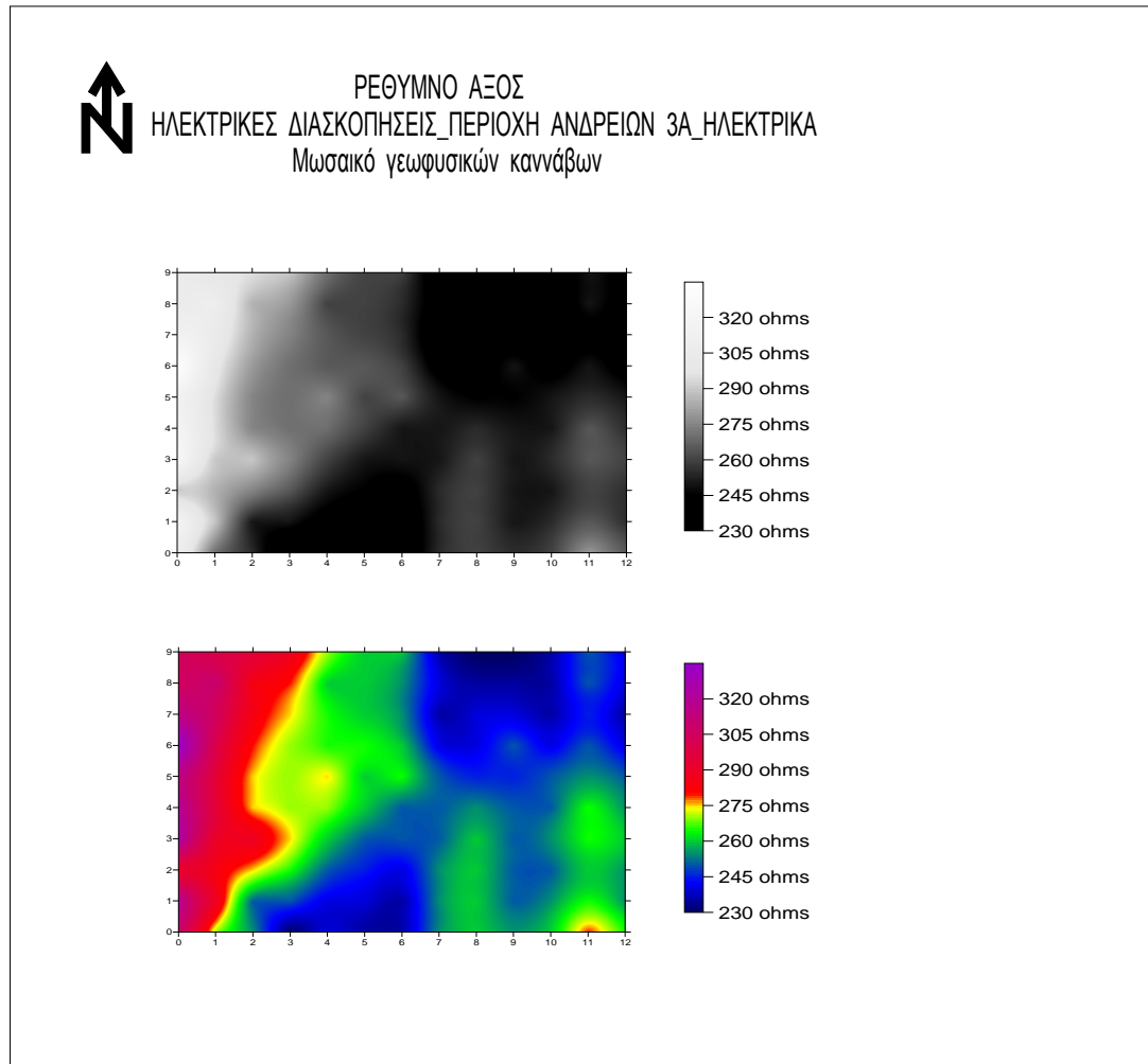
Σχήμα 4.3.2 περιοχή Ανδρείων 3Α ηλεκτρικά με συμπίεση.
