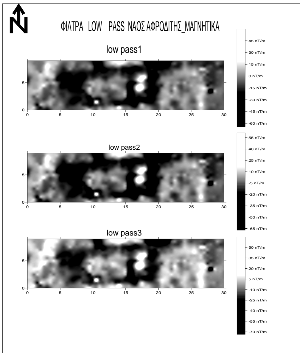
Σχήμα 4.2.1 φίλτρα low pass στο ναό Αφροδίτης-μαγνητικά.
