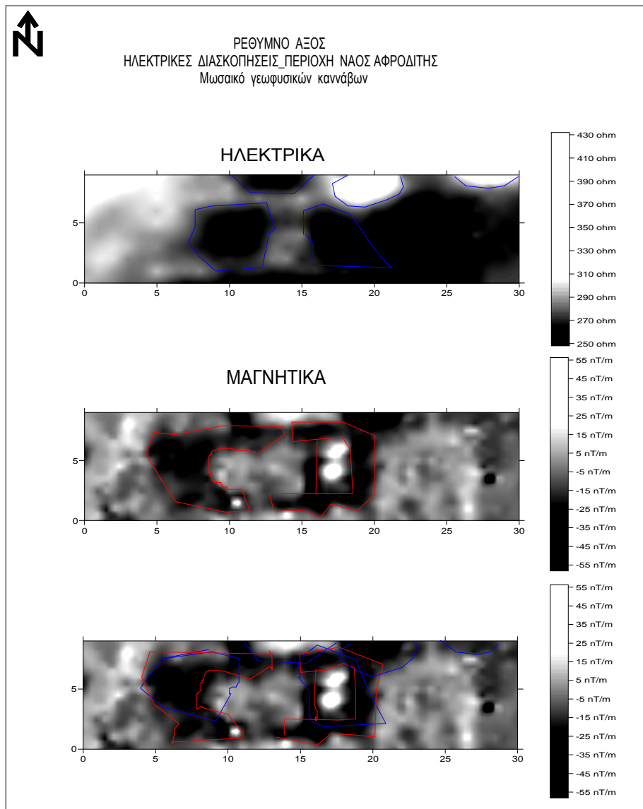
Σχήμα 4.3 χάρτης ερμηνείας Ναός Αφροδίτης
