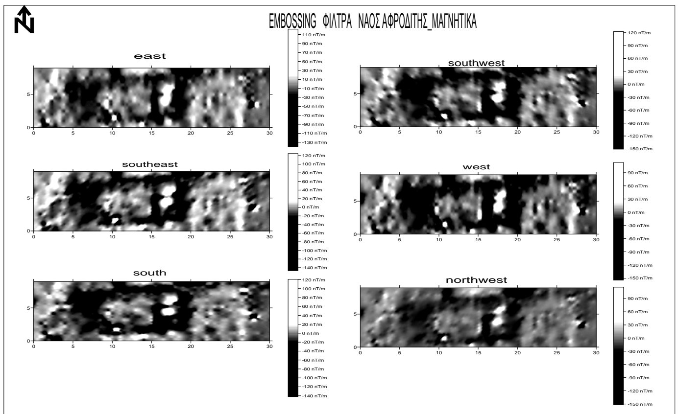
Σχήμα 4.2 φίλτρα διεύθυνσης για το ναό Αφροδίτης-μαγνητικά.
