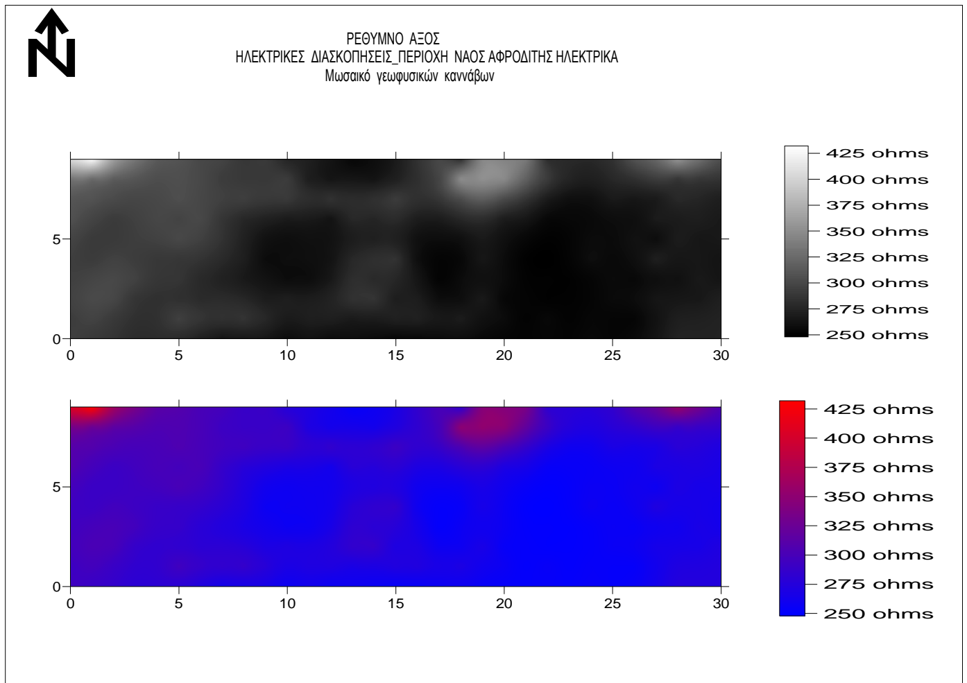
Σχήμα 4.1.2 περιοχή ναός Αφροδίτης ηλεκτρικά χωρίς συμπίεση.
