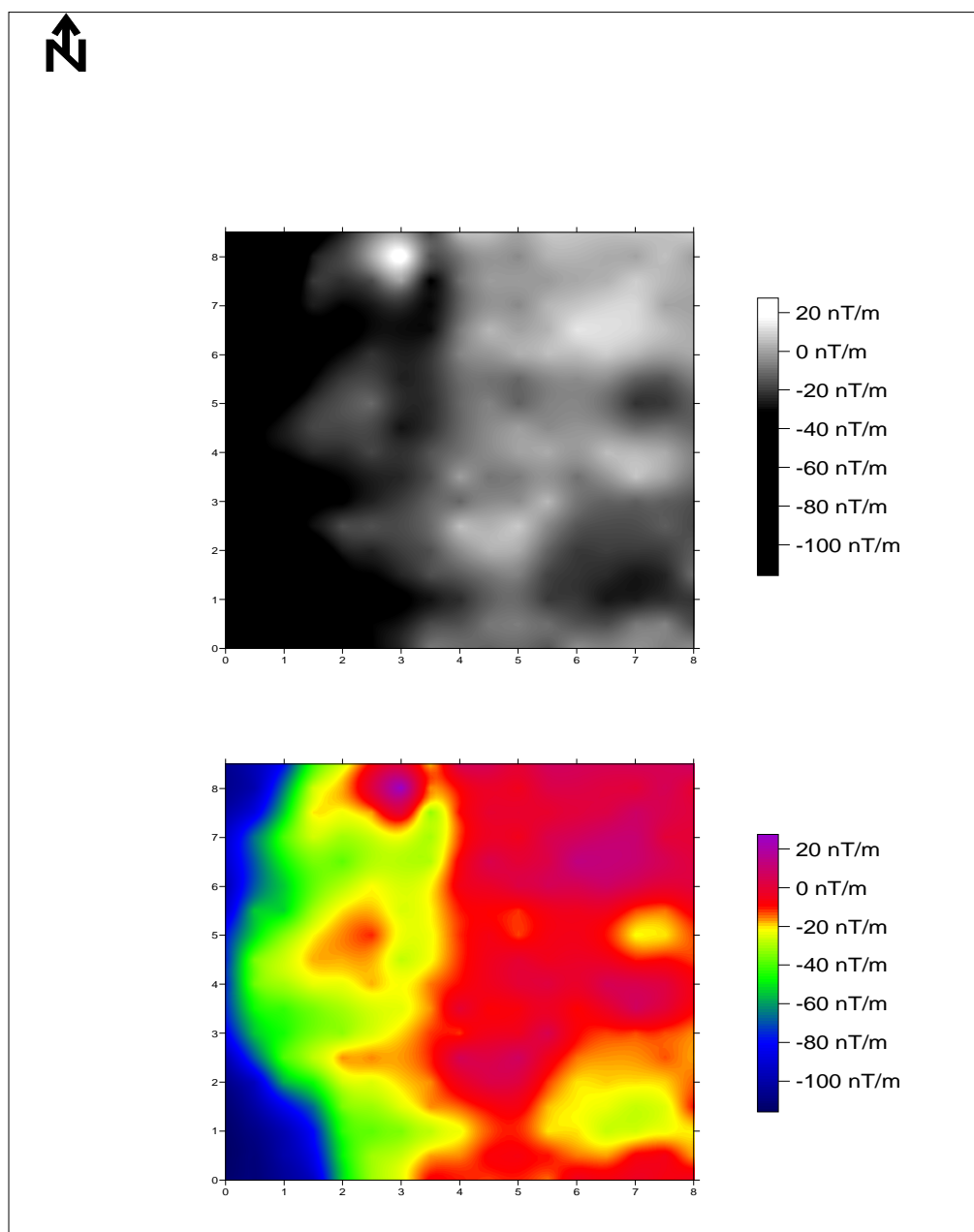
Σχήμα 4.4.2 περιοχή Ανδρείον 3B μαγνητικά με συμπίεση.
