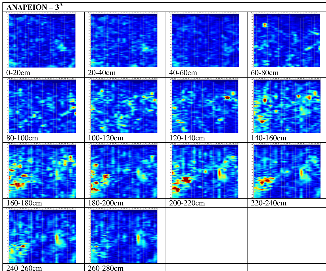
Σχήμα 4.4.3 Οριζόντιες τομές του υπεδάφους με αυξανόμενο βάθος (ανά 20cm) με τη χρήση του γεωραντάρ.
