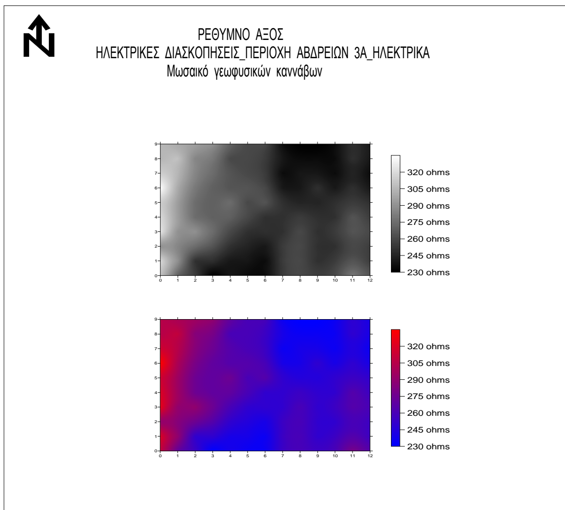
Σχήμα 4.3.1 περιοχή Ανδρείων 3Α ηλεκτρικά χωρίς συμπίεση.
