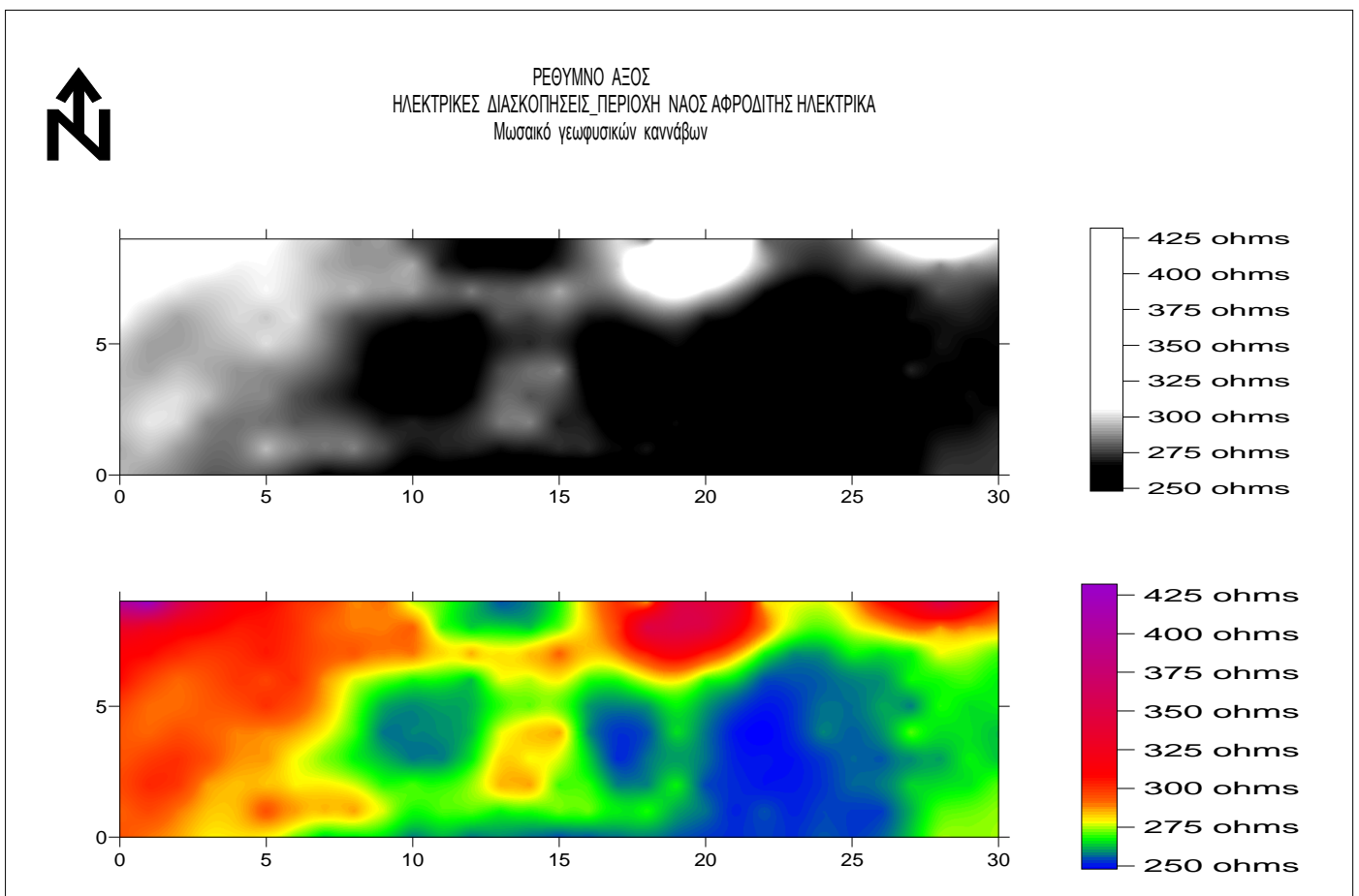
Σχήμα 4.1.3 περιοχή ναός Αφροδίτης ηλεκτρικά με συμπίεση.
