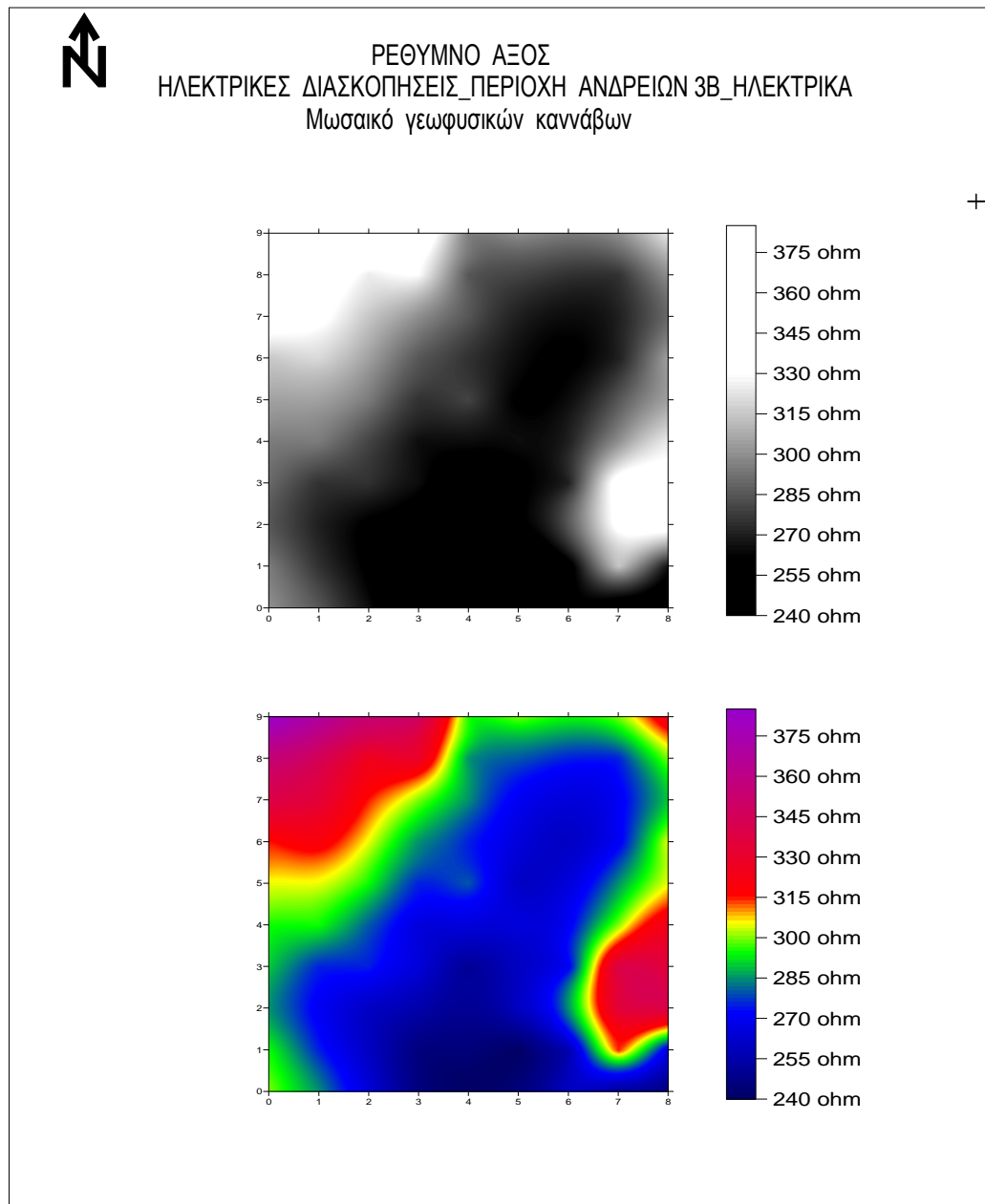
Σχήμα 4.3.4 περιοχή Ανδρείων 3B ηλεκτρικά με συμπίεση.
