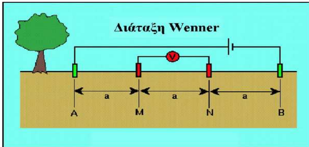
Σχήμα 2.3 Διάταξη Wenner
