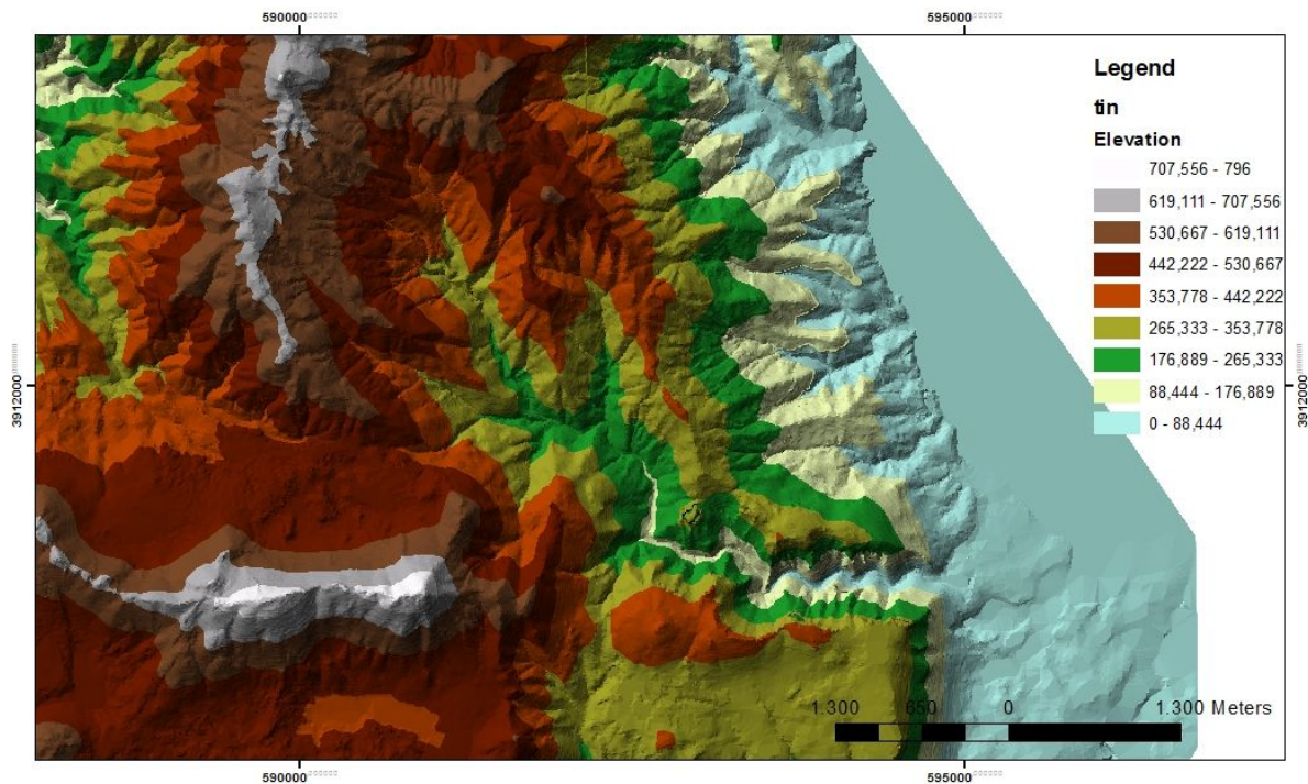
Σχήμα 1.1 Χάρτης που απεικονίζει την περιοχή μελέτης στο Ηράκλειο Κρήτης (με βάση το τοπογραφικό 1:5000 Γ.Υ.Σ.)
