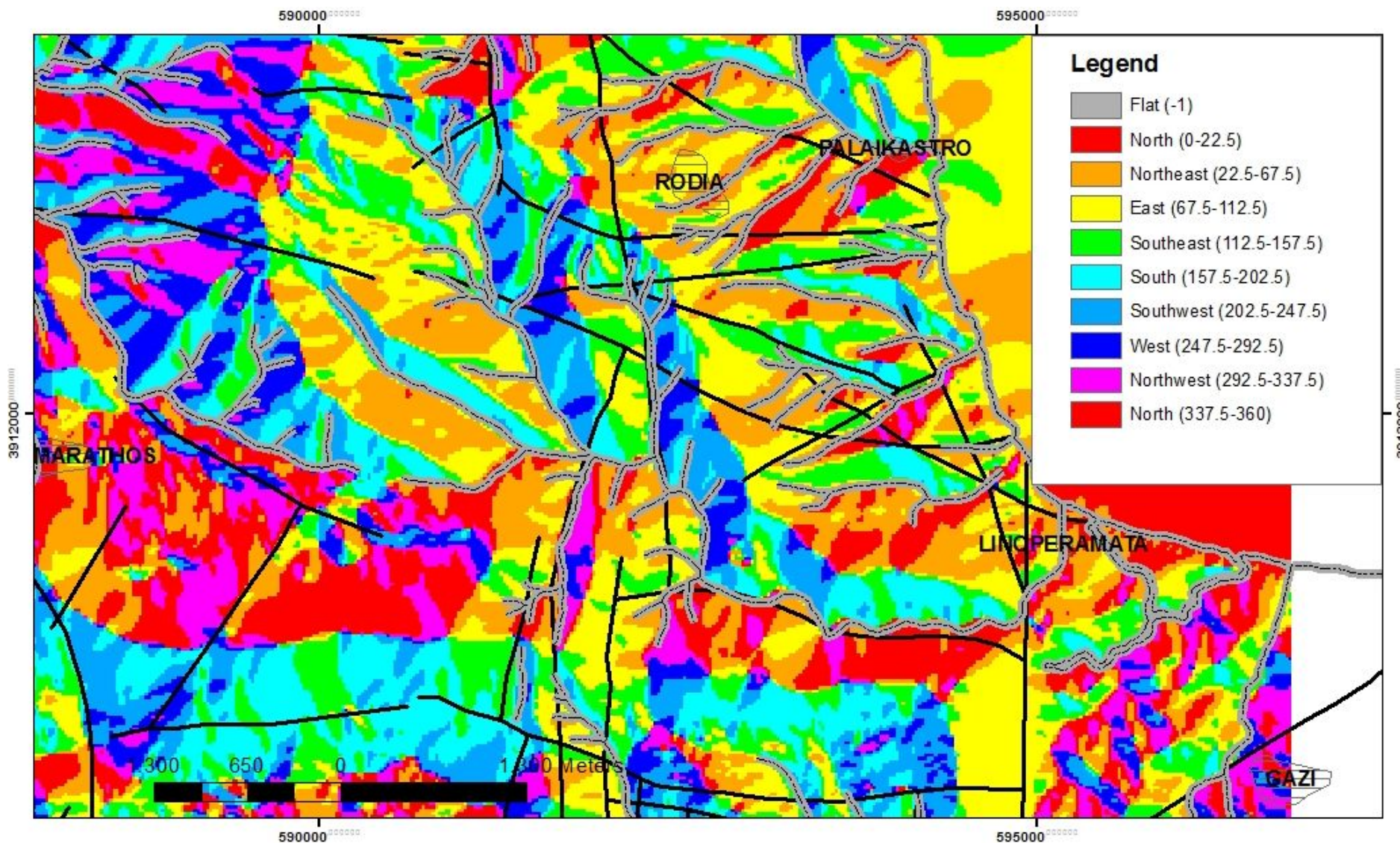
Σχήμα 4.3. Χάρτης διεύθυνσης κλίσης των επιφανειακών στοιχείων για την εξεταζόμενη περιοχή με υπέρθεση των ρηγματογενών ζωνών και του υδρογραφικού δικτύου
