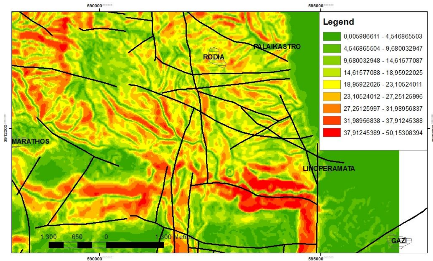
Σχήμα 4.2. α Χάρτης κλίσεων της εξεταζόμενης περιοχής, β με υπέρθεση των ρηξιγενών στοιχείων
