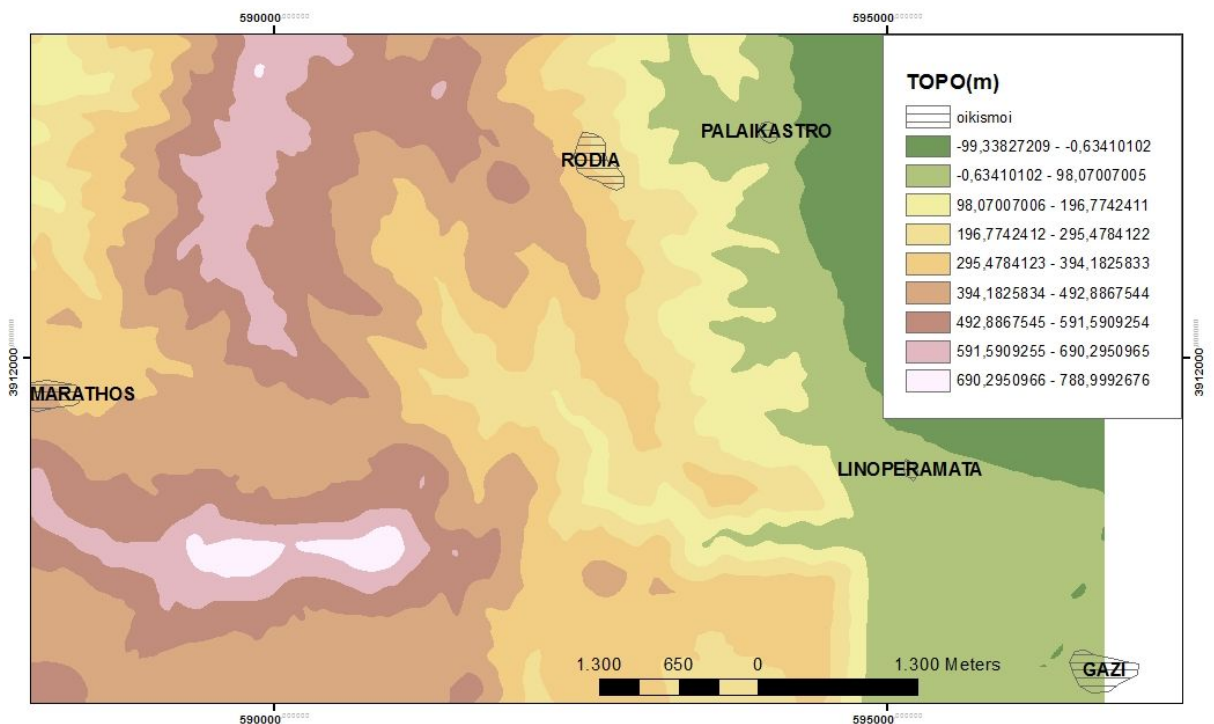
Σχήμα 4.1. Η εξεταζόμενη περιοχή
