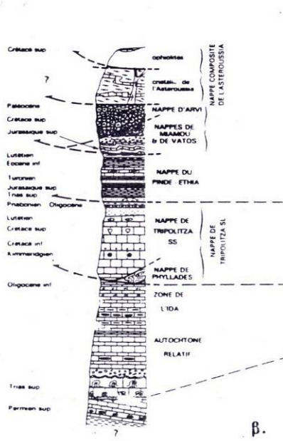
Σχήμα 2.1 α) Γεωλογικός χάρτης της Κρήτης κατά BONNEAU et al. (1977). 1. Νεογενή και Τεταρογενή, 2. Οφιολίθοι, 3. Κ. Αστερουσιών, 4. Κ. Μιαμούς, 5. Κ. Αρβης, 6. Κ. Πίνδου-Εθιάς, 7. Κ. Τρίπολης (α. Φυλλίτες-Χαλαζίτες), 8. Ζώνη Ιδας, β) και τεκτονοστρωματογραφικές στήλες των καλυμμάτων της Κρήτης, γ) κατά BONNEAU et al. (1977) και γ) κατά ΦΥΤΡΟΛΑΚΗ (1980).
