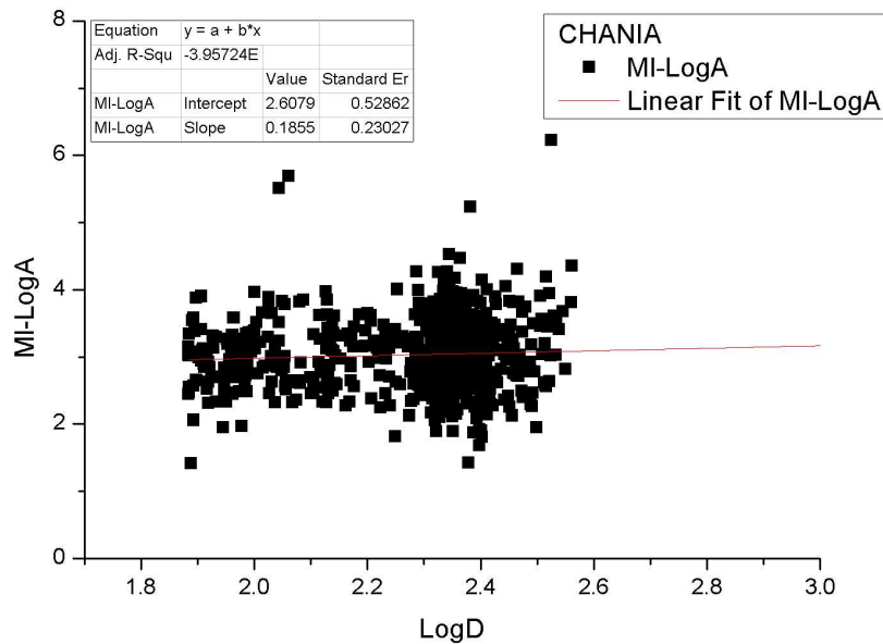
Σχήμα 3.1. Γραφική παράσταση του μεγέθους του σεισμού με βάση τον κατάλογο του ΝΟΑ σε σχέση με το λογάριθμο του πλάτους καταγραφής για το σταθμό των Χανίων.
