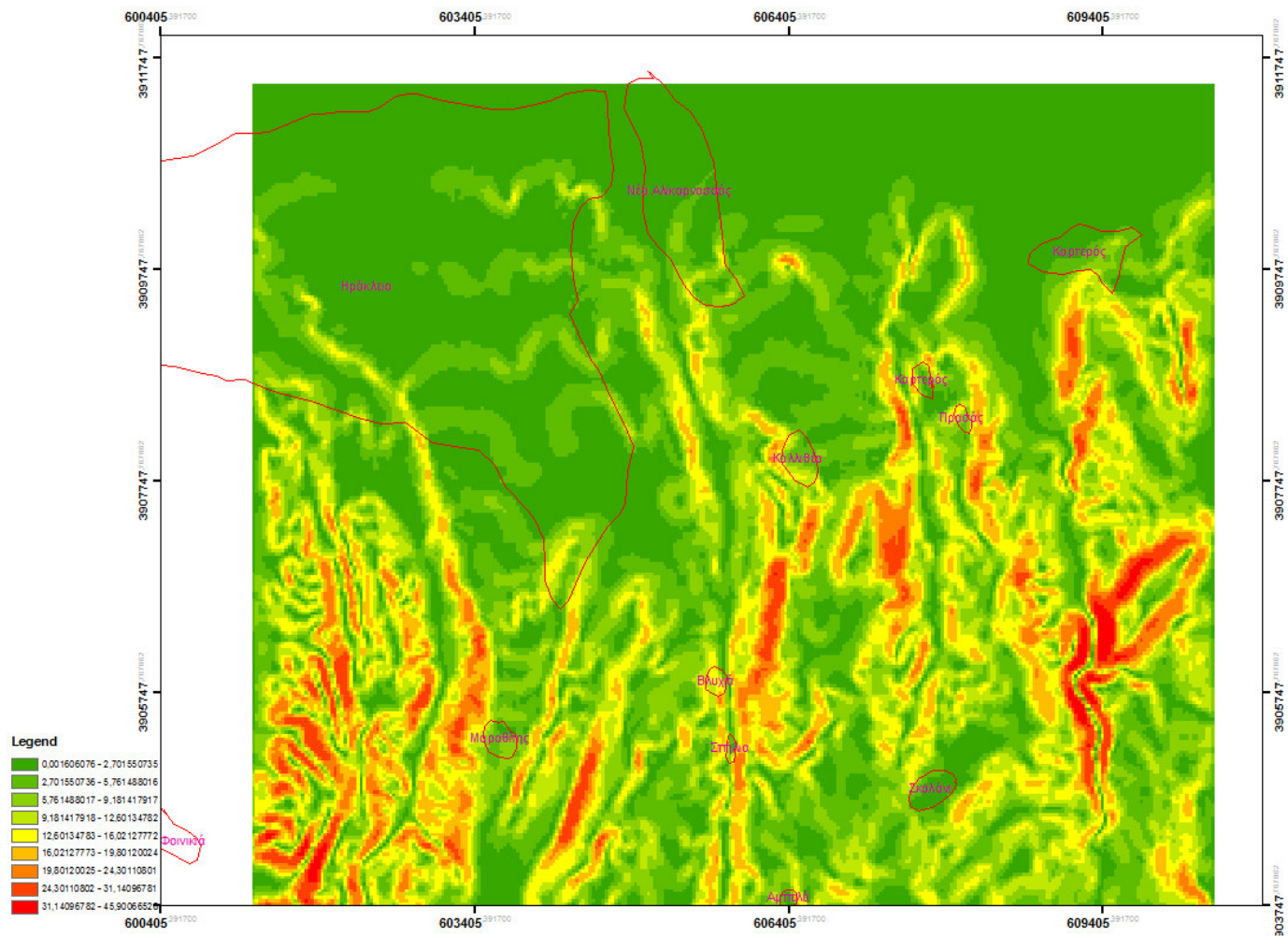
Σχήμα 4.2 Χάρτης κλίσεων
