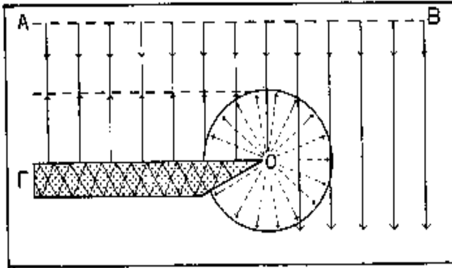
Σχήμα 21. Περίθλαση κύματος που προκαλείται στο άκρο O, ρηγματωμένου στρώματος ΟΓ (Kearey and Brooks 1984).
