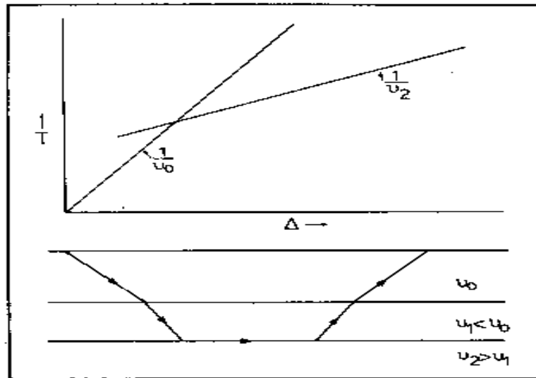
Σχήμα 33. Στρώμα μικρής ταχύτητας ( v ) μεταξύ δύο στρωμάτων μεγαλύτερων ταχυτήτων (κάτω) και αντίστοιχες καμπύλες χρόνων διαδρομής (πάνω). (Kearey and Books 1984).
