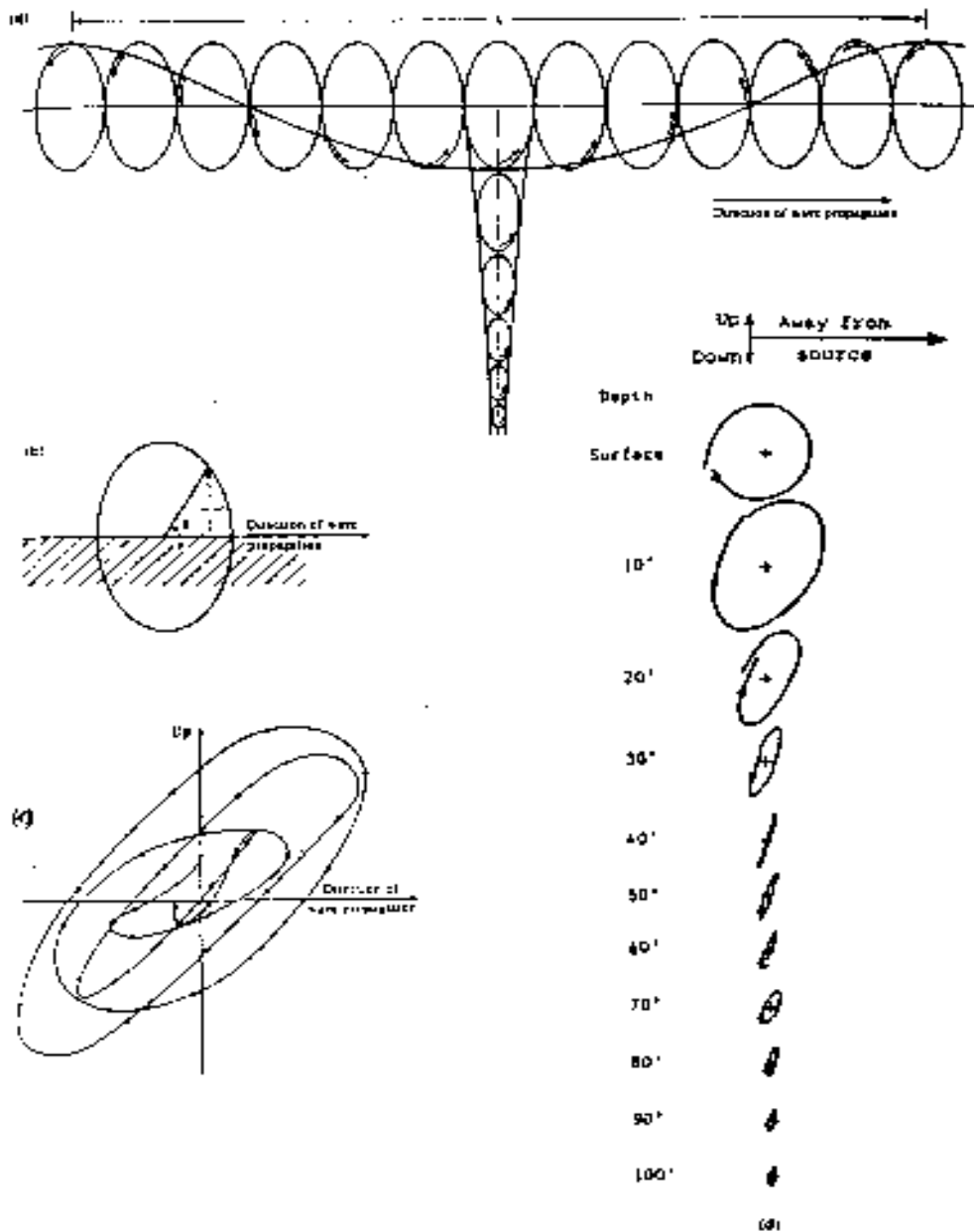
Σχήμα 14. Κύματα Rayleigh. (α) Κατακόρυφη τομή που απεικονίζει την κίνηση των κυμάτων στην επιφάνεια και την ελάττωση με το βάθος για ένα ημιχώρο, (b) Αναμενόμενη κίνηση στοιχειωδών μορίων της ύλης στην επιφάνεια του εδάφους, για ένα ημιχώρο, κατά την διάδοση επιφανειακών κυμάτων, (c) Πραγματική κίνηση στοιχειωδών μορίων της ύλης στην επιφάνεια του εδάφους (Howell, 1959), (d) Κίνηση των επιφανειακών κυμάτων που προκλήθηκαν από έκρηξη, όπως καταγράφηκαν από θαμμένα γεώφωνα : παρατηρείται ότι η κίνηση των υλικών σημείων είναι ανάστροφη μέχρι το βάθος των 40ft (0.192λ) (Dobrin, 1951).
