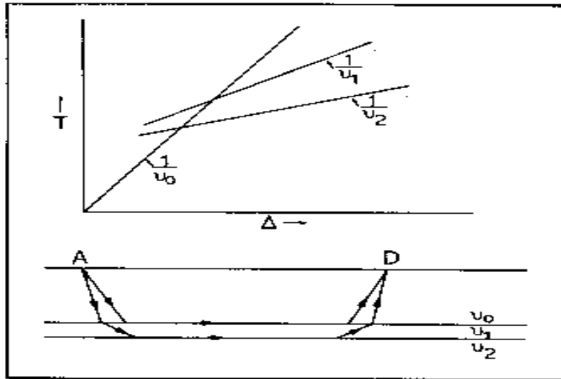
Σχήμα 32. Στρώμα μικρού πάχους (ταχύτητας u_0 ) μεταξύ δύο στρωμάτων σχετικά μεγάλων παχών (κάτω) και αντίστοιχες καμπύλες χρόνων διαδρομής (πάνω) (Kearey and Books 1984).
