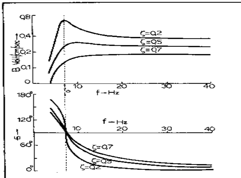
Σχήμα 24. Δυναμική μεγέθυνση, B, του γεωφώνου (πάνω) και διαφορά φάσης, \phi , μεταξύ ταχύτητας εδάφους και τάσης εξόδου του γεωφώνου (κάτω) σε συνάρτηση με τη συχνότητα ταλάντωσης του εδάφους για τρεις τιμές του παράγοντα απόσβεσης (Telford et al. 1976).
