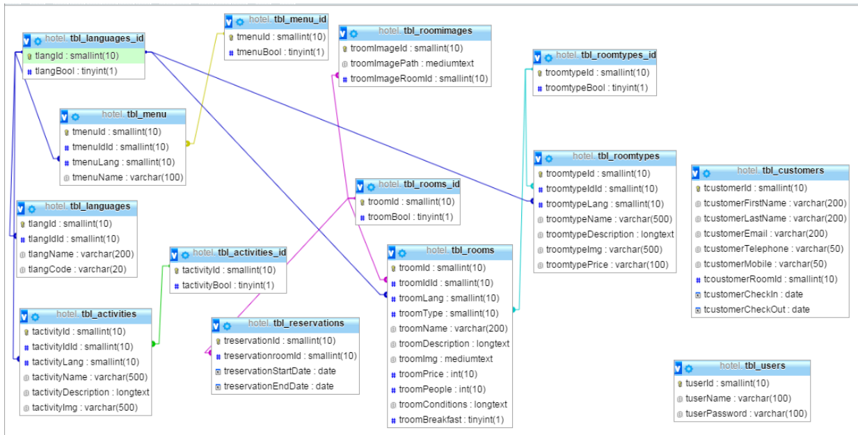
Εικόνα 16: Το σχήμα της βάσης δεδομένων
