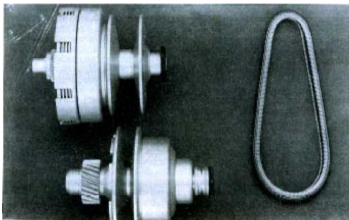
Σχήμα 3.7 Η δημιουργία της απαιτούμενης (για τη μετάδοση της κίνησης) τριβής μεταξύ του ιμάντα και των τροχαλιών δεν γίνεται με την πρόταση του ιμάντα αλλά με τη συμπίεση των πλαϊνών των μεταλλικών στοιχείων από τις παρειές της τροχαλίας
