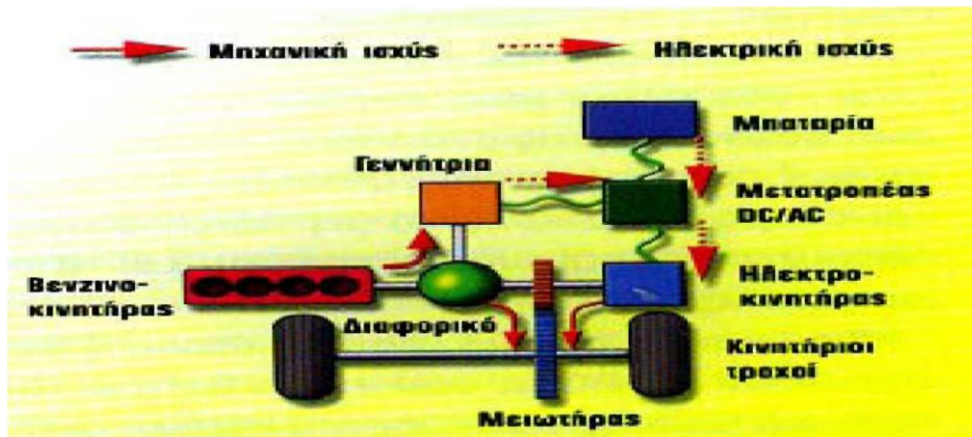
Σχήμα 4.3 Μικτή συνδεσμολογία σε υβριδικό όχημα
