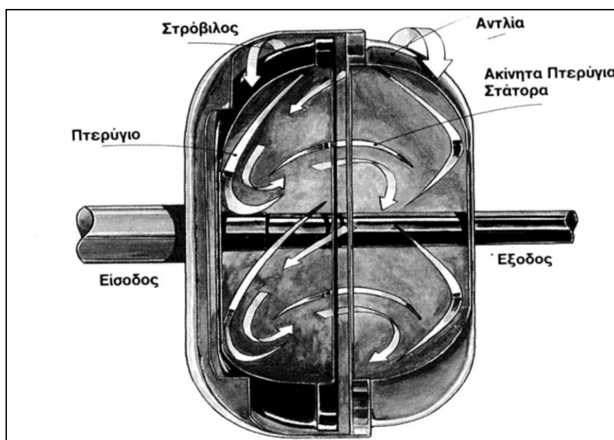
Σχήμα 3.3 Υδραυλικός μετατροπέας ροπής
