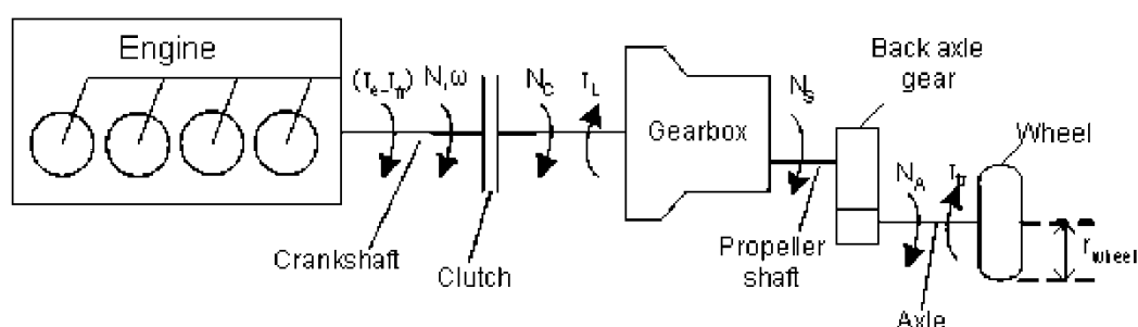
Σχήμα 3.1 Σχηματική απεικόνιση απλουστευμένης λειτουργίας συμβατικού οχήματος
