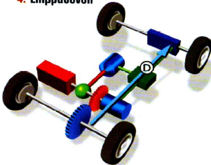
Σχήμα 5.19 Ροή ισχύος κατά την επιβράδυνση
