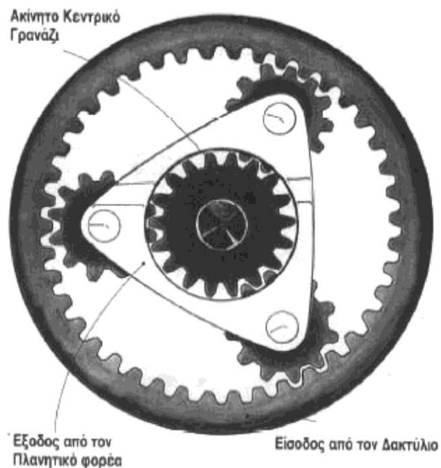
Σχήμα 3.4 Η μετάδοση της κίνησης μέσω επικυκλικού συστήματος
