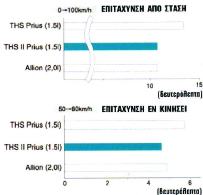
Σχήμα 6.7 Σύγκριση επιδόσεων του Prius THS II με το προηγούμενο THS αλλά και με ένα συμβατικό
