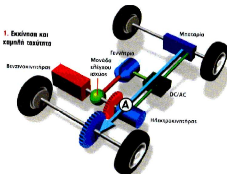
Σχήμα 5.16 Ροή ισχύος στην εκκίνηση και σε χαμηλές ταχύτητες
