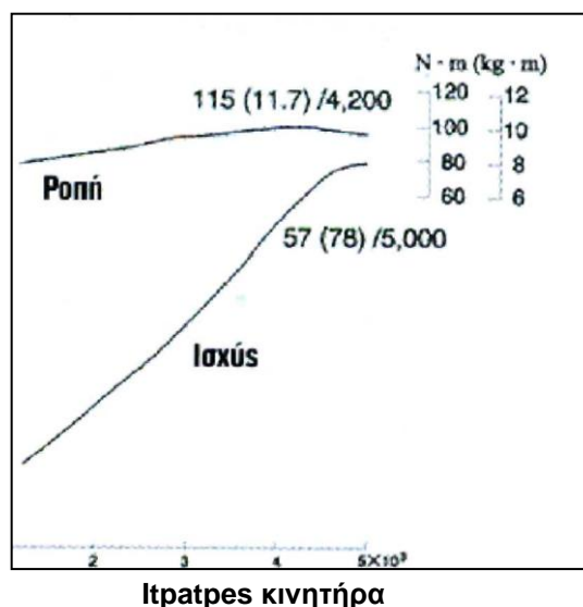
Σχήμα 6.9 Διάγραμμα ροπής και ισχύος του Prius THS II
