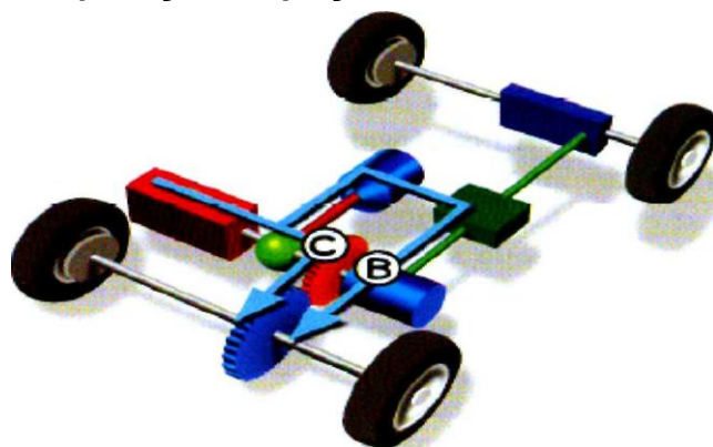
Σχήμα 5.17 Ροή ισχύος σε ομαλές συνθήκες οδήγησης
