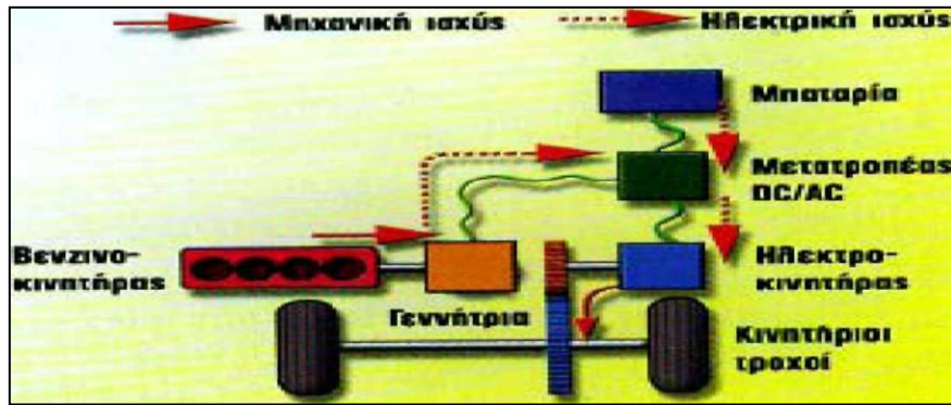
Σχήμα 4.1 Σειριακή συνδεσμολογία σε υβριδικό όχημα με βενζινοκινητήρα
