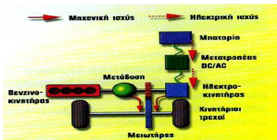
Σχήμα 4.2 Παράλληλη συνδεσμολογία σε υβριδικό όχημα
