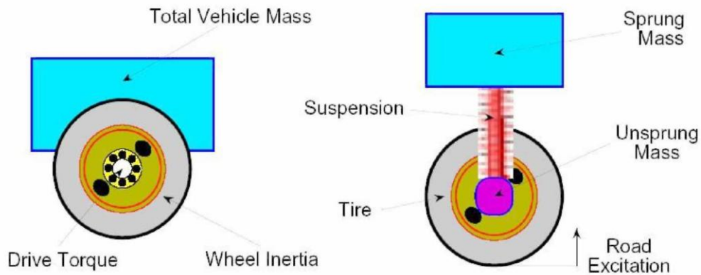
Σχήμα.3.8 Δυναμική οχήματος σε διαμήκεις (αριστερά) και καθ' ύψος (δεξιά) κατευθύνσεις
