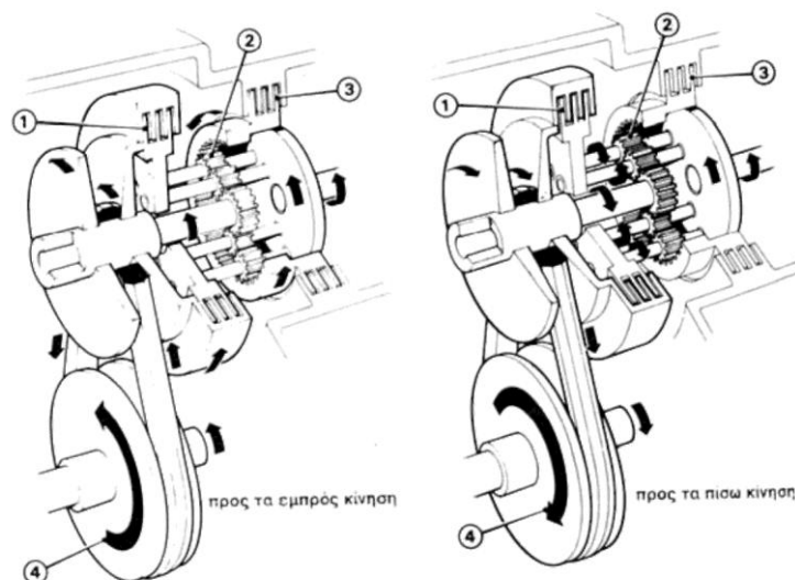
Σχήμα 3.6 Λειτουργία επικυκλικών γρاناζιών
