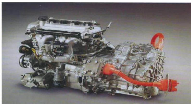
Σχήμα 6.10 Ρεαλιστική απεικόνιση του κινητήρα του Prius
