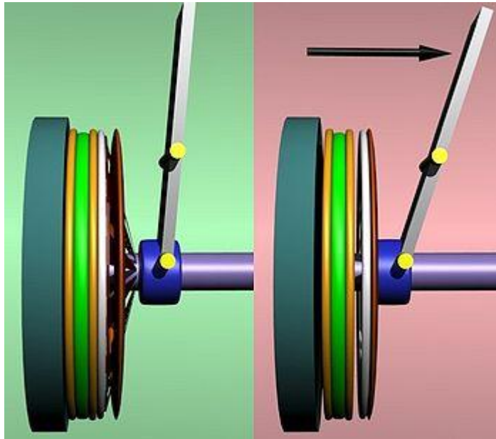
Λειτουργία του μηχανικού ξηρού συμπλέκτη τριβής-Αποσύμπλεξη
