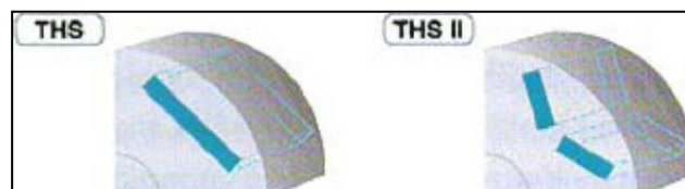
Σχήμα 6.5 Η προηγούμενη και η νέα βελτιωμένη διάταξη των μαγνητών νεοδυμίου στον ηλεκτροκινητήρα
