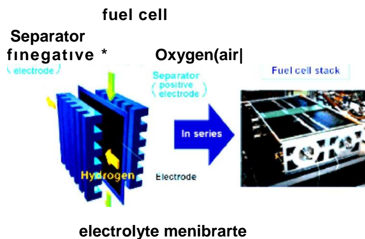
Σχήμα 4.6 Η δομή μιας κυψέλης καυσίμου
