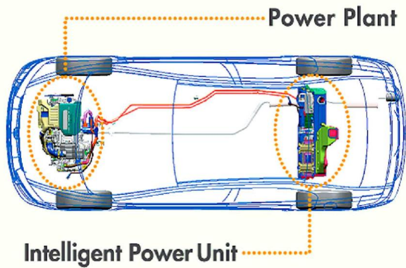
Σχήμα 7.21 Το υβριδικό σύστημα του Honda Civic
