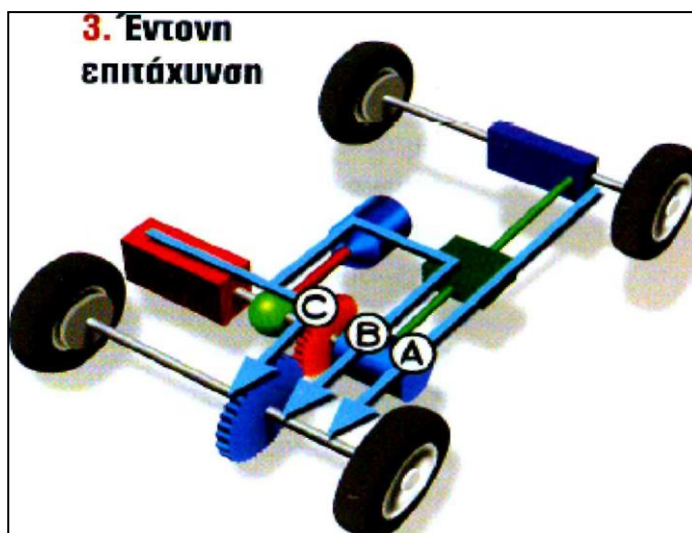
Σχήμα 5.18 Ροή ισχύος στη διάρκεια έντονης επιτάχυνσης
