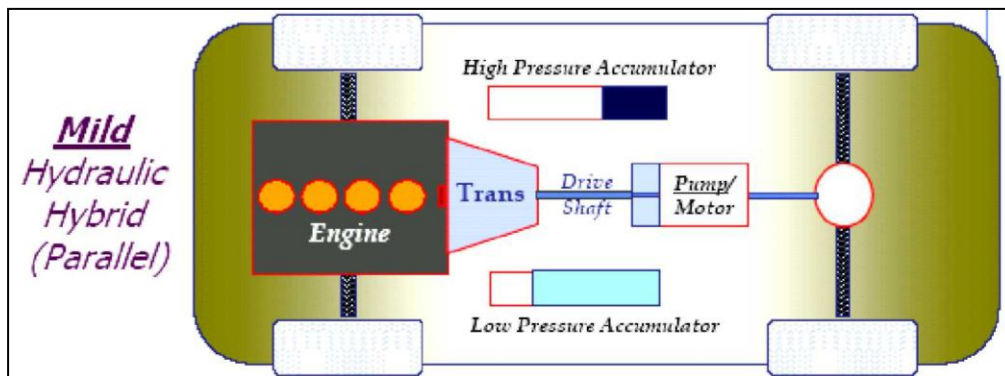
Σχήμα 4.13 Το Υδραυλικό Βοηθητικό Σύστημα Προώθησης σε υδραυλικό υβριδικό όχημα
