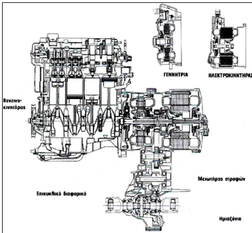
Σχήμα 6.1 Το ηλεκτρομηχανικό μέρος του THS
