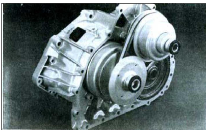
Σχήμα 3.5 Όταν η διάμετρος της τροχαλίας του κινητήρα έχει τη μικρότερη διάμετρο (και η δεύτερη τη μεγαλύτερη), τότε το CVT διαθέτει την "κοντύτερη" σχέση μετάδοσης. Στην ακριβώς αντίθετη περίπτωση το CVT λειτουργεί με τη "μακρύτερη" δυνατή σχέση.
