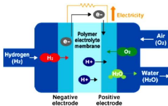
Σχήμα 4.5 Σχηματική αναπαράσταση λειτουργίας μιας κυψέλης καυσίμου
