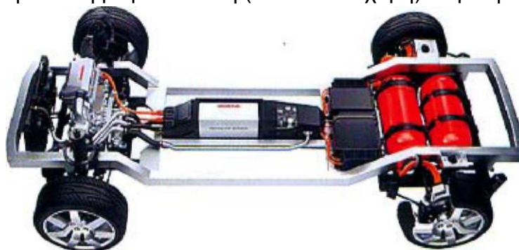
Σχήμα 4.11 Το πλαίσιο και τα ηλεκτρομηχανικά μέρη του FCX Concept
