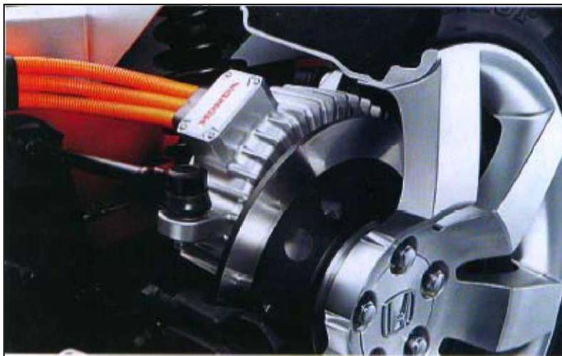
Σχήμα 4.9 Οι μικροί "in-hub" ηλεκτροκινητήρες των πίσω τροχών, ισχύος 25kW ο καθένας. ("έκκεντρα") στο εσωτερικό των πίσω τροχών.
