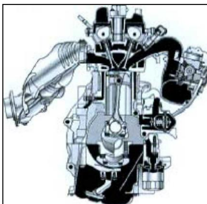
Σχήμα 6.8 Ο κινητήρας του Prius είναι υποτετράγωνος, με το στροφαλοφόρο τοποθετημένο ελαφρά πιο «πίσω» από το νοητό επίπεδο των αξόνων των κυλίνδρων
