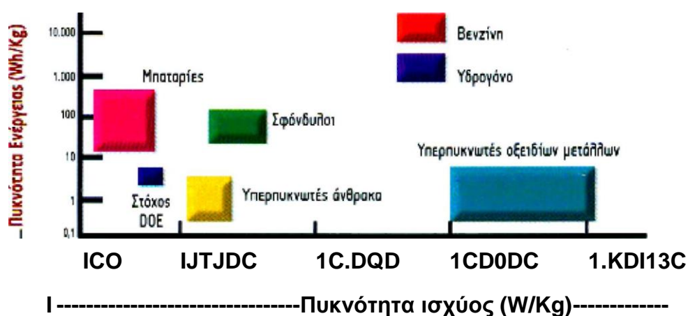
Σχήμα 5.11 Συγκριτική παράθεση πυκνότητας ενέργειας (ενέργεια ανά κιλό μάζας) και πυκνότητας ισχύος (αποδιδόμενη ισχύς ανά κιλό μάζας) για τις καθιερωμένες μορφές αποθήκευσης ενέργειας αλλά και δυο καύσιμα, του παρόντος και του μέλλοντος ( βενζίνη και υδρογόνο).
