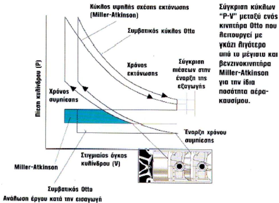
Σχήμα 5.15 Σύγκριση κύκλων P-V μεταξύ κινητήρων Otto και Atkinson
