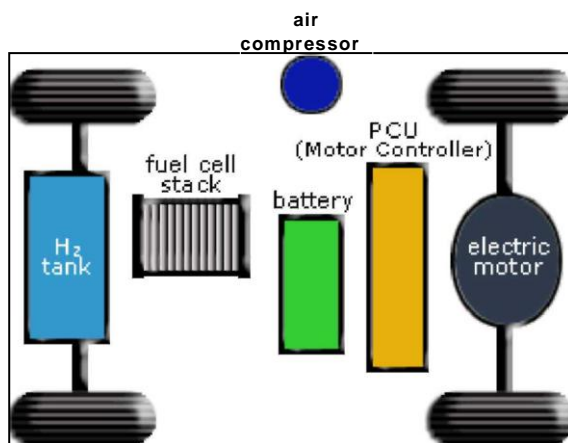
Σχήμα 4.7 Βασικά στοιχεία ενός υδρογονικού FCV
