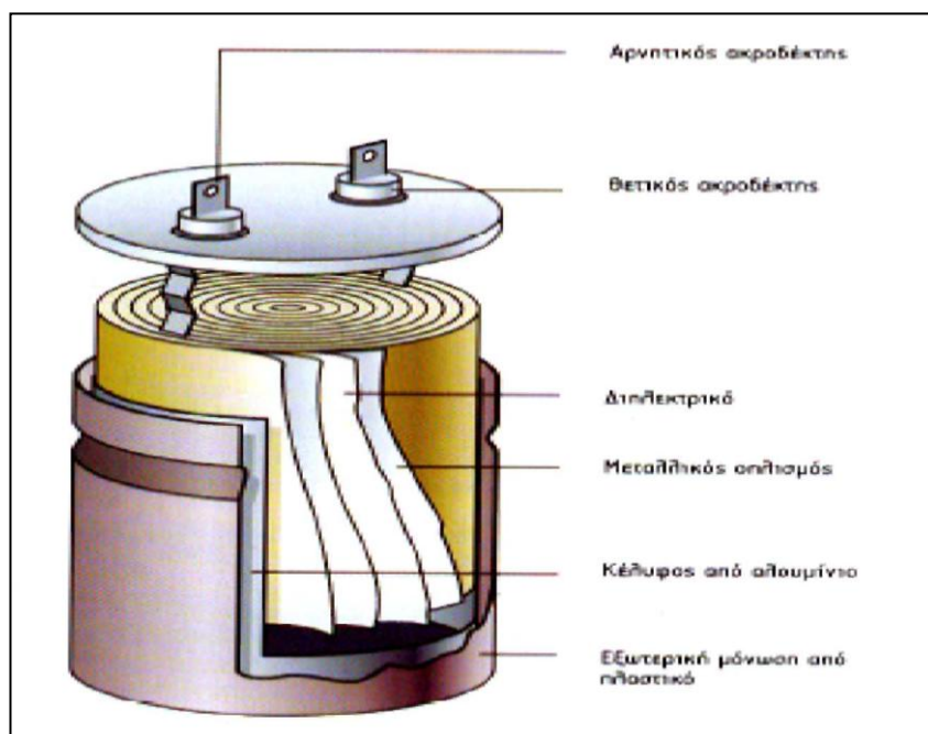
Σχήμα 5.7 Τυπική μορφή συμβατικού πυκνωτή
