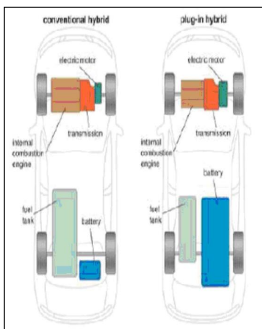
Σχήμα 5.2 Σύγκριση συστήματος ενός HEV και ενός PHEV
