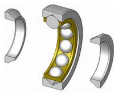
Ωστικός τριβέας
