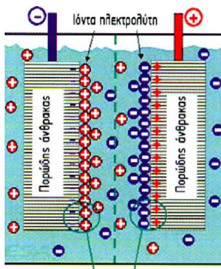
Σχήμα 5.10 Σχηματική παράσταση ενός υπερπυκνωτή διπλού στρώματος σε "ώρα εργασίας".
