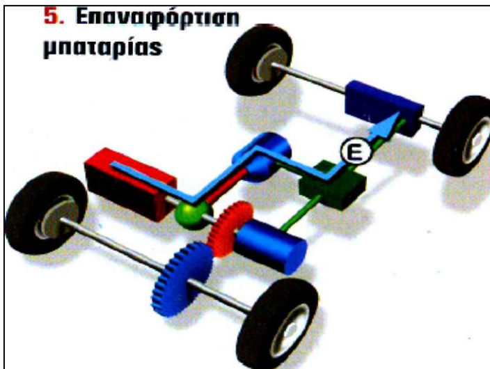
Σχήμα 5.20 Ροή ισχύος κατά την ακινησία οχήματος
