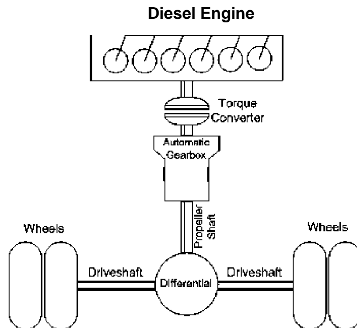
Σχήμα 3.2 Σχηματική απεικόνιση μετάδοσης ισχύος σε φορτηγό με αυτόματο κιβώτιο ταχυτήτων
