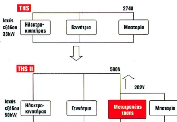
Σχήμα 6.6 Αύξηση της απόδοσης του ηλεκτροκινητήρα μέσω της προσθήκης ενός μετατροπέα τάσης στο THS II.
