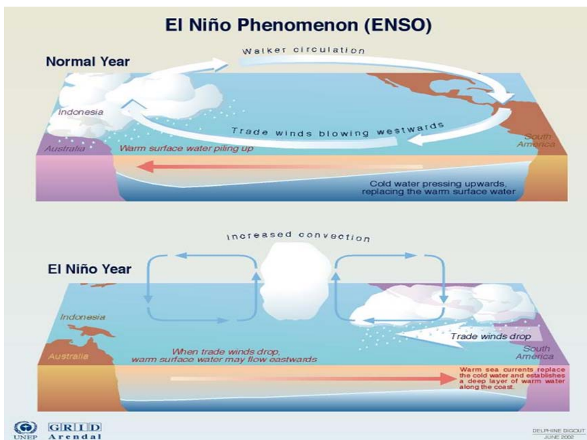
Εικόνα 10: Το φαινόμενο του Ελ Νίνο
