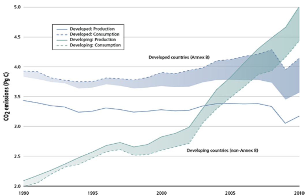
Εικόνα 7: Εκπομπές διοξειδίου του άνθρακα στις αναπτυγμένες και αναπτυσσόμενες χώρες (1990-2010)
