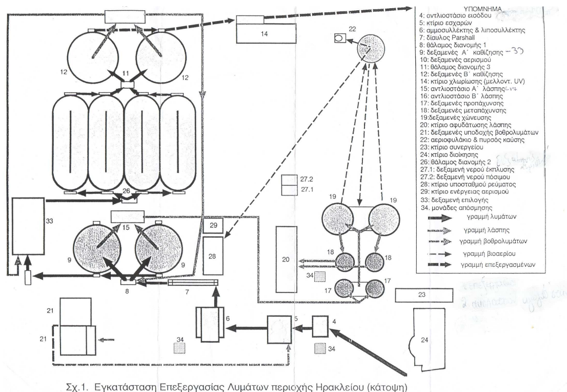
Σχ.1. Εγκατάσταση Επεξεργασίας Λυμάτων περιοχής Ηρακλείου (κάτοψη)
