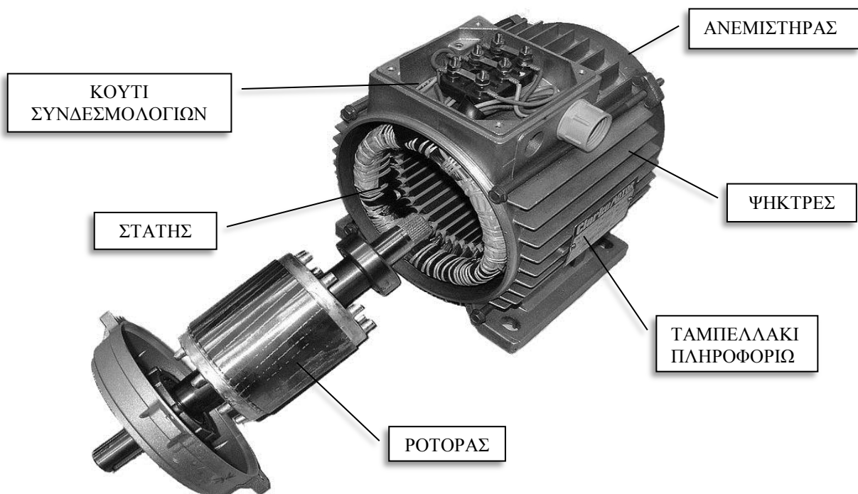
Εικόνα 2.1: βασικά μέρη ηλεκτρικού κινητήρα
