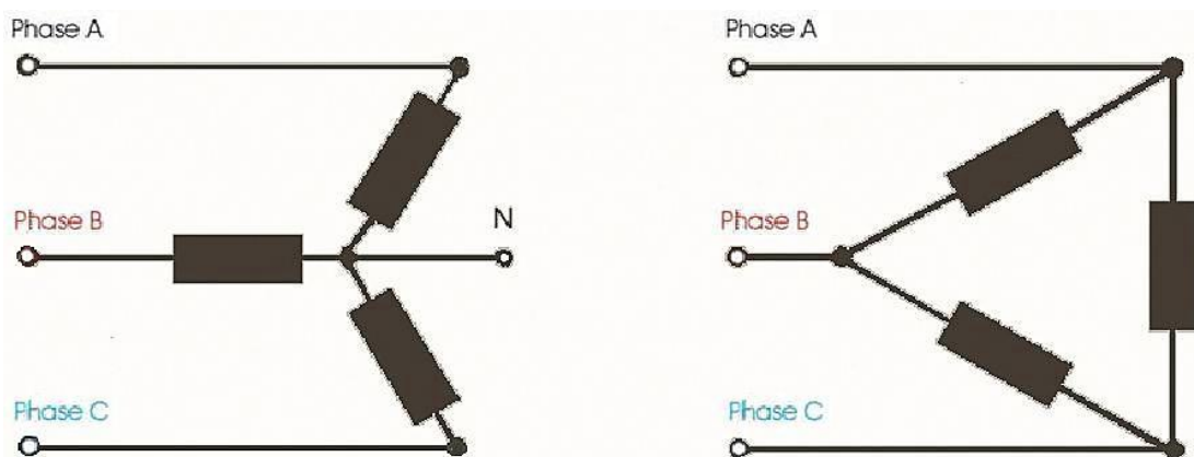
Εικόνα 2.8: Συνδεσμολογίας Αστέρα και Συνδεσμολογίας Τριγώνου αντίστοιχα
