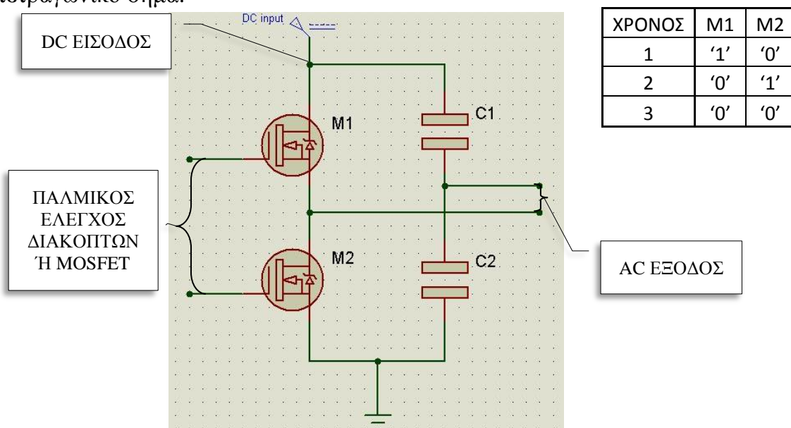
Εικόνα 4.1: αντιστροφέας μισής γέφυρας (half-bridge inverter)
