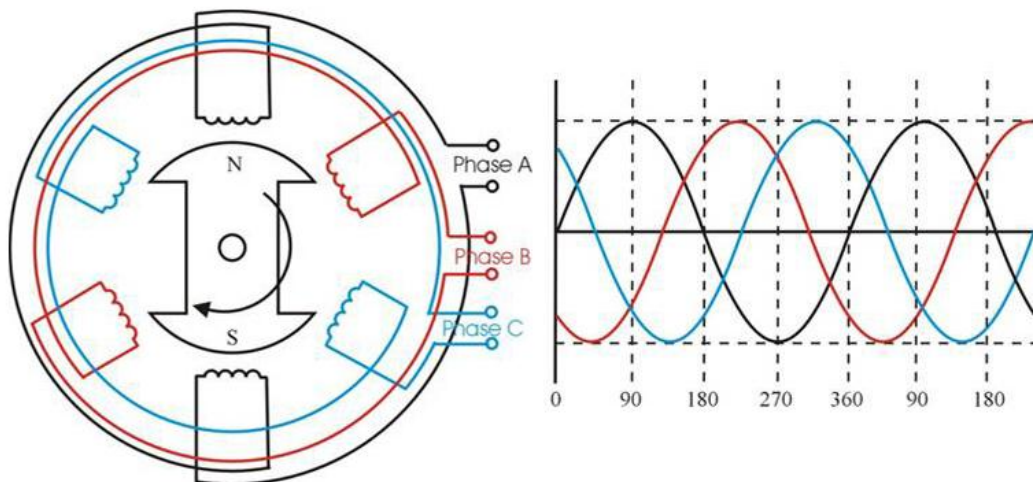
Εικόνα 2.6: τριφασική λειτουργία κινητήρα
