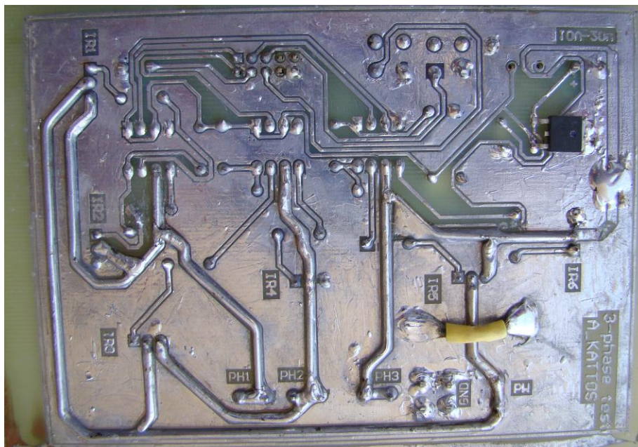
Εικόνα 5.2: κάτω όψη κυκλώματος με τρεις αντιστροφείς μισής γέφυρας
