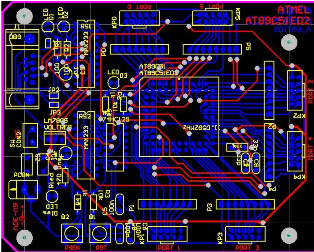
Εικόνα 5.3: PCB αναπτυξιακού κυκλώματος μικροεπεξεργαστή Atmel AT89C51ED2
