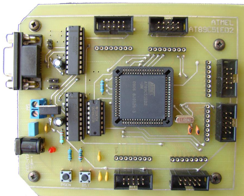
Εικόνα 5.5: πάνω όψη αναπτυξιακού κυκλώματος
