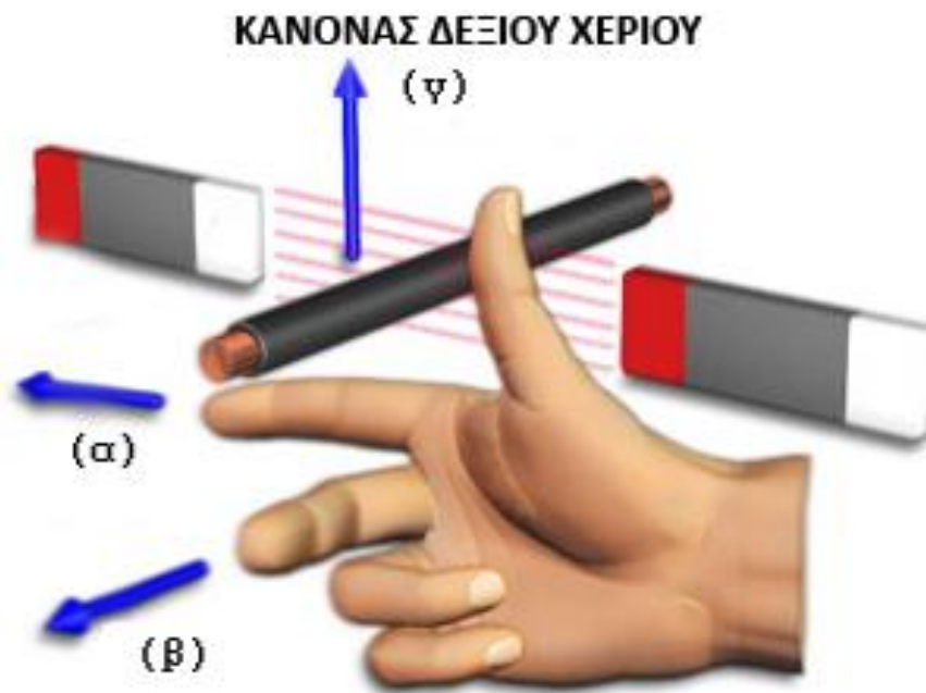
Εικόνα 2.2: κανόνας δεξιού χεριού
