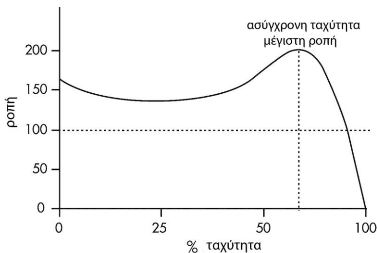
Εικόνα 2.13: γραφική παράσταση Ροπής – Ταχύτητας
