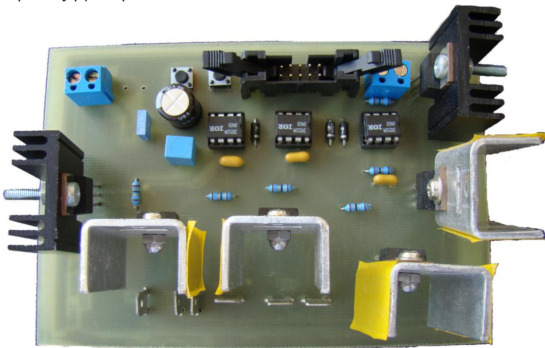
Εικόνα 5.1: πάνω όψη κυκλώματος με τρεις αντιστροφείς μισής γέφυρας
