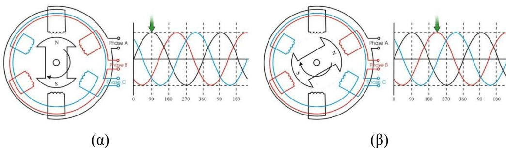
Εικόνα 2.6: τριφασική λειτουργία κινητήρα
