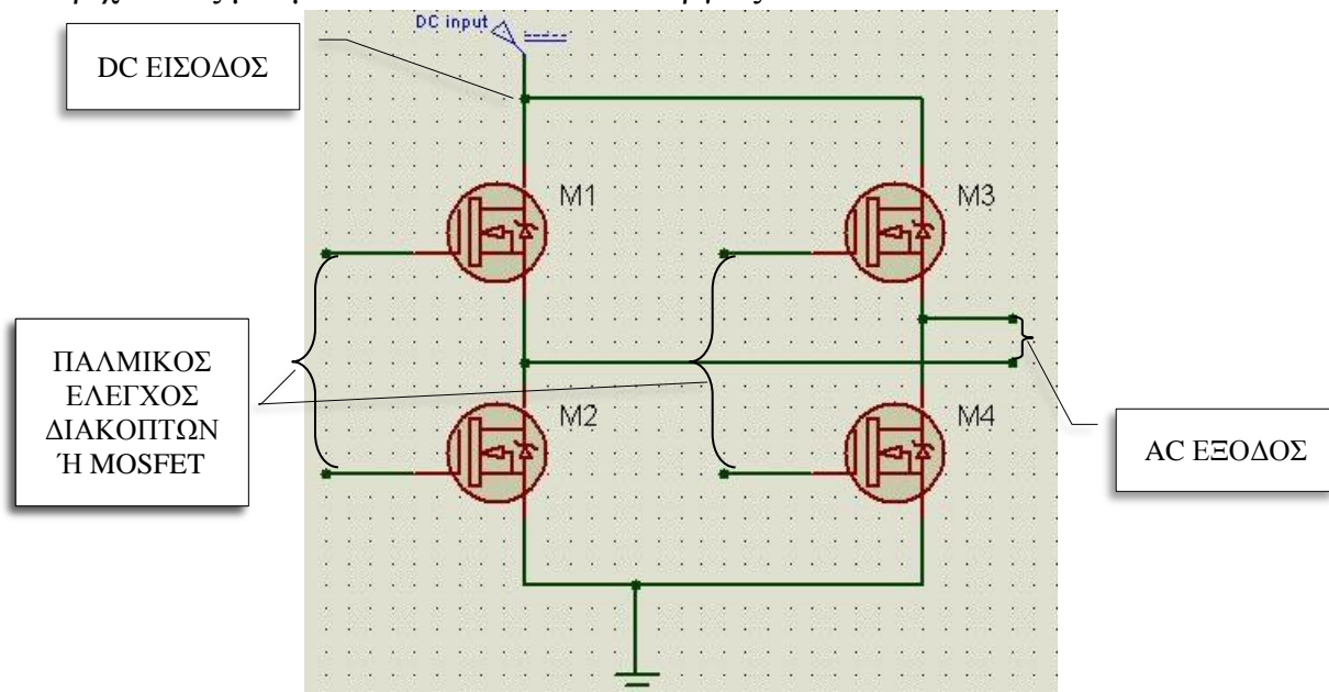
Εικόνα 4.2: αντιστροφέας πλήρης γέφυρας (full-bridge inverter)
