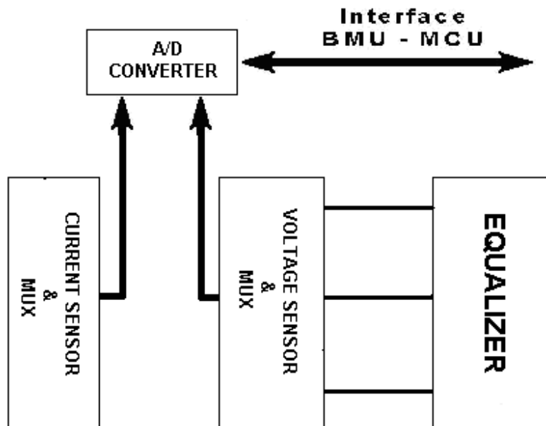
Σχ. 4.3 Τα μέρη της BMU
