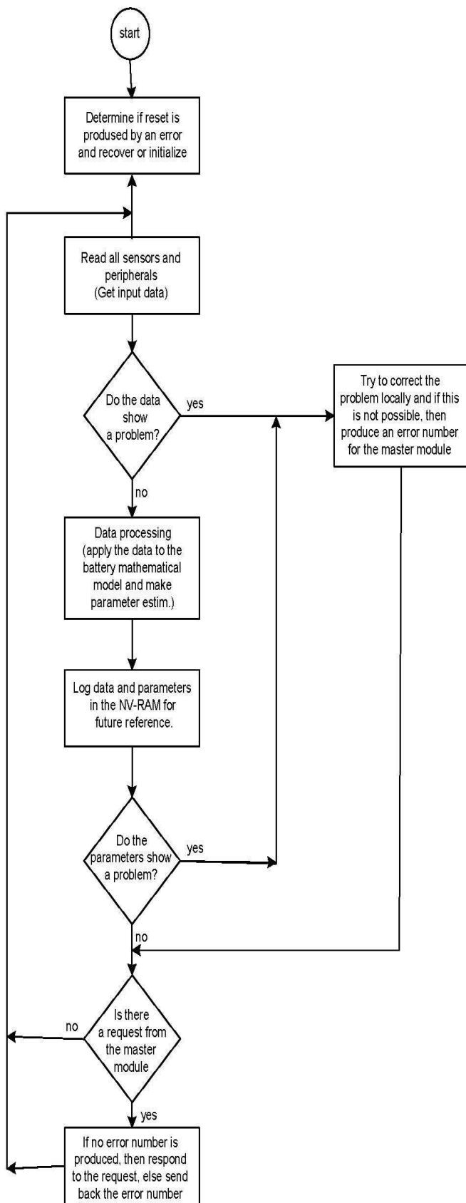
Σχ. 4.2 Flow chart του κώδικα του SBM
