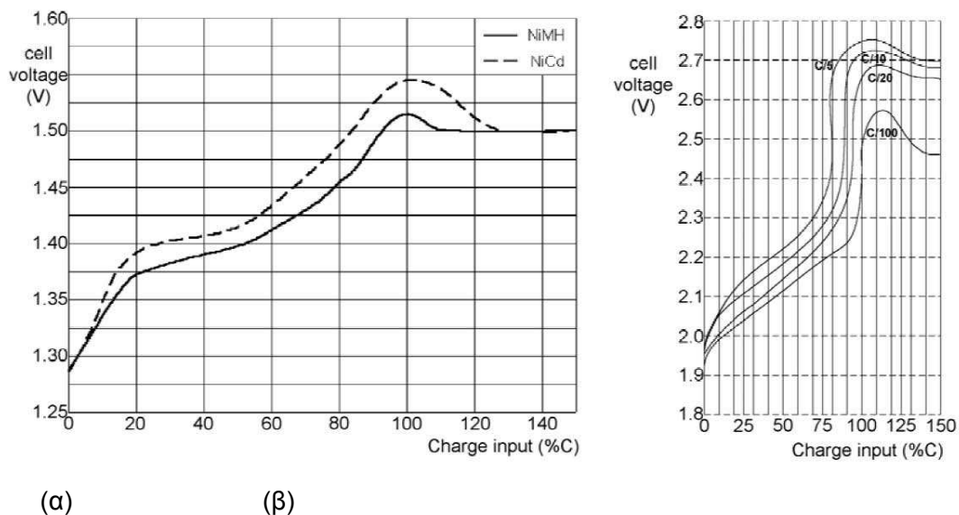
Σχ. 1.2. Χαρακτηριστικές καμπύλες φόρτισης στοιχείων (α) με αλκαλικό ηλεκτρολύτη (β) μολύβδου-οξέος
