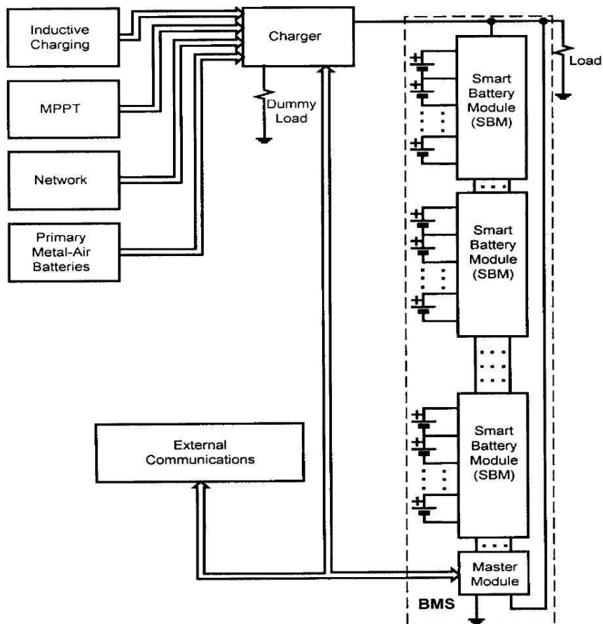
Σχ. 1.4 Block διάγραμμα τοπολογίας ενός τυπικού BMS
