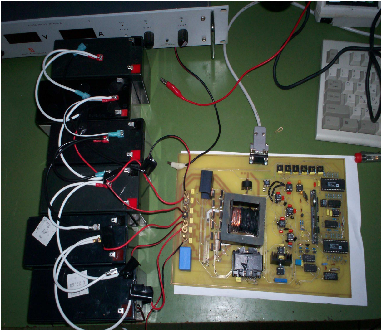
Φωτ. 4.4 Τελικό σύστημα (BMS)
