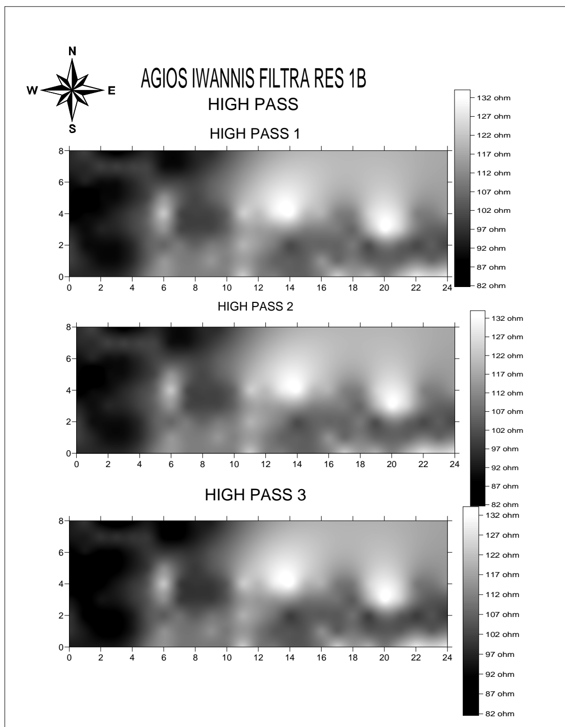
Σχήμα 4.2.2 φίλτρα high pass Άγιος Ιωάννης 1β-ηλεκτρικά.
