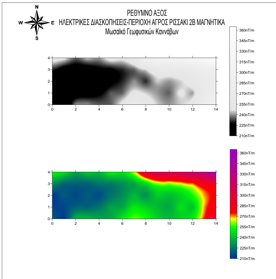
Σχήμα 4.4.2 περιοχή Αγρός Ρισσάκι 2B μαγνητικά με συμπίεση.
