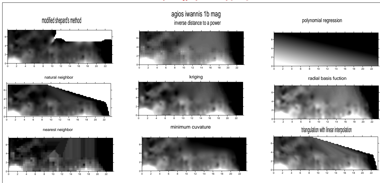
Σχήμα 4.2.4 εφαρμογή του grid data στον Άγιο Ιωάννη 1β με διαφορές από τις παραπάνω μεθόδους.
