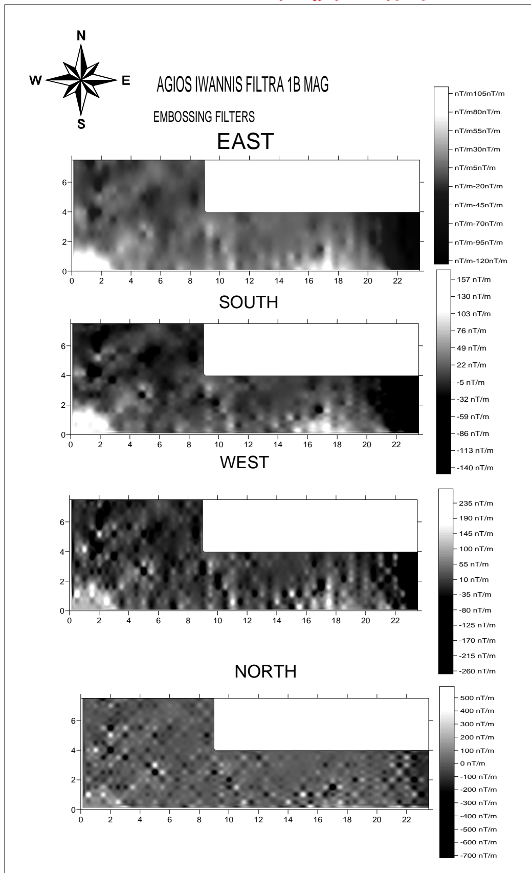
Σχήμα 4.2 φίλτρα διεύθυνσης για τον Άγιο Ιωάννη 1β.
