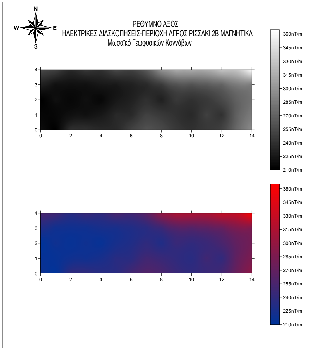
Σχήμα 4.4.1 περιοχή Αγρός Ρισσάκι 2B μαγνητικά χωρίς συμπίεση.
