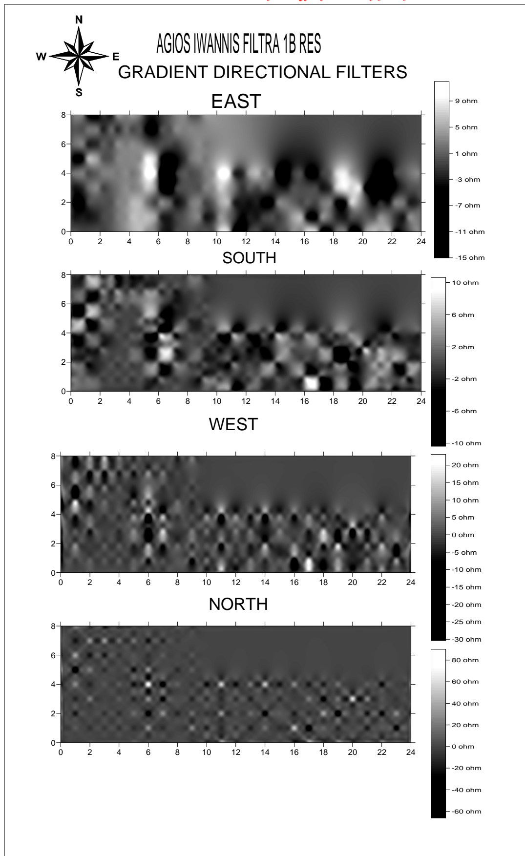
Σχήμα4.2.3 φίλτρα διεύθυνσης Αγιος Ιωάννης 1β -ηλεκτρικά.
