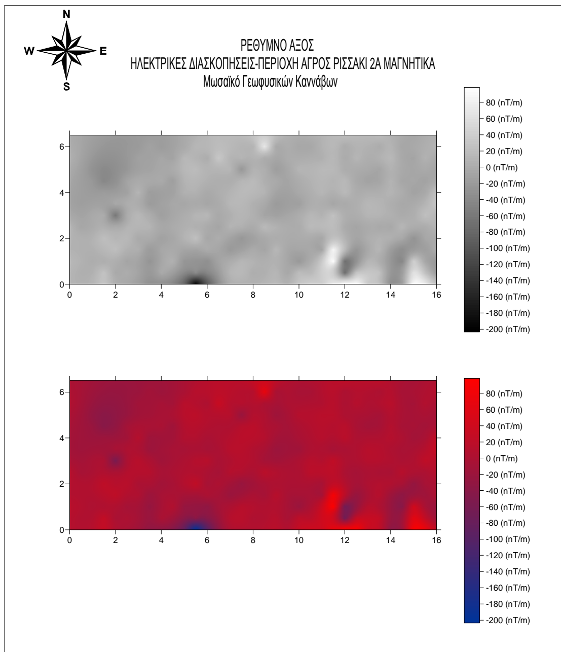
Σχήμα 4.3.5 περιοχή Αγρός Ρισσάκι 2Α μαγνητικά χωρίς συμπίεση.
