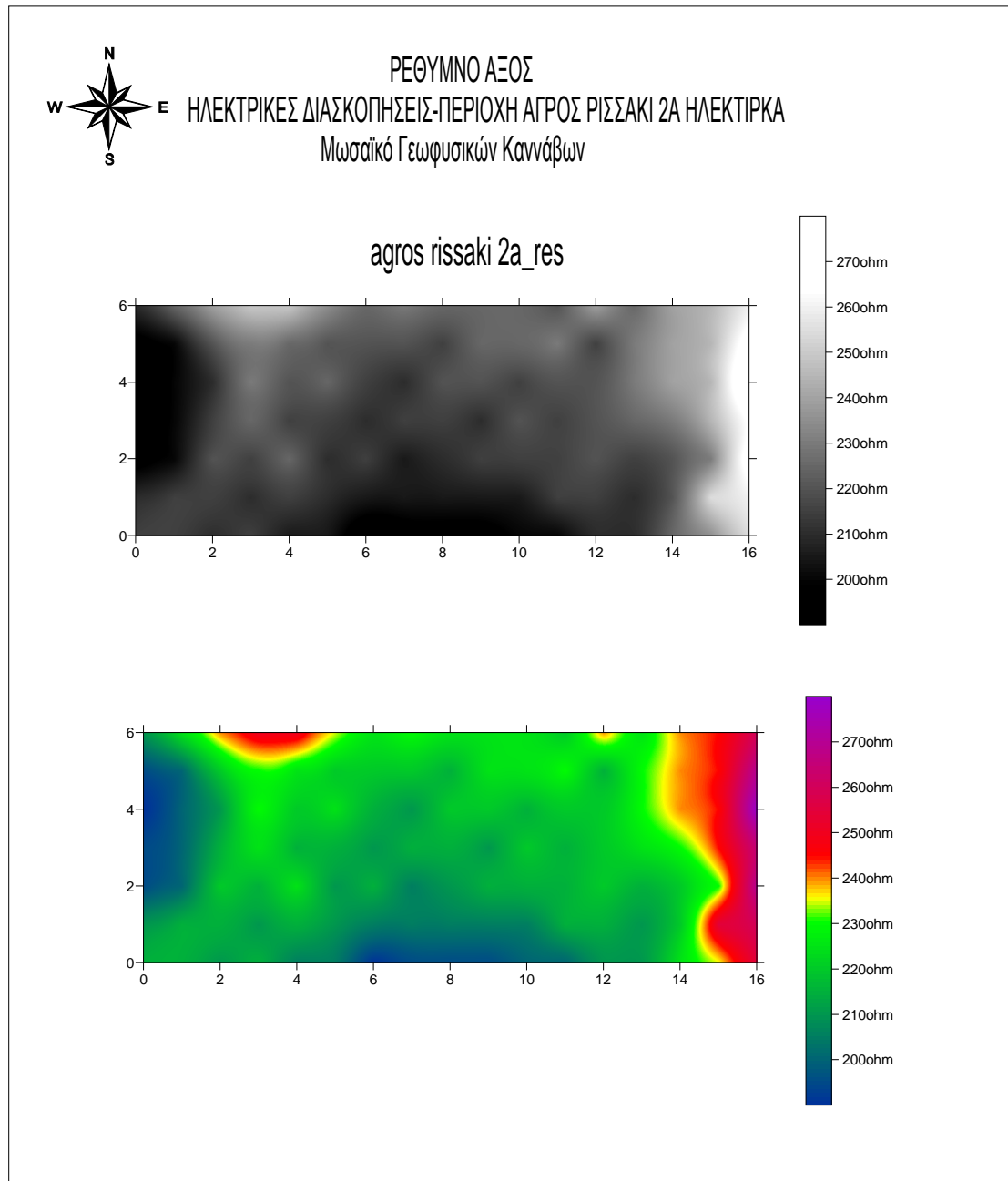
Σχήμα 4.3.2 περιοχή Αγρός Ρισσάκι 2α ηλεκτρικά με συμπίεση.
