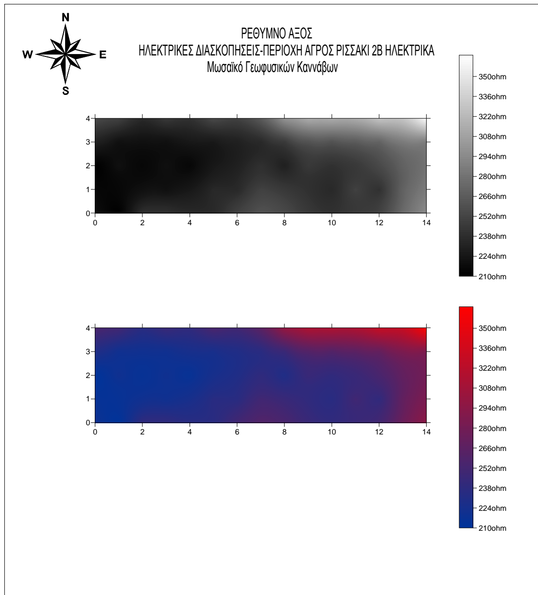
Σχήμα 4.3.3 περιοχή Αγρός Ρισσάκι 2B ηλεκτρικά χωρίς συμπίεση.
