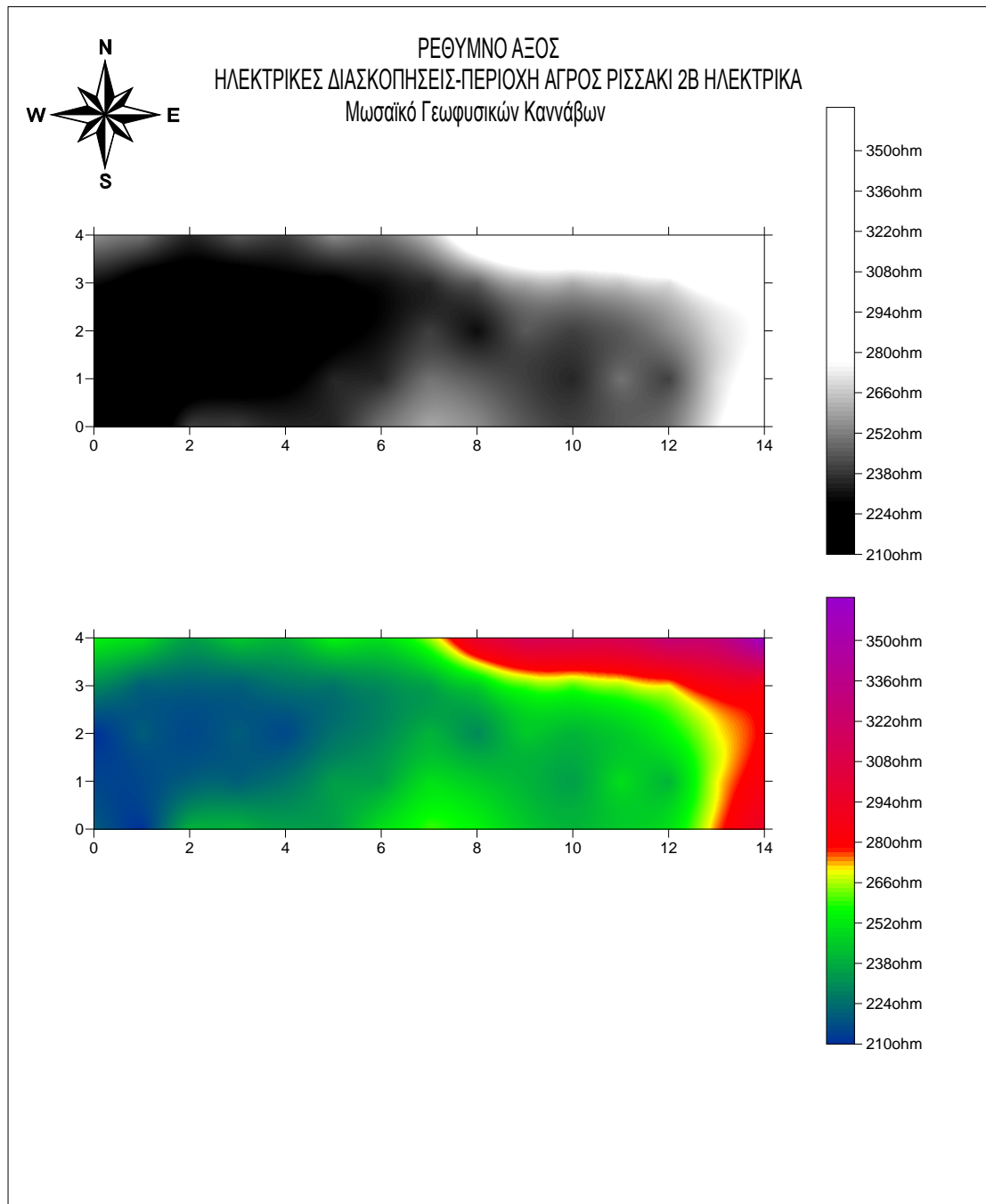
Σχήμα 4.3.4 περιοχή Αγρός Ρισσάκι 2B ηλεκτρικά με συμπίεση.
