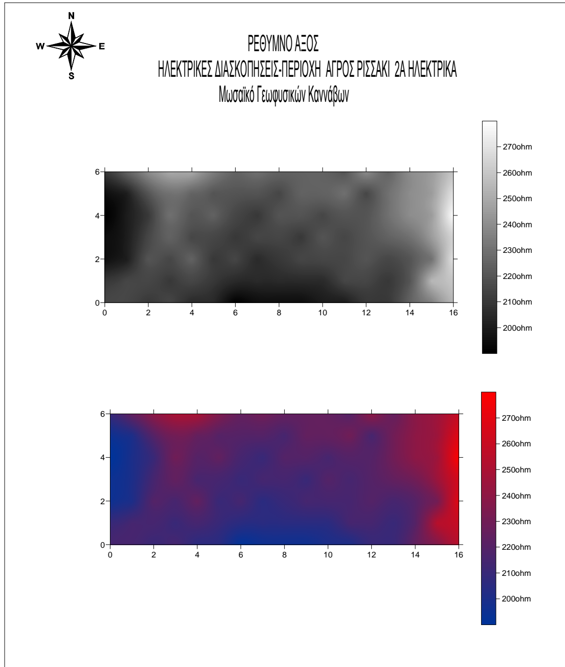
Σχήμα 4.3.1 περιοχή Αγρός Ρισσάκι 2Α ηλεκτρικά χωρίς συμπίεση.
