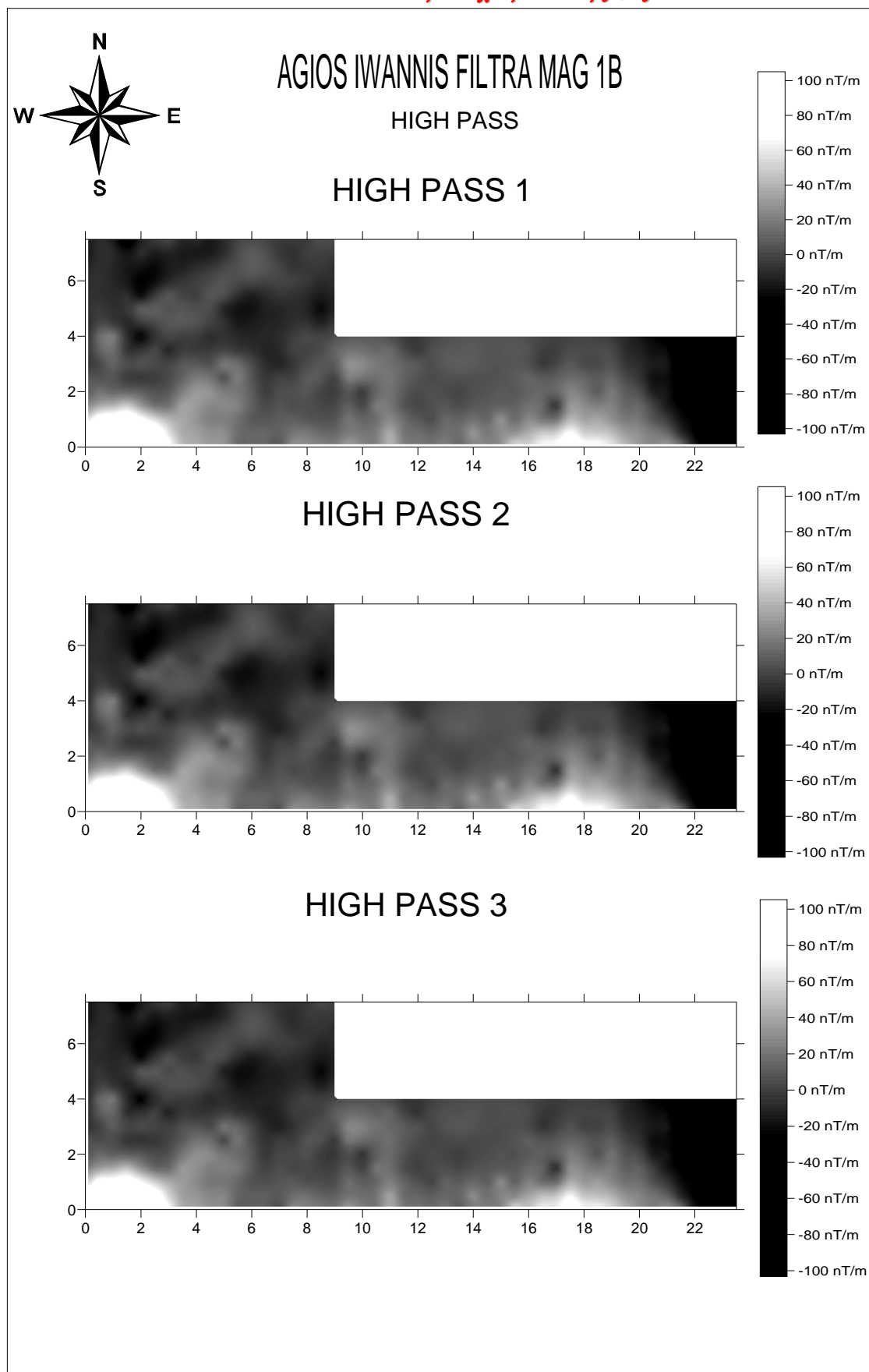
Σχήμα 4.1.5 φίλτρα high pass στον Άγιο Ιωάννη 1β.
