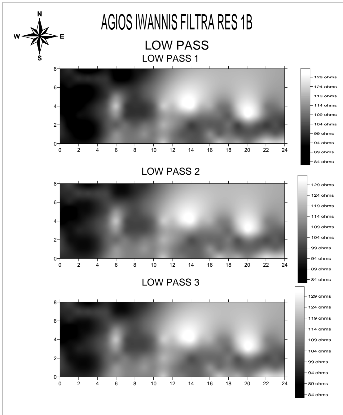
Σχήμα4.2.4 φίλτρα low pass Άγιος Ιωάννης 1β-ηλεκτρικά.
