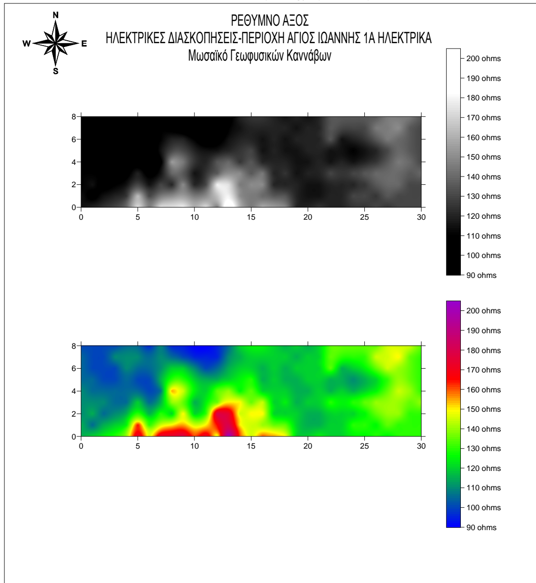
Σχήμα 4.1.3 περιοχή Άγιος Ιωάννης 1α ηλεκτρικά με συμπίεση.
