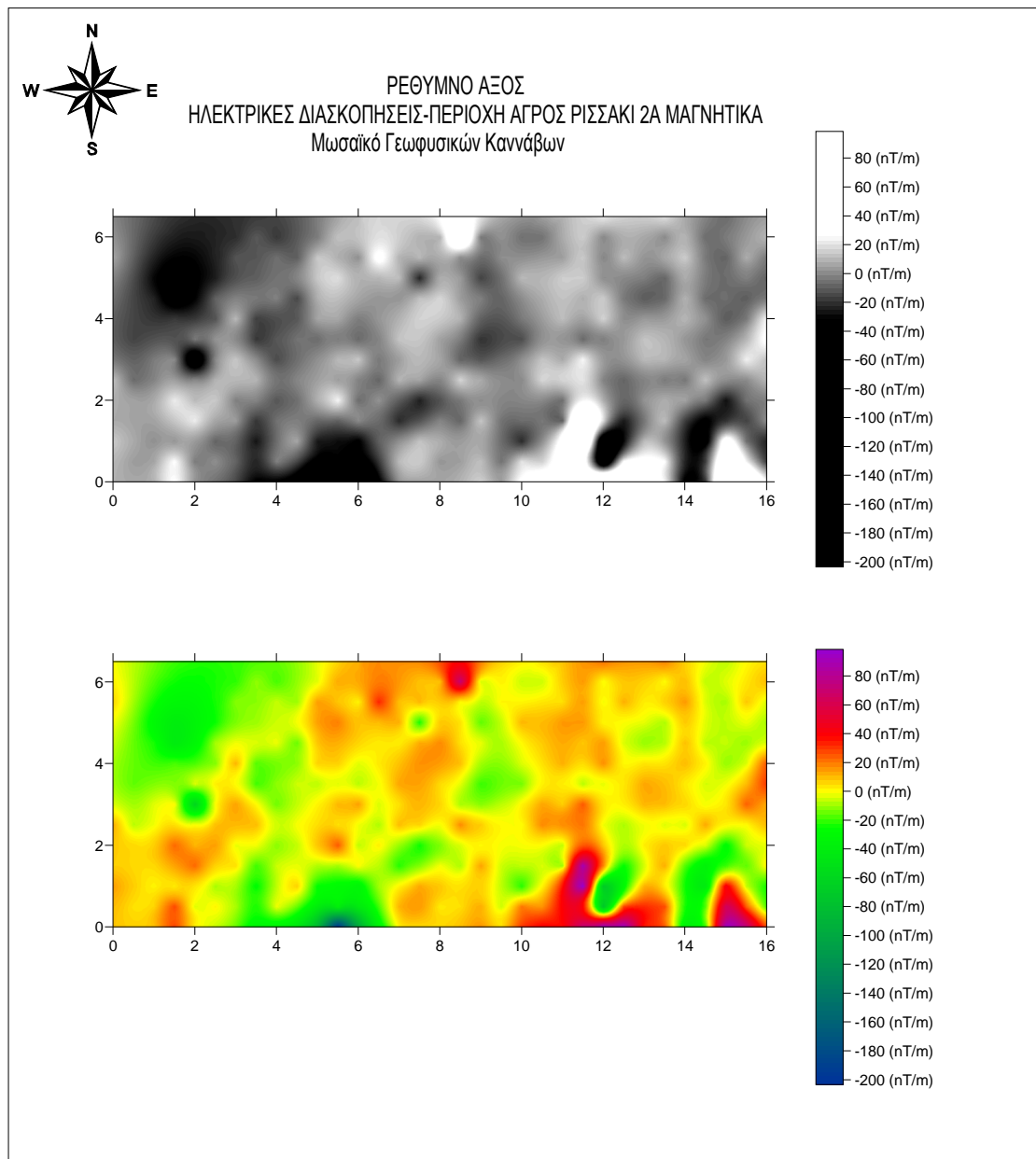
Σχήμα 4.4 περιοχή Αγρός Ρισσάκι 2Α μαγνητικά με συμπίεση.
