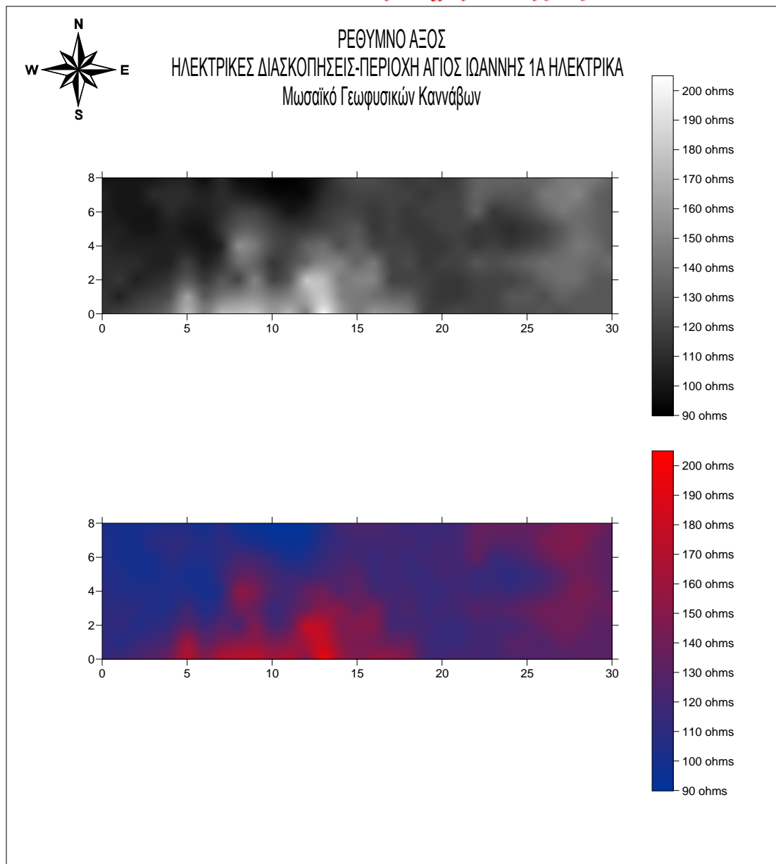
Σχήμα 4.1.2 περιοχή Άγιος Ιωάννης 1α ηλεκτρικά χωρίς συμπίεση.
