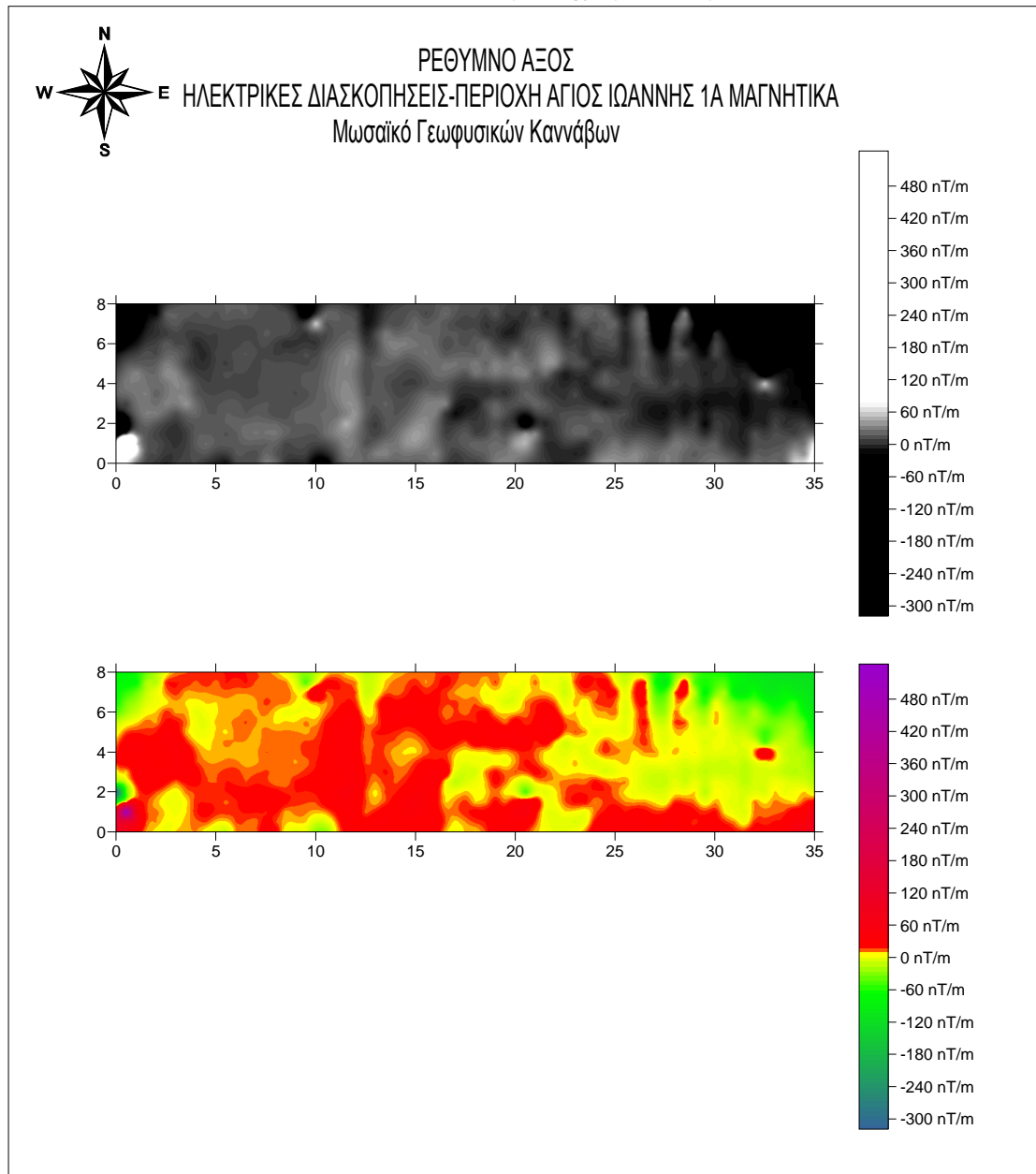
Σχήμα 4.1.1 περιοχή Άγιος Ιωάννης 1α μαγνητικά με συμπίεση
