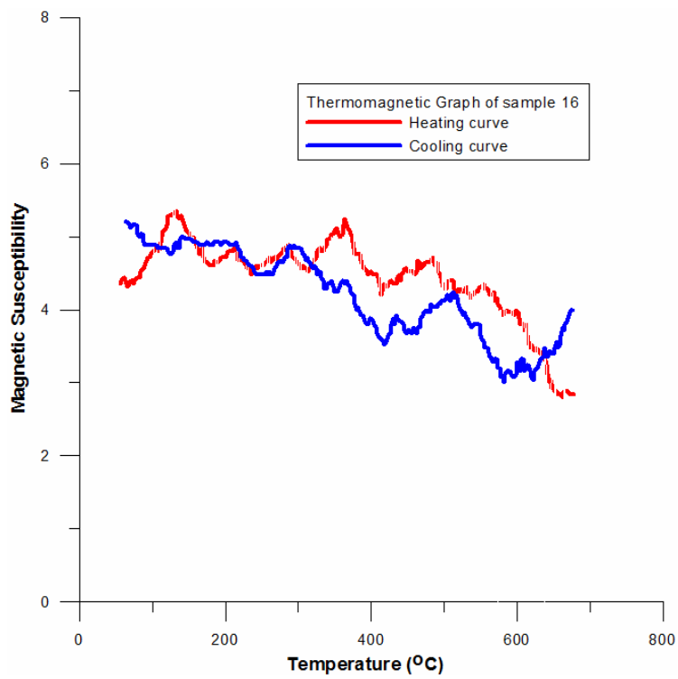
Σχήμα 4.20 θερμομαγνητική απόκριση για το δείγμα 16
