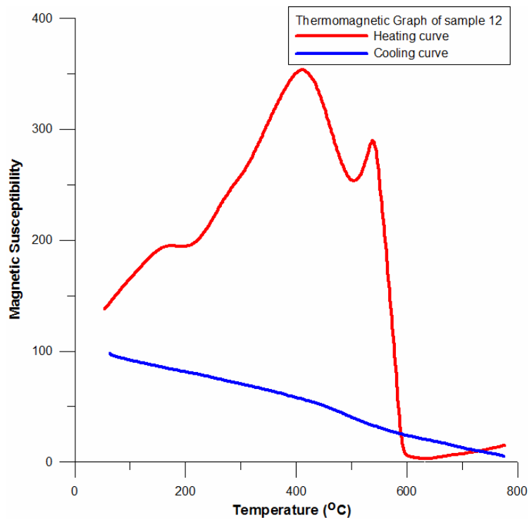
Σχήμα 4.16 θερμομαγνητική απόκριση για το δείγμα 12
