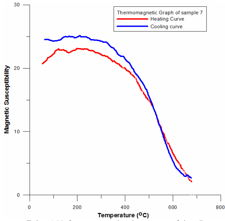
Σχήμα 4.11 θερμομαγνητική απόκριση για το δείγμα 7
