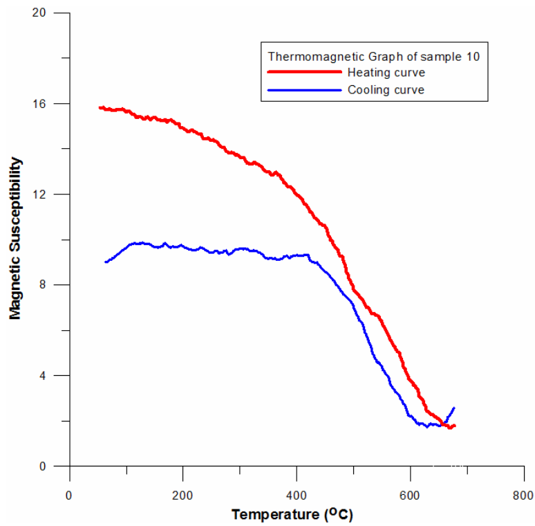
Σχήμα 4.14 θερμομαγνητική απόκριση για το δείγμα 10
