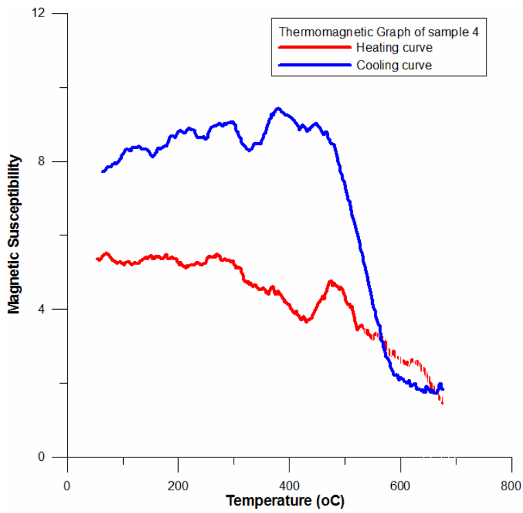
Σχήμα 4.8 θερμομαγνητική απόκριση για το δείγμα 4
