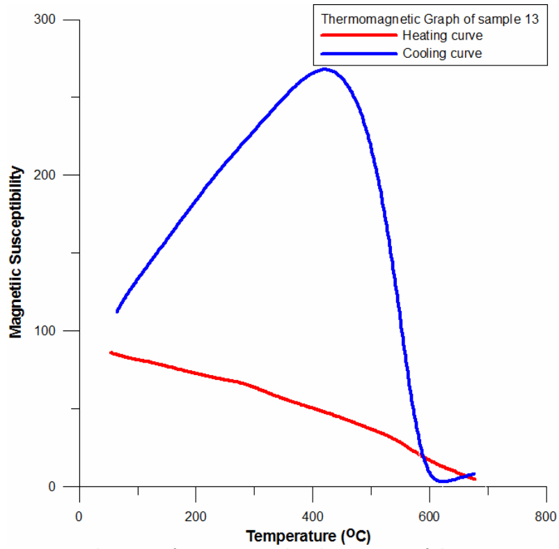
Σχήμα 4.17 θερμομαγνητική απόκριση για το δείγμα 13
