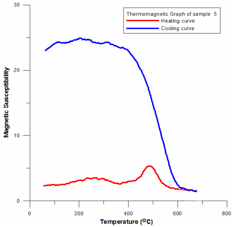
Σχήμα 4.9 θερμομαγνητική απόκριση για το δείγμα 5
