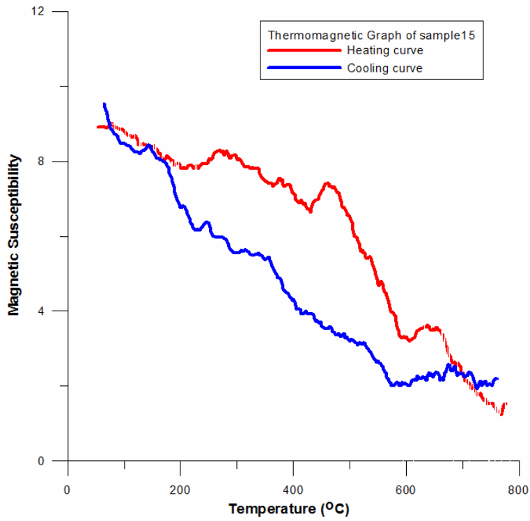
Σχήμα 4.19 θερμομαγνητική απόκριση για το δείγμα 15
