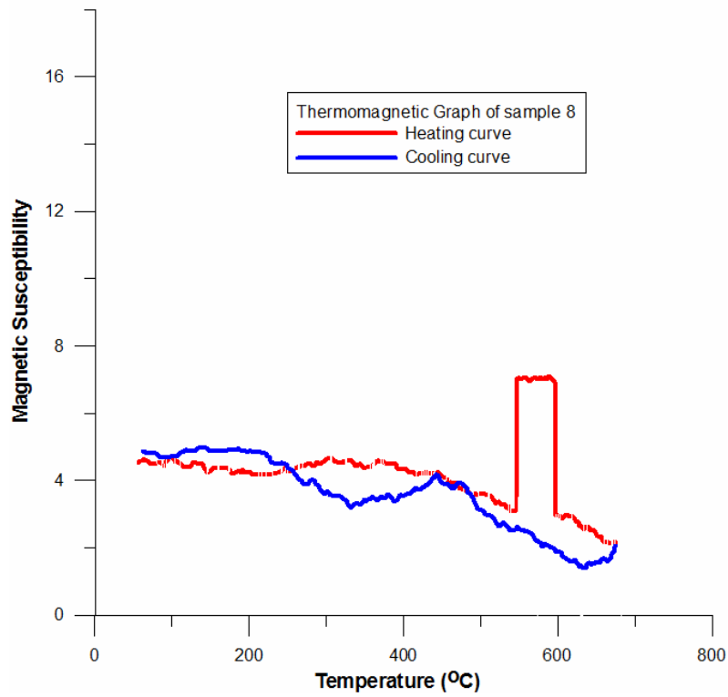
Σχήμα 4.12 θερμομαγνητική απόκριση για το δείγμα 8
