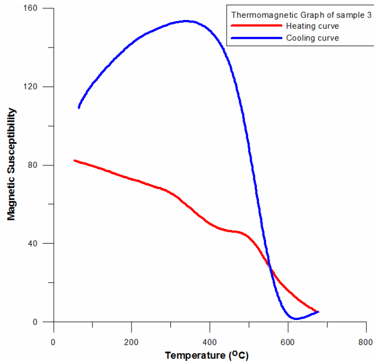
Σχήμα 4.7 θερμομαγνητική απόκριση για το δείγμα 3
