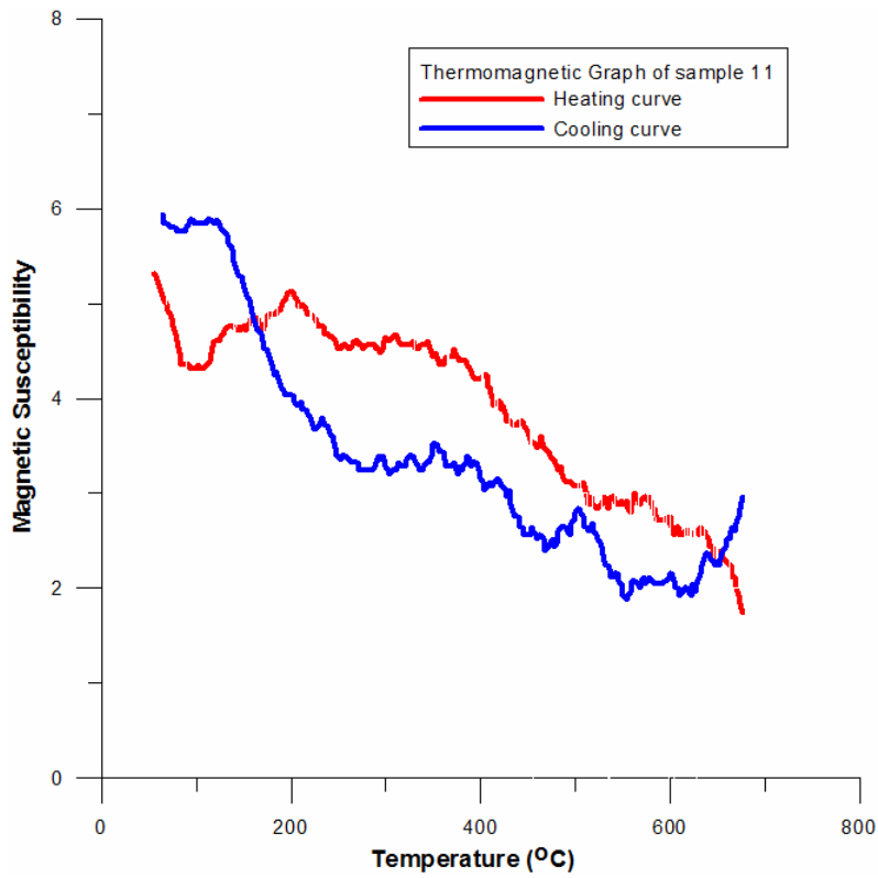
Σχήμα 4.15 θερμομαγνητική απόκριση για το δείγμα 11
