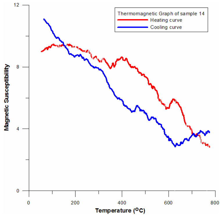
Σχήμα 4.18 θερμομαγνητική απόκριση για το δείγμα 14
