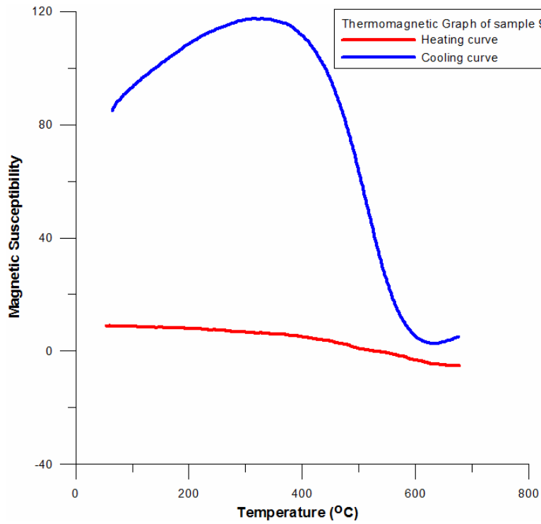
Σχήμα 4.13 θερμομαγνητική απόκριση για το δείγμα 9
