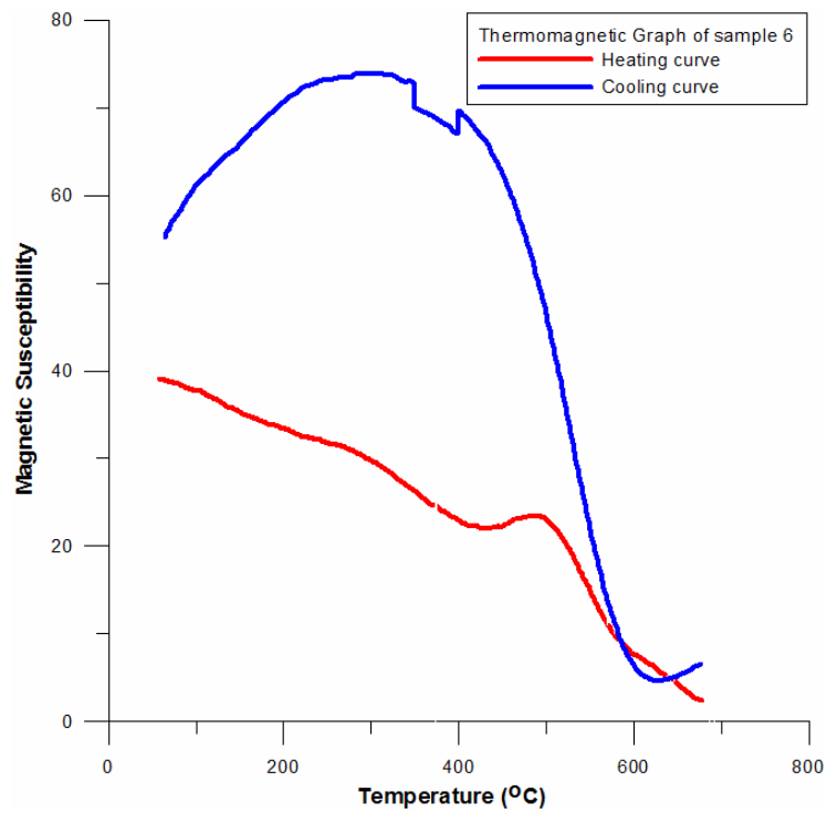
Σχήμα 4.10 θερμομαγνητική απόκριση για το δείγμα 6
