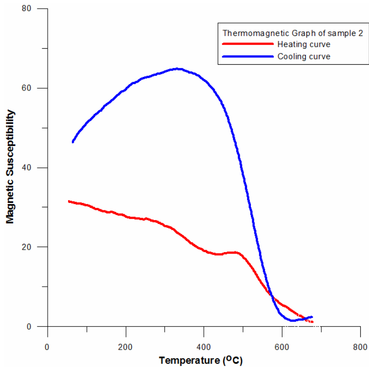
Σχήμα 4.6 θερμομαγνητική απόκριση για το δείγμα 2
