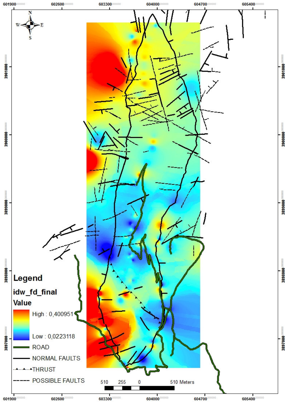
Σχήμα 4.4 Απεικόνιση της κατανομής της εξαρτώμενης από την συχνότητα μαγνητικής επιδεκτικότητας
