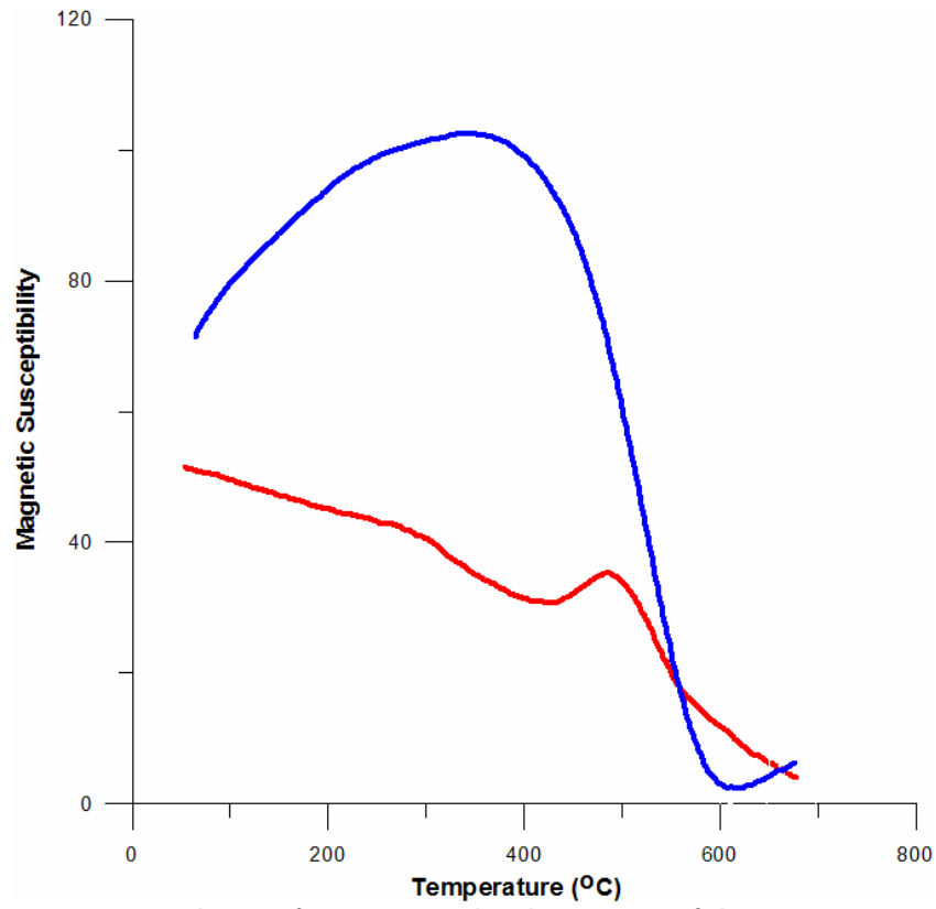
Σχήμα 4.5 θερμομαγνητική απόκριση για το δείγμα 1
