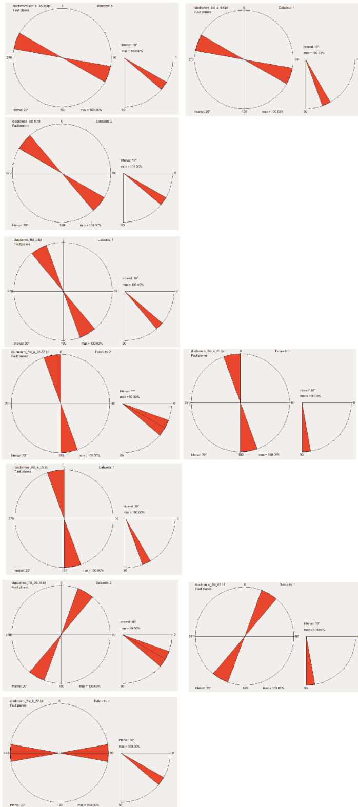
Σχήμα 3.9. Ταξινόμηση (σύμφωνα με την παράταξη και την κλίση) των κανονικών ρηγμάτων για την
