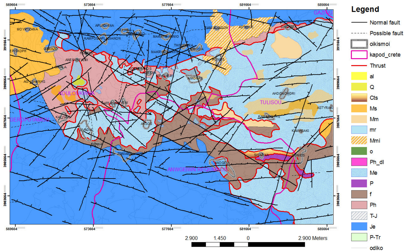
Σχήμα 2.2 Γεωλογικός χάρτης της περιοχής μελέτης
