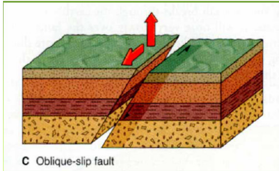
Σχήμα 3.5. Πλάγια ρήγματα.
