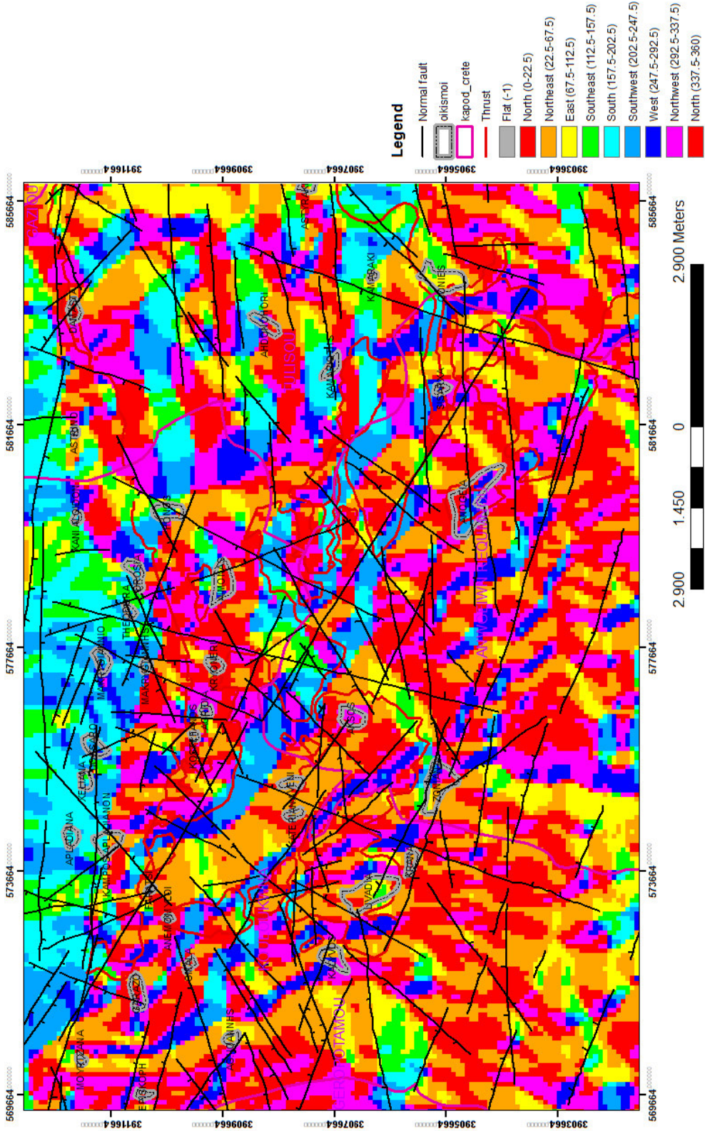
Σχήμα 3.3. Χάρτης που απεικονίζει τις επικρατούσες διευθύνσεις των τοπογραφικών στοιχείων της περιοχής μελέτης σε συνδυασμό με της τεκτονική χαρτογράφηση
