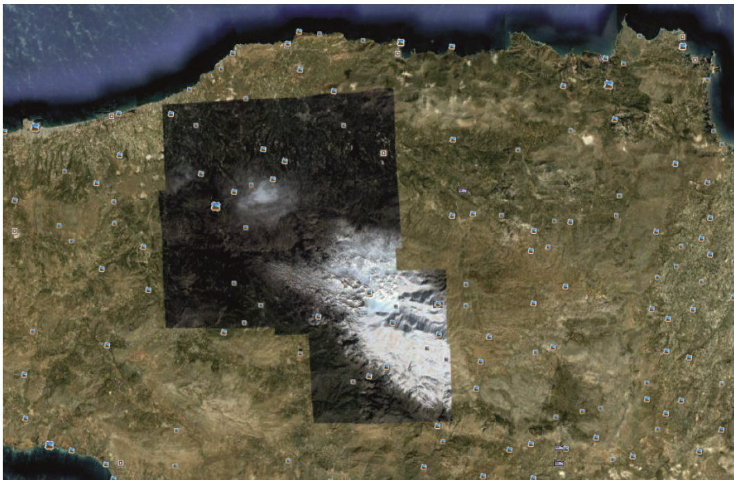
Σχήμα 1.1 Εικόνα της ευρύτερης περιοχής του Ψηλορείτη (από google earth)
