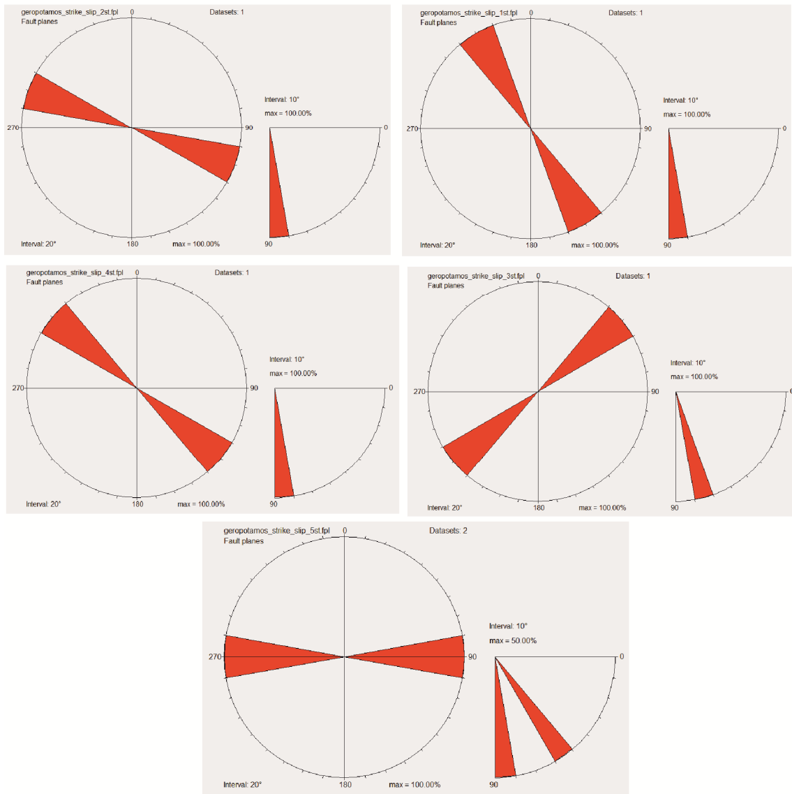
Σχήμα 3.6. Ταξινόμηση (σύμφωνα με την παράταξη και την κλίση) των strike-slip ρηγμάτων για την περιοχή του Γεροπόταμου
