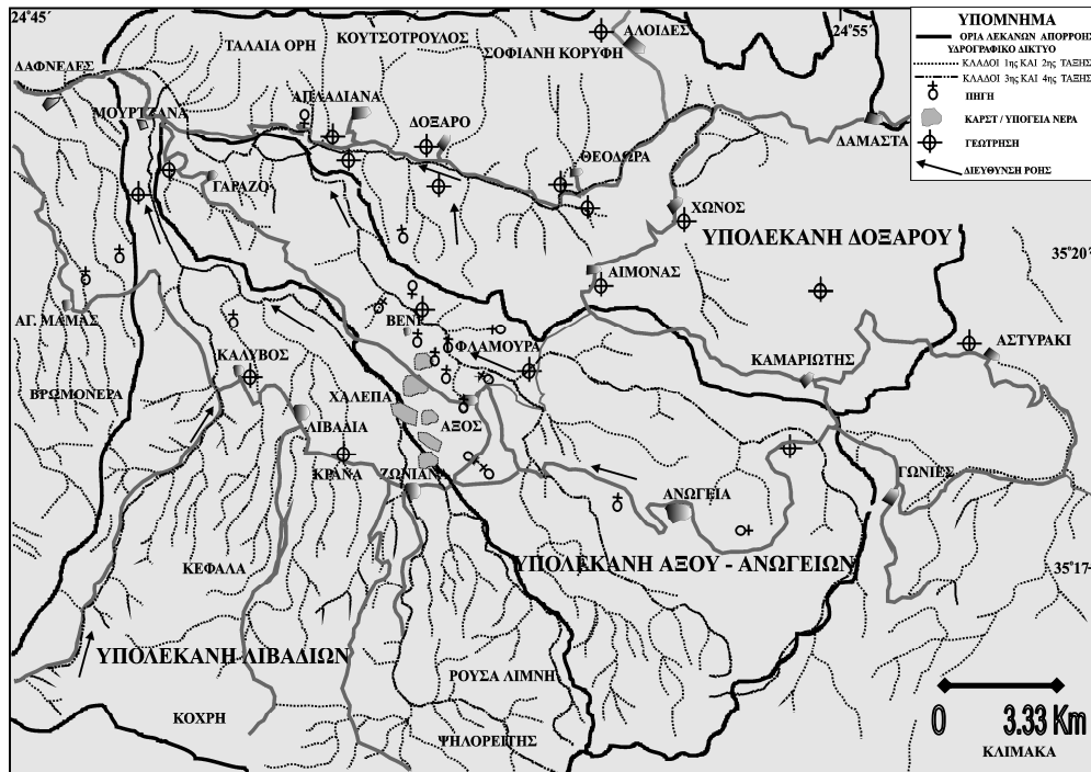
Σχήμα 2.3 Υδρογραφικό δίκτυο της περιοχής μελέτης (αρίθμηση κατά Strahler)
