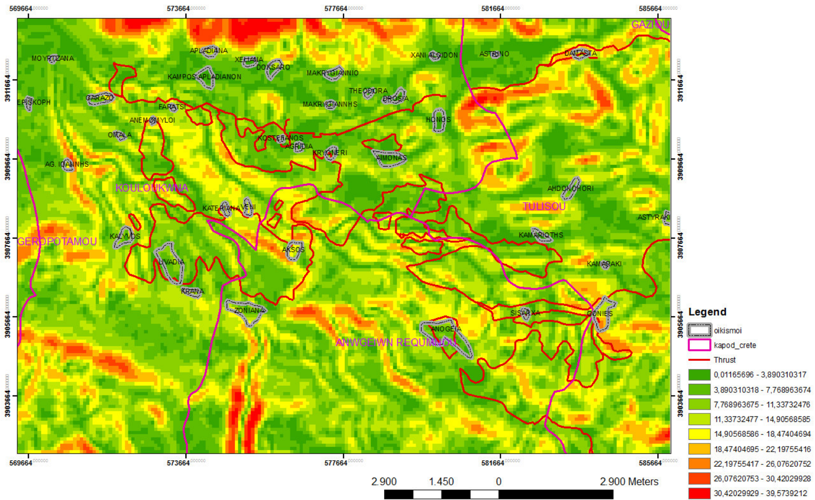
Σχήμα 2.1 Χάρτης κλίσεων της περιοχής μελέτης
