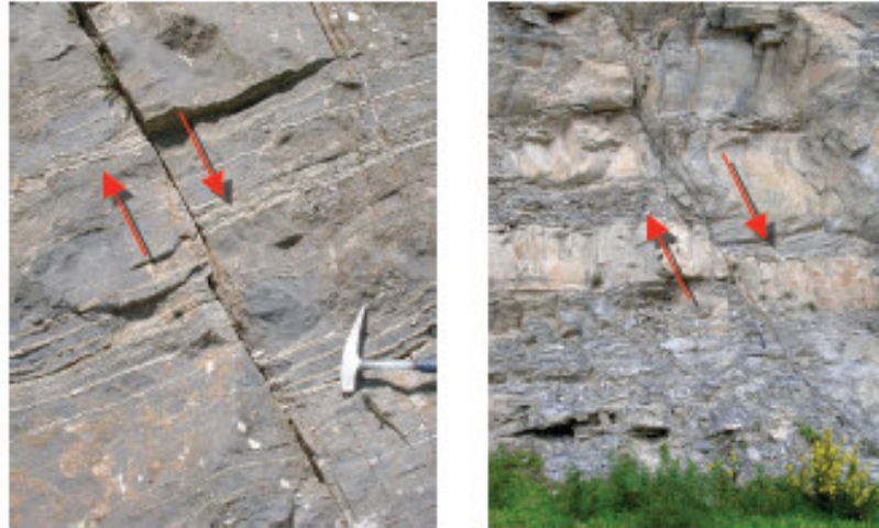
Σχήμα 3.3. Παραδείγματα κανονικών ρηγμάτων.
