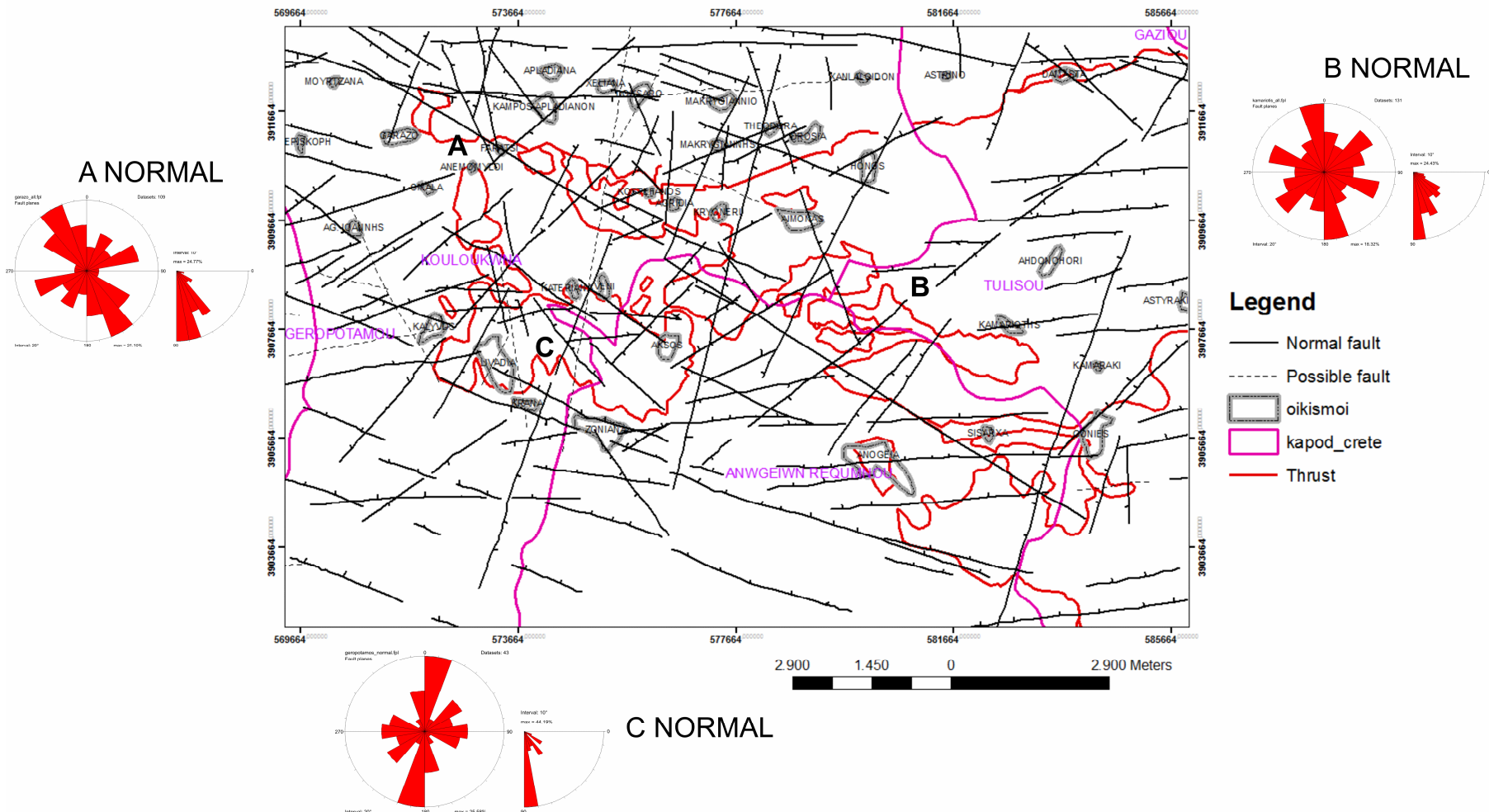
Σχήμα 3.3. Ροδοδιαγράμματα κατανομής των κανονικών ρηγμάτων στην περιοχή μελέτης
