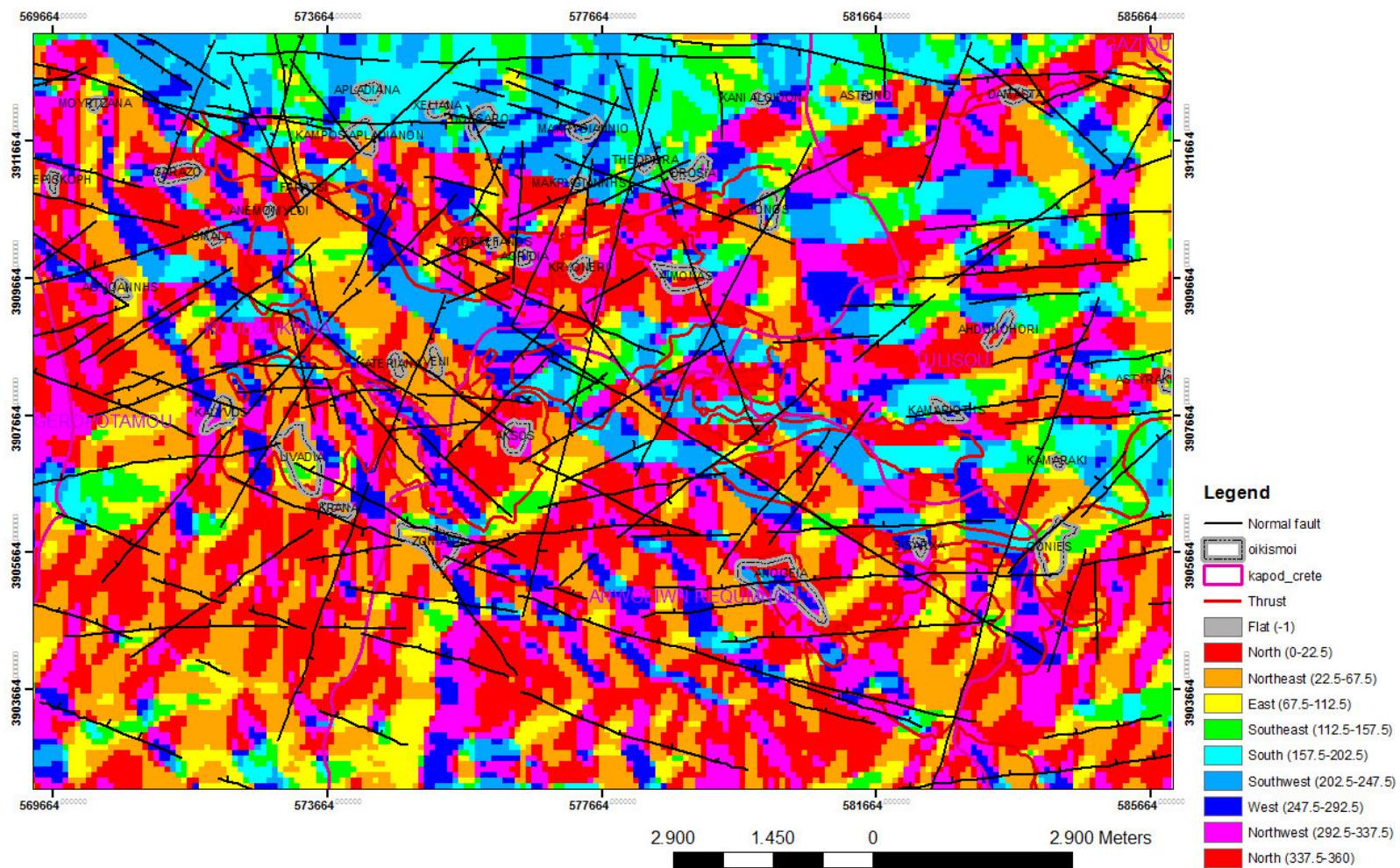
Σχήμα 3.4. Χάρτης που απεικονίζει τις επικρατούσες διευθύνσεις των τοπογραφικών στοιχείων της περιοχής μελέτης σε συνδυασμό με της τεκτονική χαρτογράφηση
