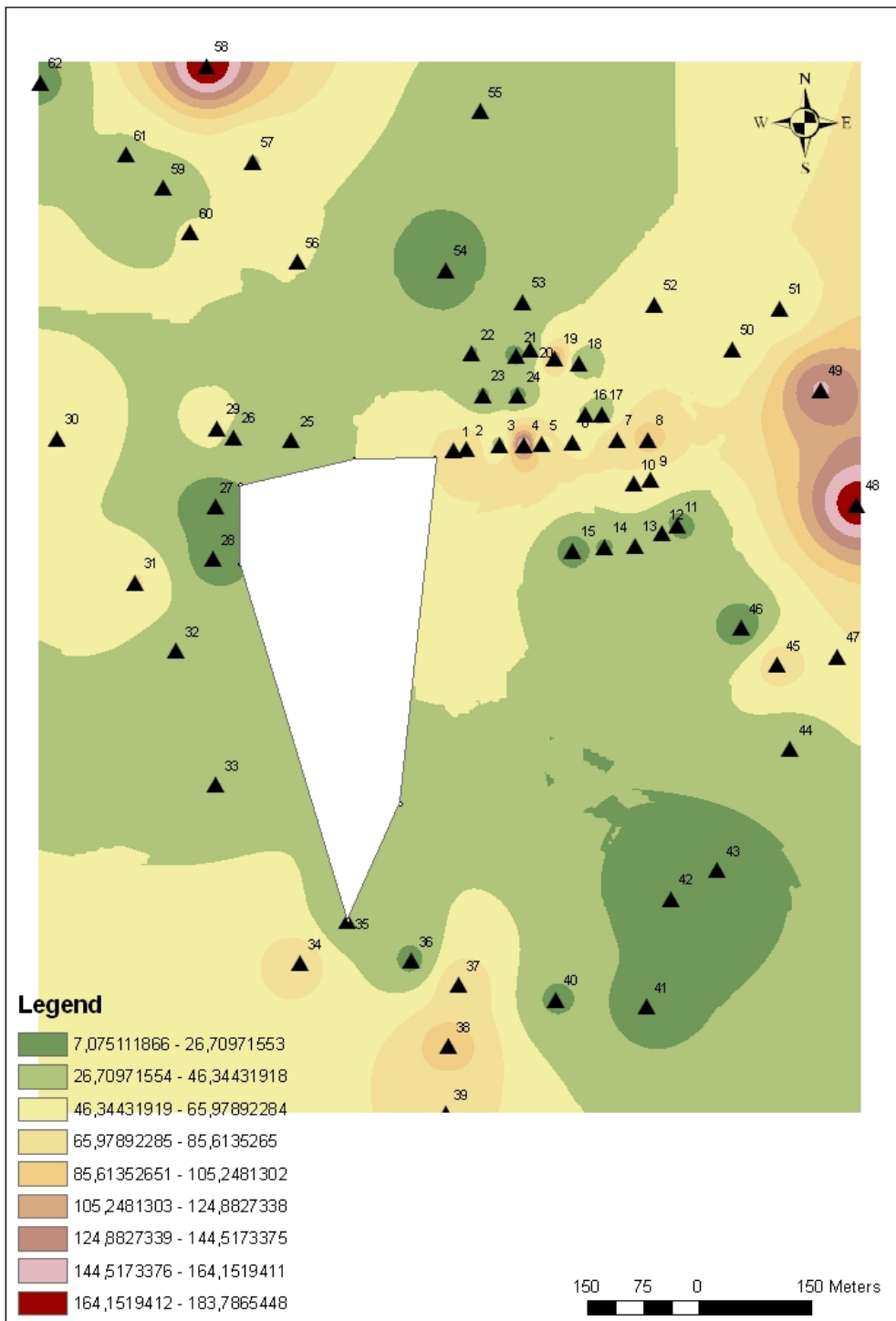
Σχήμα 4.3 Απεικόνιση της κατανομής της μαγνητικής επιδεκτικότητας (SI units) σε υψηλή συχνότητα με την μέθοδο παρεμβολής IDW, στον υποσταθμό της ΔΕΗ Χανίων.
