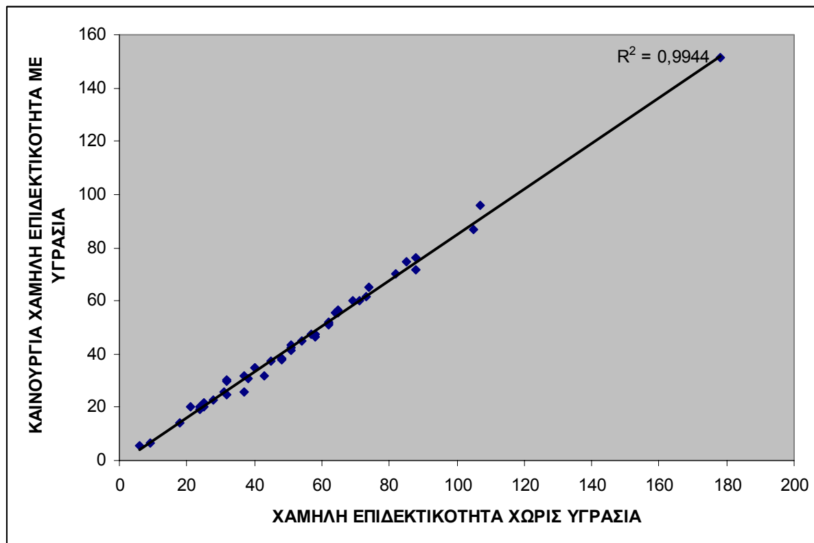
Σχήμα 4.9 Συσχετισμός παλιάς χαμηλής επιδεκτικότητας χωρίς υγρασία με την καινούργια χαμηλή επιδεκτικότητα με υγρασία (SI units).
