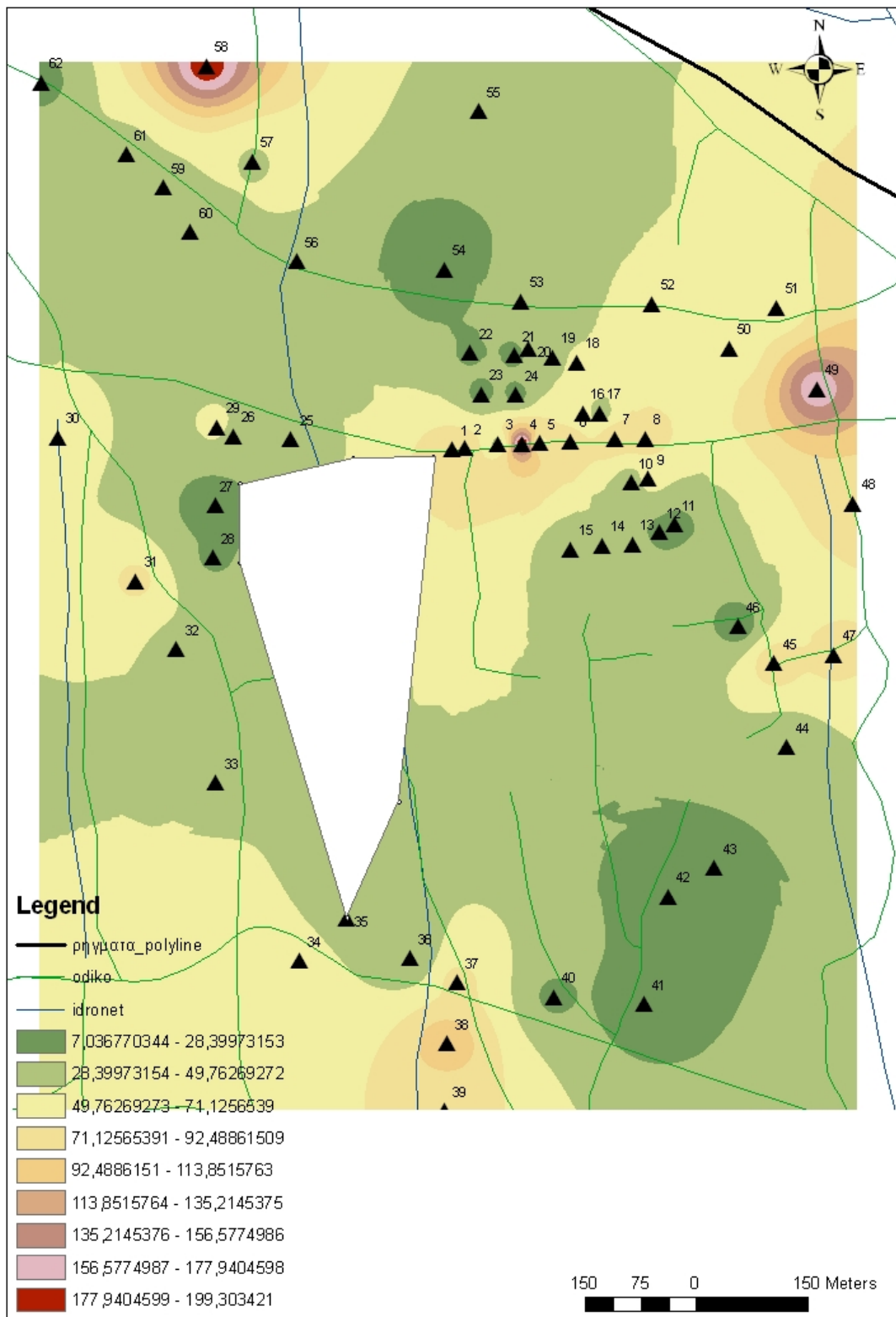
Σχήμα 4.10 Ερμηνεία της κατανομής της μαγνητικής επιδεκτικότητας (SI μονάδες) σε χαμηλή συχνότητα με την μέθοδο παρεμβολής IDW, στον υποσταθμό της ΔΕΗ Χανίων.
