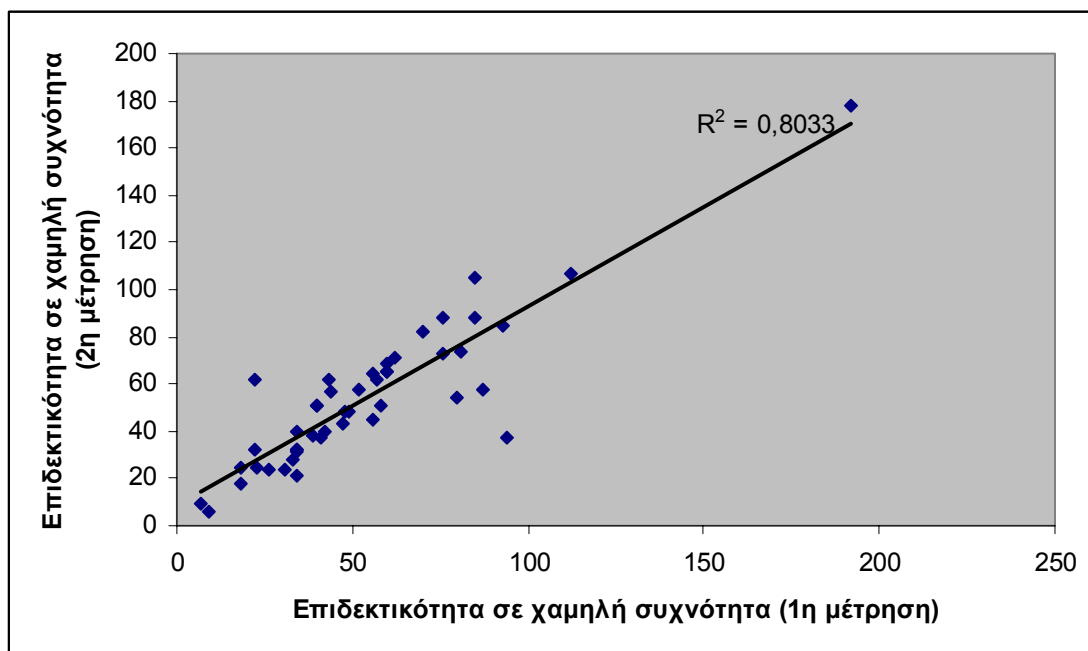
Σχήμα 4.5 Συσχετισμός μετρήσεων χαμηλής επιδεκτικότητας από τις δύο φάσεις μετρήσεων (SI units).
