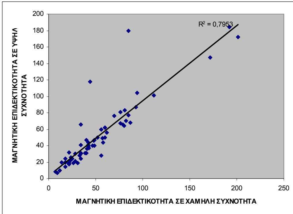
Σχήμα 4.4 Συσχετισμός χαμηλής και υψηλής επιδεκτικότητας (SI units).
