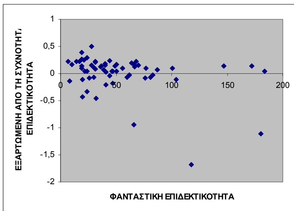
Σχήμα 4.8 Συσχετισμός φανταστικής επιδεκτικότητας με την εξαρτώμενη από τη συχνότητα επιδεκτικότητα (SI units).
