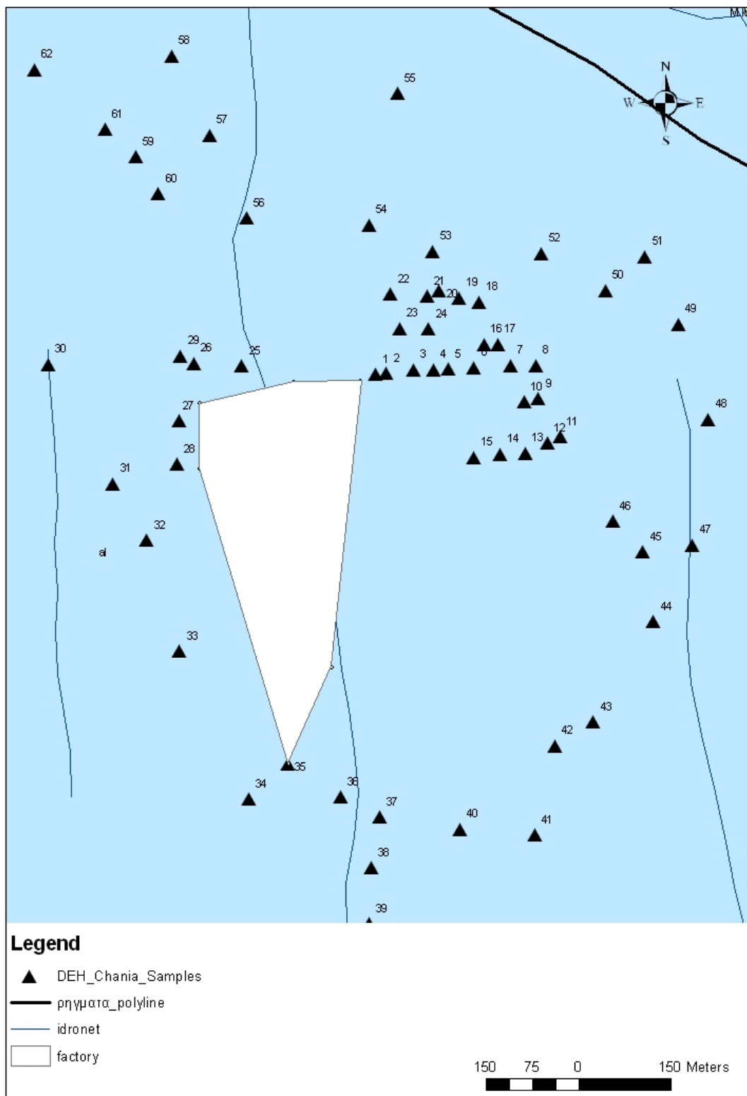
Σχήμα 2.2 Γεωλογία της εξεταζόμενης περιοχής.
