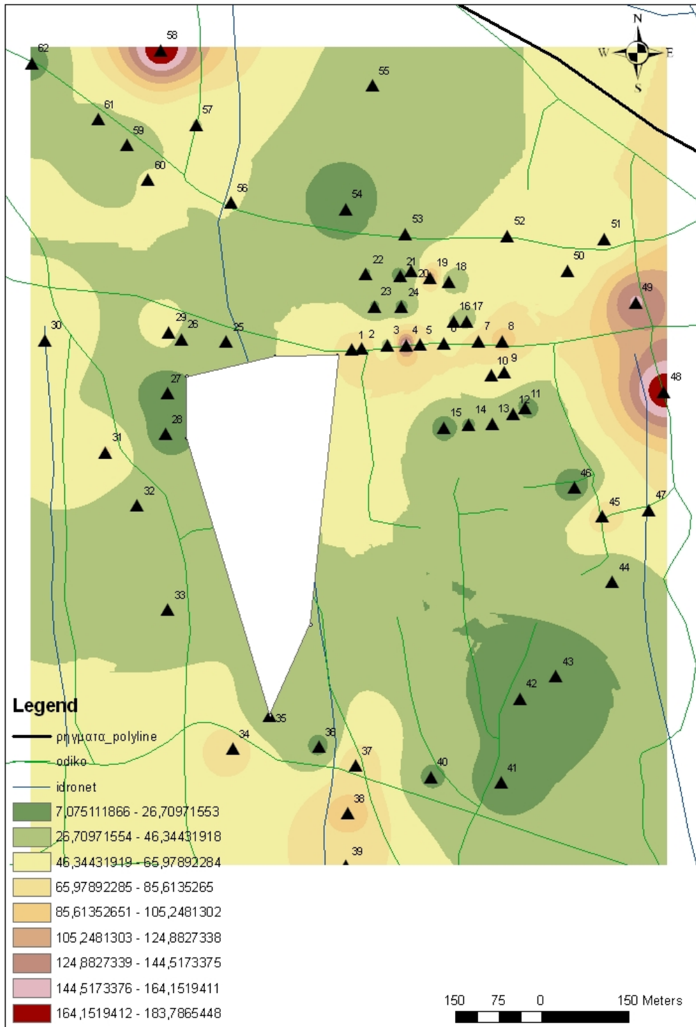
Σχήμα 4.11 Ερμηνεία της κατανομής της μαγνητικής επιδεκτικότητας ( m^3 Kg^{-1} ) σε υψηλή συχνότητα με την μέθοδο παρεμβολής IDW, στον υποσταθμό της ΔΕΗ Χανίων.
