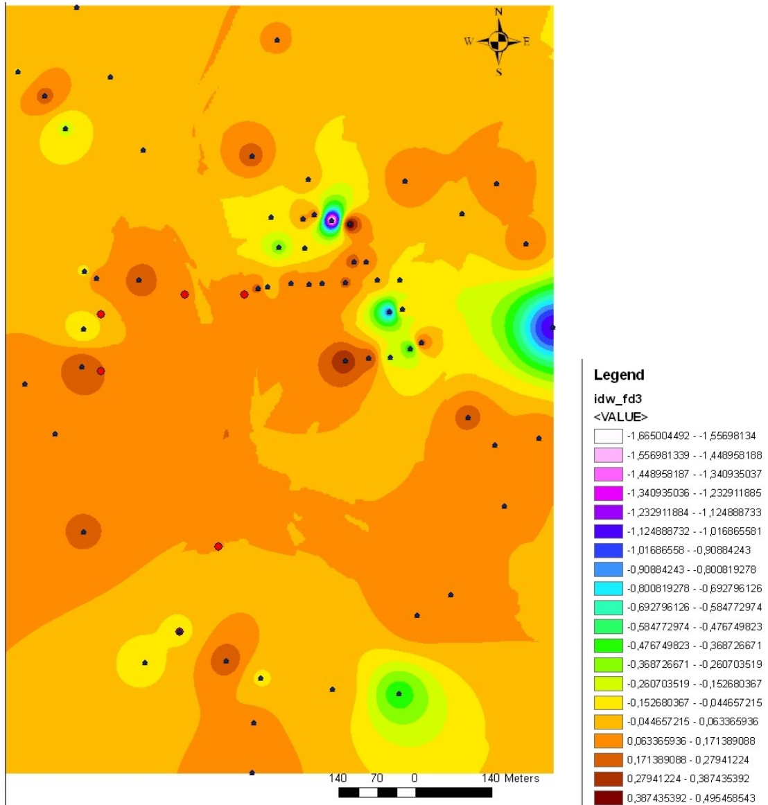
Σχήμα 4.6 Απεικόνιση της κατανομής της μαγνητικής επιδεκτικότητας η οποία εξαρτάται από την συχνότητα.
