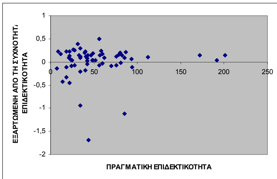
Σχήμα 4.7 Συσχετισμός πραγματικής επιδεκτικότητας με την εξαρτώμενη από τη συχνότητα επιδεκτικότητα (SI units).
