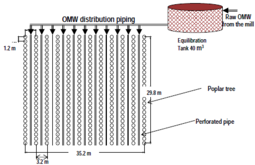
Απεικόνιση της τεχνολογίας υπεδάφιας διάθεσης υγρών αποβλήτων ελαιοτριβείου σε συνδυασμό με φυτοεξυγίανση - Ελαιοτριβείο ΚΟΚΟΛΗΣ (ΧΑΝΙΑ-ΒΑΣΙΛΑΚΗ)
