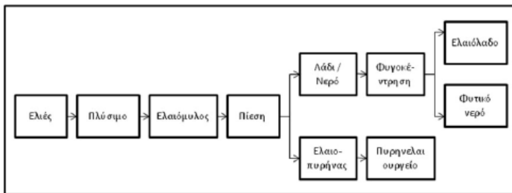
Διάγραμμα ροής του παραδοσιακού συστήματος παραγωγής ελαιόλαδου
