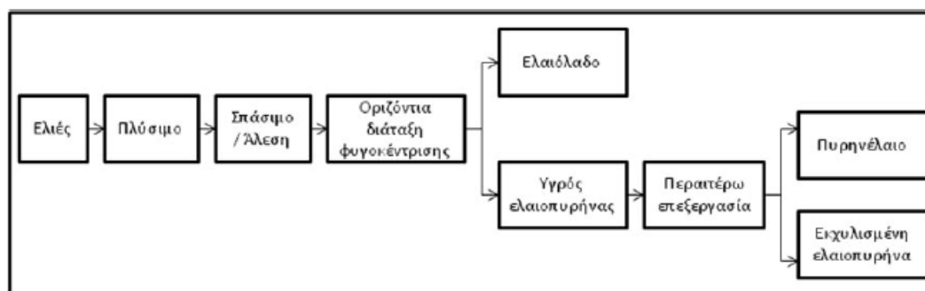
Διάγραμμα ροής του διφασικού συστήματος παραγωγής ελαιολάδου
