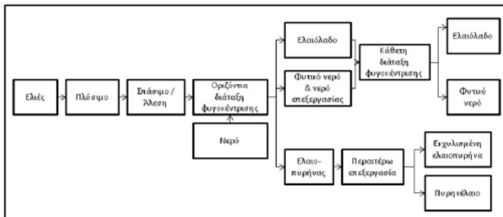
Διάγραμμα ροής του τριφασικού συστήματος παραγωγής ελαιολάδου
