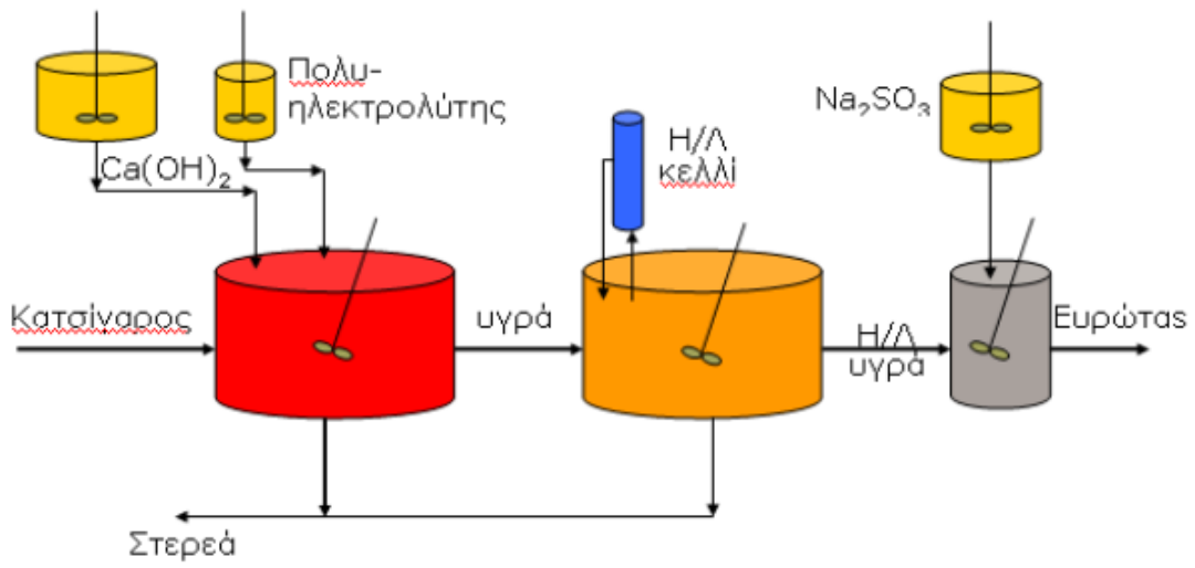
Σχηματική διάταξη μονάδας ηλεκτρόλυσης του κατσίγαρου.
