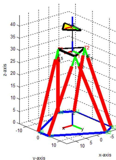
Εικόνα 5.2.1.: απεικόνιση θέση μέγιστης ευελιξίας της πλατφόρμας “Stewart” (εικονική - πραγματική)
