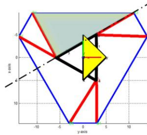
Εικόνα 5.1.2.2.: παραλληλισμός της πλευράς της άνω βάσης ( T_1 T_2 ) με το επίπεδο του τριγώνου ( T_2 B_3 B_4 )
