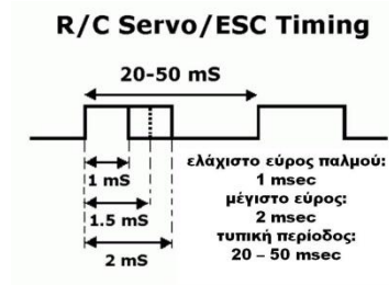
Εικόνα 3.3.2.1. εύρος παλμού του σήματος ελέγχου
