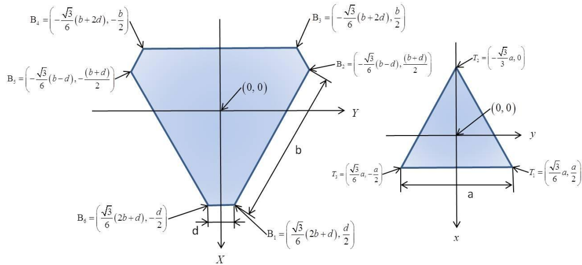
Σχήμα 2.1.2.: Η βάση είναι ένα ημικανονικό εξαγώνο με μήκη πλευρών b, d και η άνω βάση ένα ισόπλευρο τρίγωνο πλευράς a
