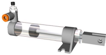
Εικόνα 1.5.3.: πνευματικός επενεργητής
