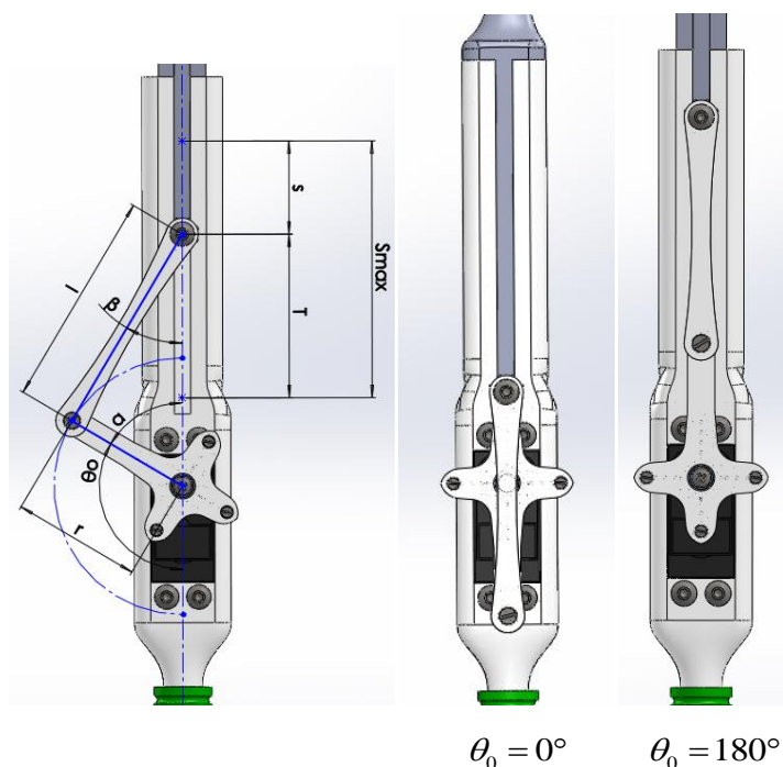
Εικόνα 3.3.1.: κατασκευασμένη πρισματική άρθρωση
