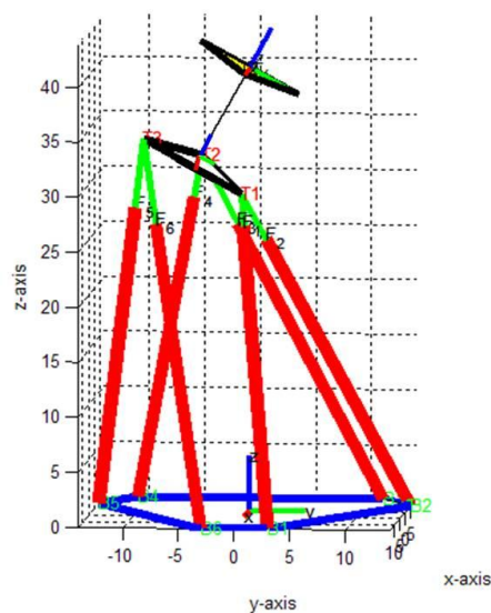
Εικόνα 5.2.4.2.: μέγιστη περιστροφή γύρω από τον άξονα των X του πλαισίου συντεταγμένων της κάτω βάσης της πλατφόρμας κατά γωνία \alpha^\circ < 0
