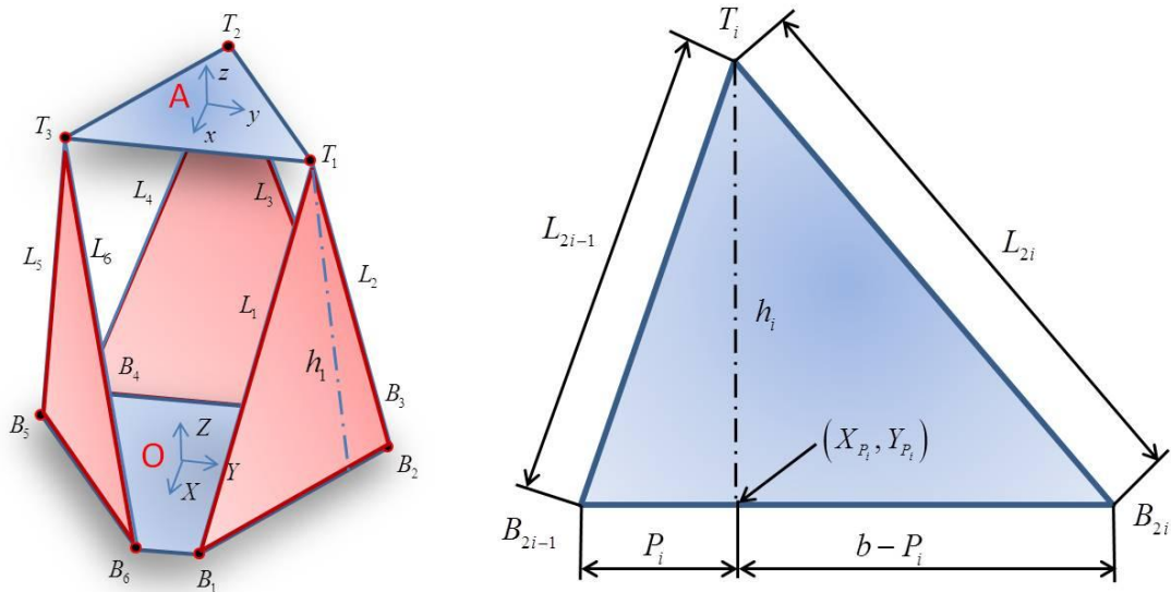
Σχήμα 2.1.6.: ύψος τριγώνων
