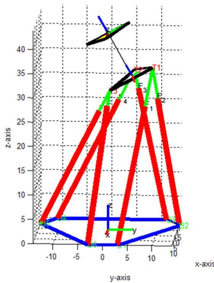
Εικόνα 5.2.4.1.: μέγιστη περιστροφή γύρω από τον άξονα των X του πλαισίου συντεταγμένων της κάτω βάσης της πλατφόρμας κατά γωνία \alpha^\circ > 0
