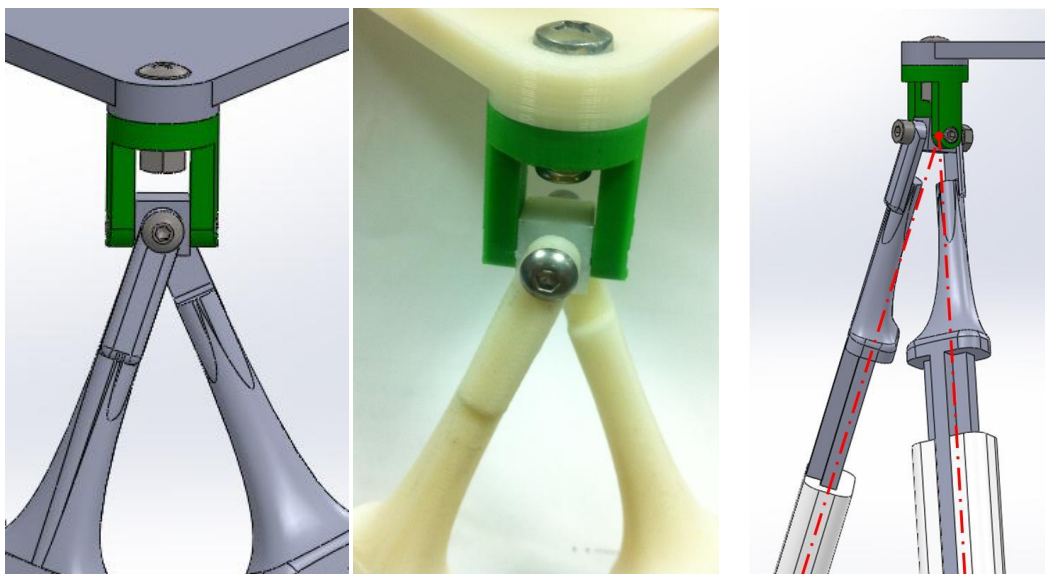
Εικόνα 3.1.2.5.1.: άρθρωση άνω βάσης (σχεδιασμένη - κατασκευασμένη)
