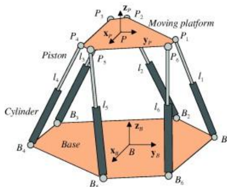
Εικόνα 1.2.1.: πλατφόρμα “Stewart”
