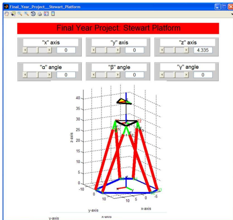
Εικόνα 4.5.3.2.1: απεικόνιση της εφαρμογής ελέγχου της πλατφόρμας "Stewart"
