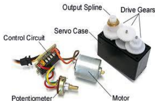
Εικόνα 4.2.1.1. εσωτερικό σερβοκινητήρα
