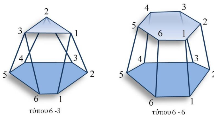
Σχήμα 1.2.4.: τύποι πλατφόρμας "Stewart"
