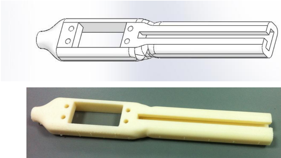
Εικόνα 3.1.2.3.1.1.: σταθερός σύνδεσμος πρισματικής άρθρωσης (σχεδιασμένος – κατασκευασμένος)
