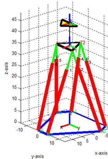
Εικόνα 5.1.3.2.: μέγιστη θέση της πλατφόρμας
