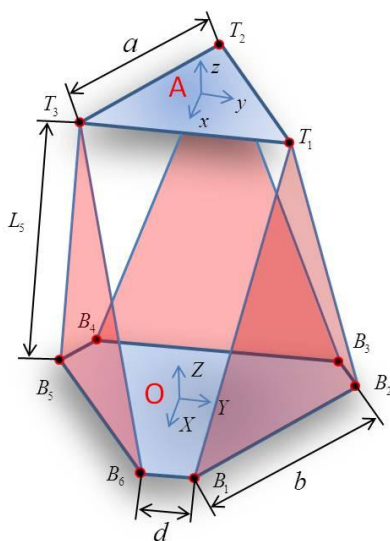
Σχήμα 5.1.3.1.: διαστάσεις πλατφόρμας
