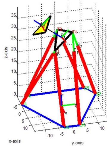
Εικόνα 5.1.3.7.: περιστροφή γύρω από τον άξονα των X
