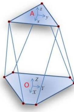
Σχήμα 2.1.1.: Η γεωμετρία της πλατφόρμας “Stewart”
