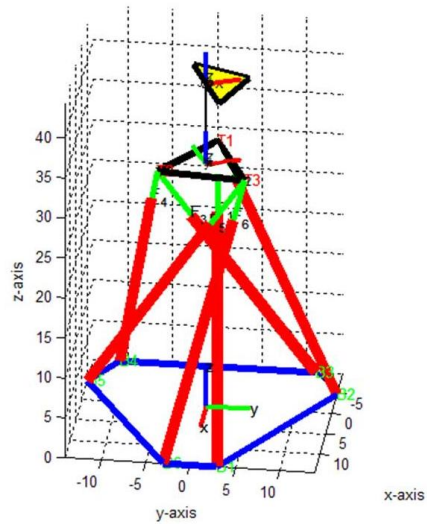
Εικόνα 5.1.3.9.: περιστροφή γύρω από τον άξονα των z
