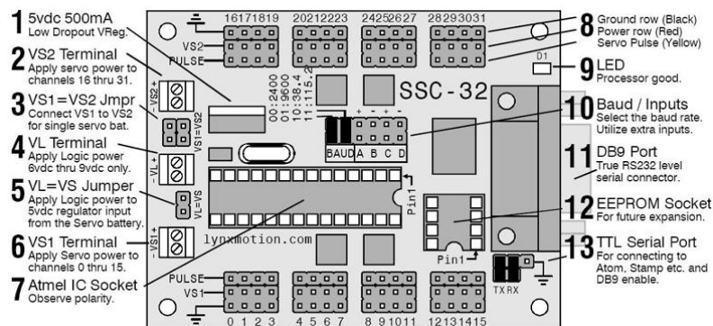
Εικόνα 4.4.1.1. μέρη πλακέτας ssc - 32
