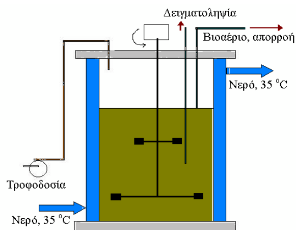
Σχήμα 7.1: Πειραματική διάταξη αντιδραστήρα συνεχούς λειτουργίας (CSTR) για την παραγωγή μεθανίου.
