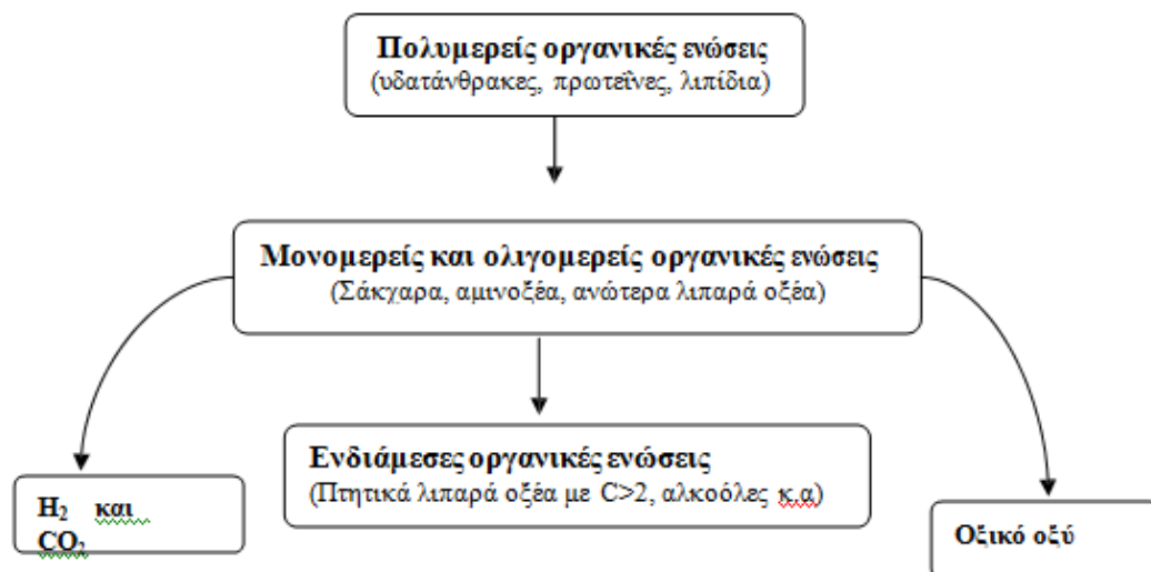
Σχήμα 4.2: Η διεργασία της αναερόβιας χώνευσης για την παραγωγή υδρογόνου από οργανική ύλη.
