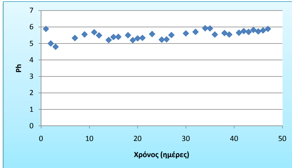
Διάγραμμα 8.2: Μεταβολή του pH κατά την διάρκεια λειτουργίας των αντιδραστήρων.
