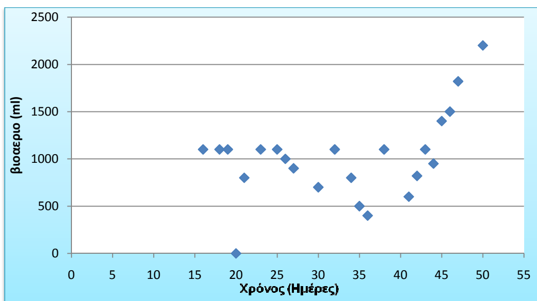
Διάγραμμα 8.1: Μεταβολή του ρυθμού παραγωγής βιοαερίου κατά την διάρκεια λειτουργίας του αντιδραστήρα.
