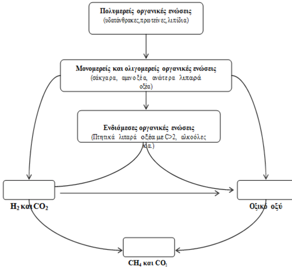
Σχήμα 4.1: Η διεργασία της αναερόβιας χώνευσης για την παραγωγή βιοαερίου από οργανική ύλη
