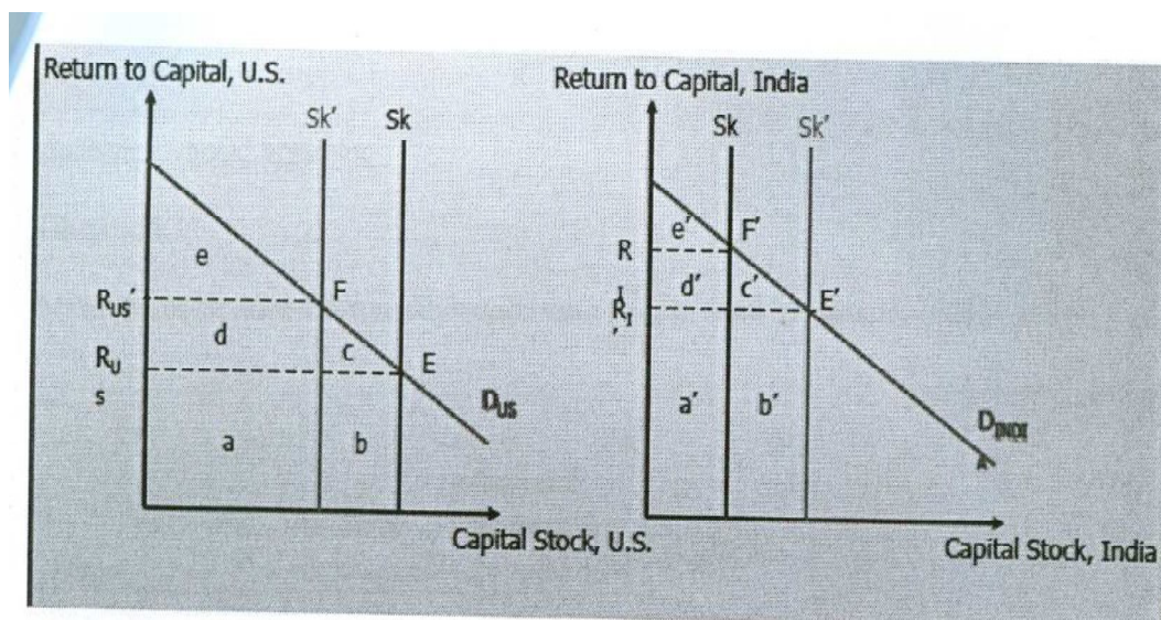
ΔΙΑΓΡΑΜΜΑ 4 : Οι συνέπειες της ευημερίας και της εκροής στη διεθνή κινητικότητα κεφαλαίου.
