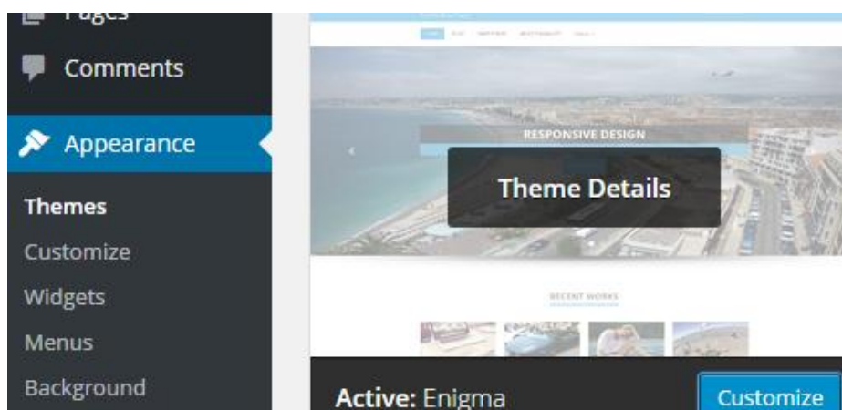
Εικόνα 25. Επιλογή θέματος
