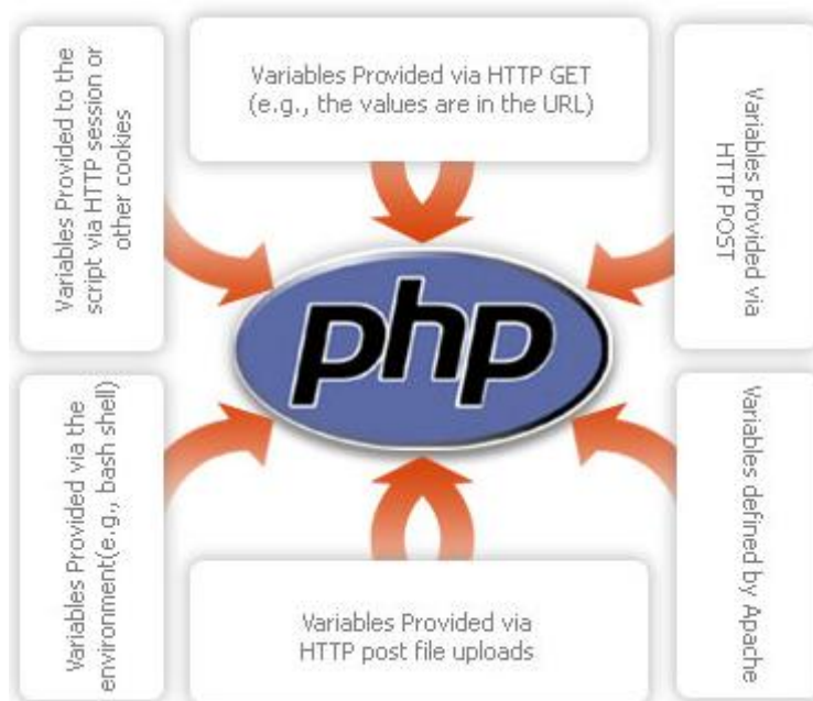
Εικόνα 9.PHP
