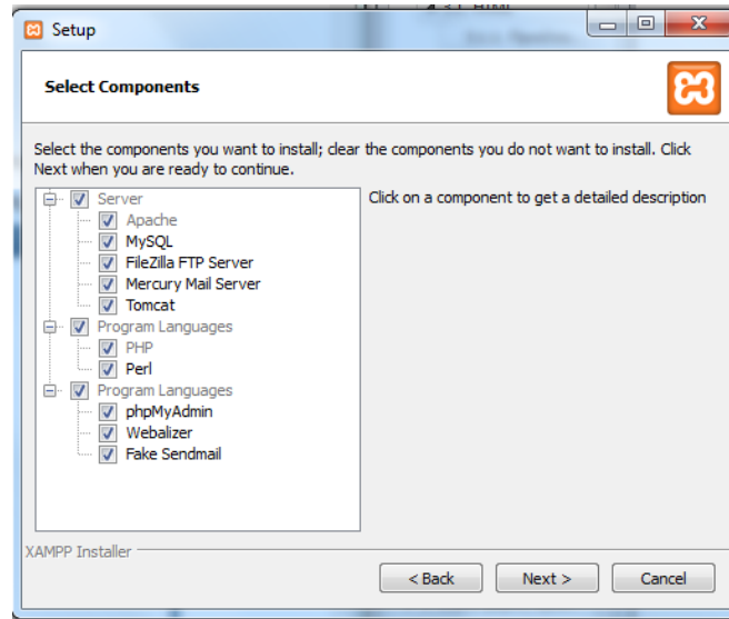
Εικόνα 13.Εγκατάσταση xampp-Βήμα 2
