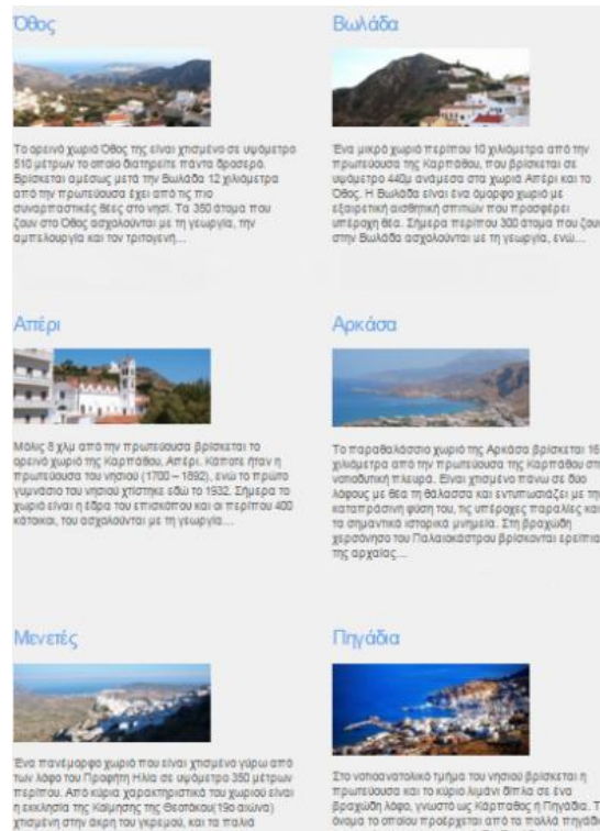
Εικόνα 27. Menu-Χωριά
