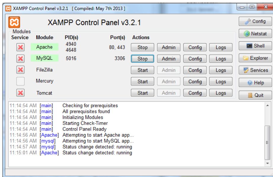
Εικόνα 16.Control Panel Xampp
