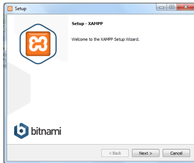
Εικόνα 12.Εγκατάσταση xampp-Βήμα 1
