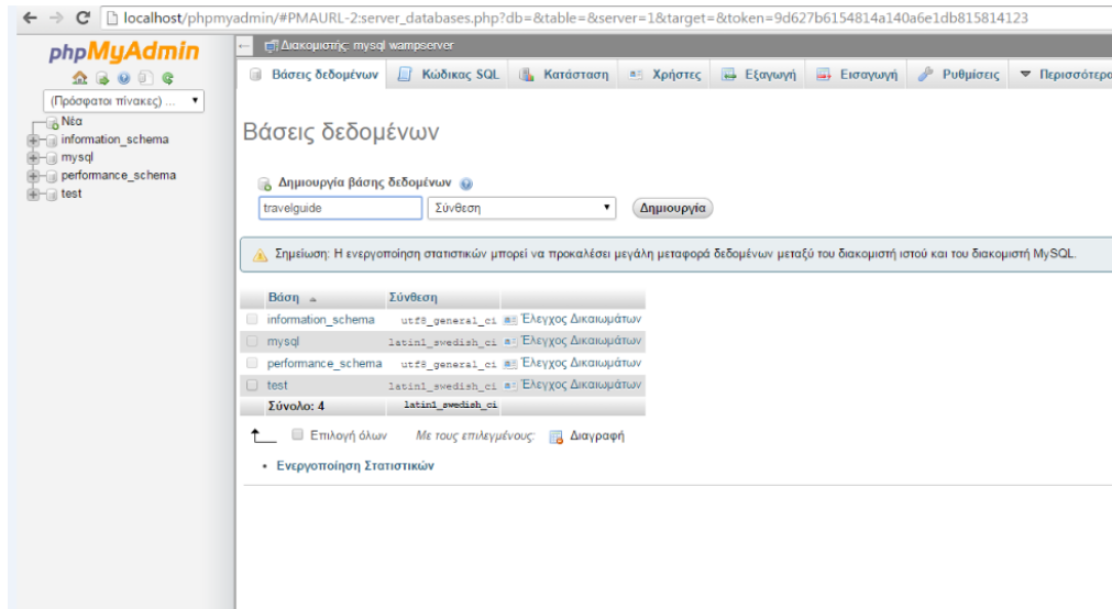
Εικόνα 17. Δημιουργία βάσης
