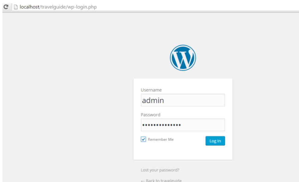
Εικόνα 24.Login
