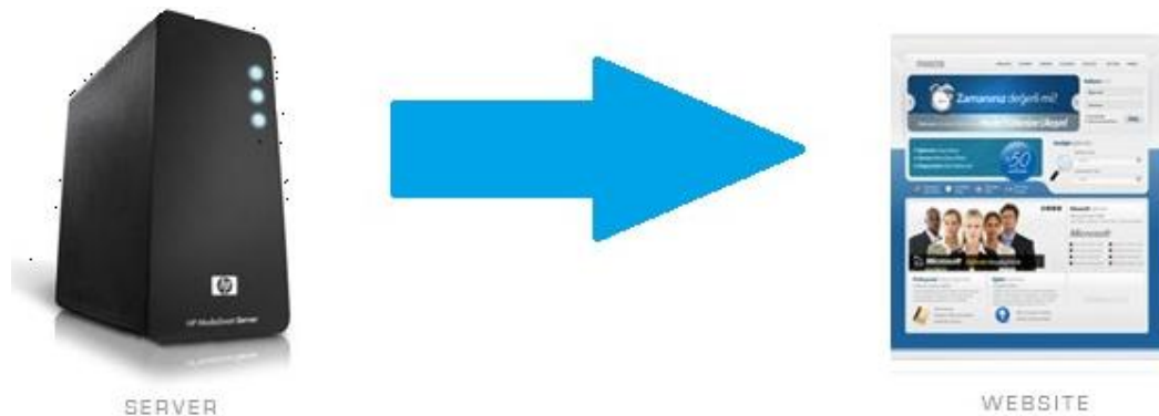
Εικόνα 1. Στατική Ιστοσελίδα
