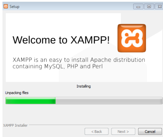
Εικόνα 15.Εγκατάσταση xampp-Βήμα 4
