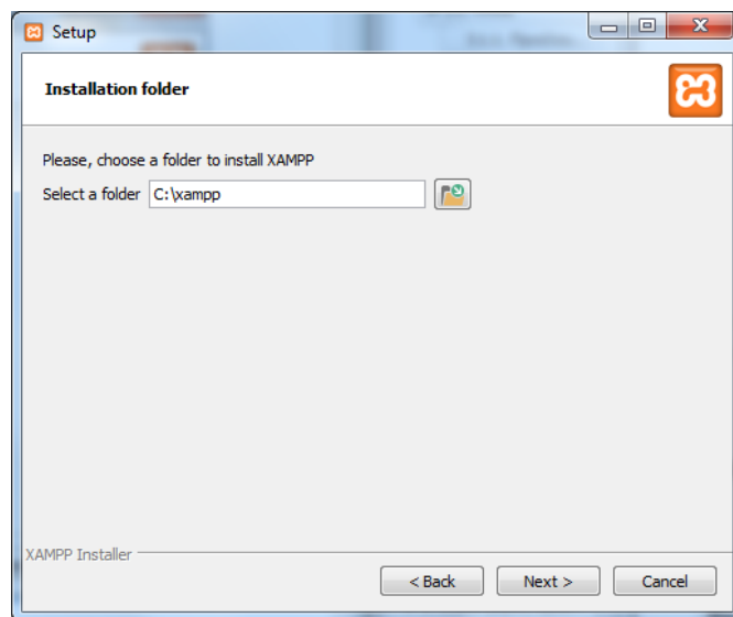
Εικόνα 14.Εγκατάσταση xampp-Βήμα 3
