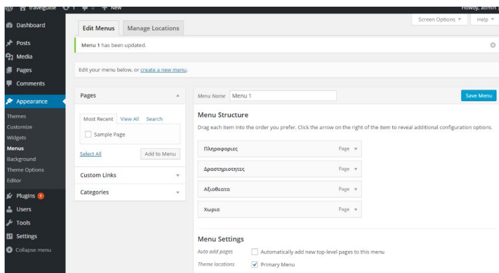
Εικόνα 26.Κεντρικό menu
