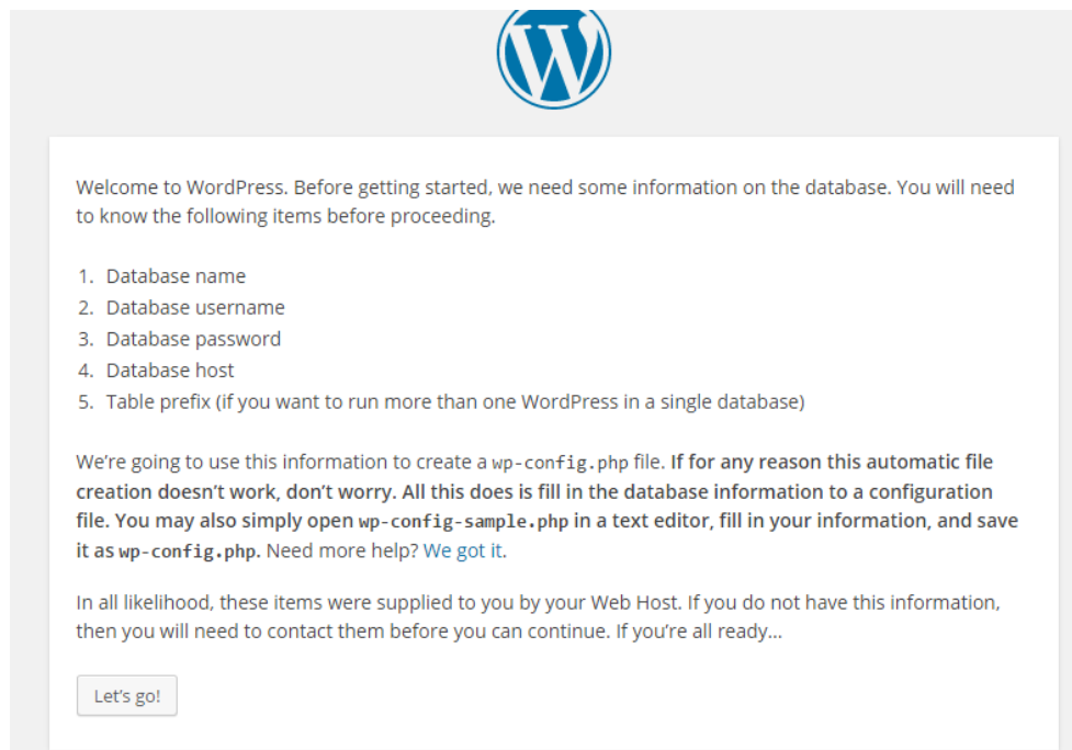
Εικόνα 19. Σελίδα εγκατάστασης
