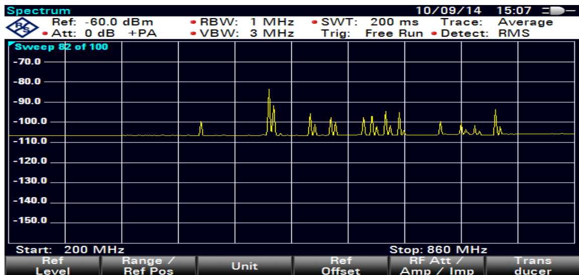
Οθόνη του αναλυτή φάσματος κατά την μέτρηση στην Z κατεύθυνση της κεραίας λήψης
